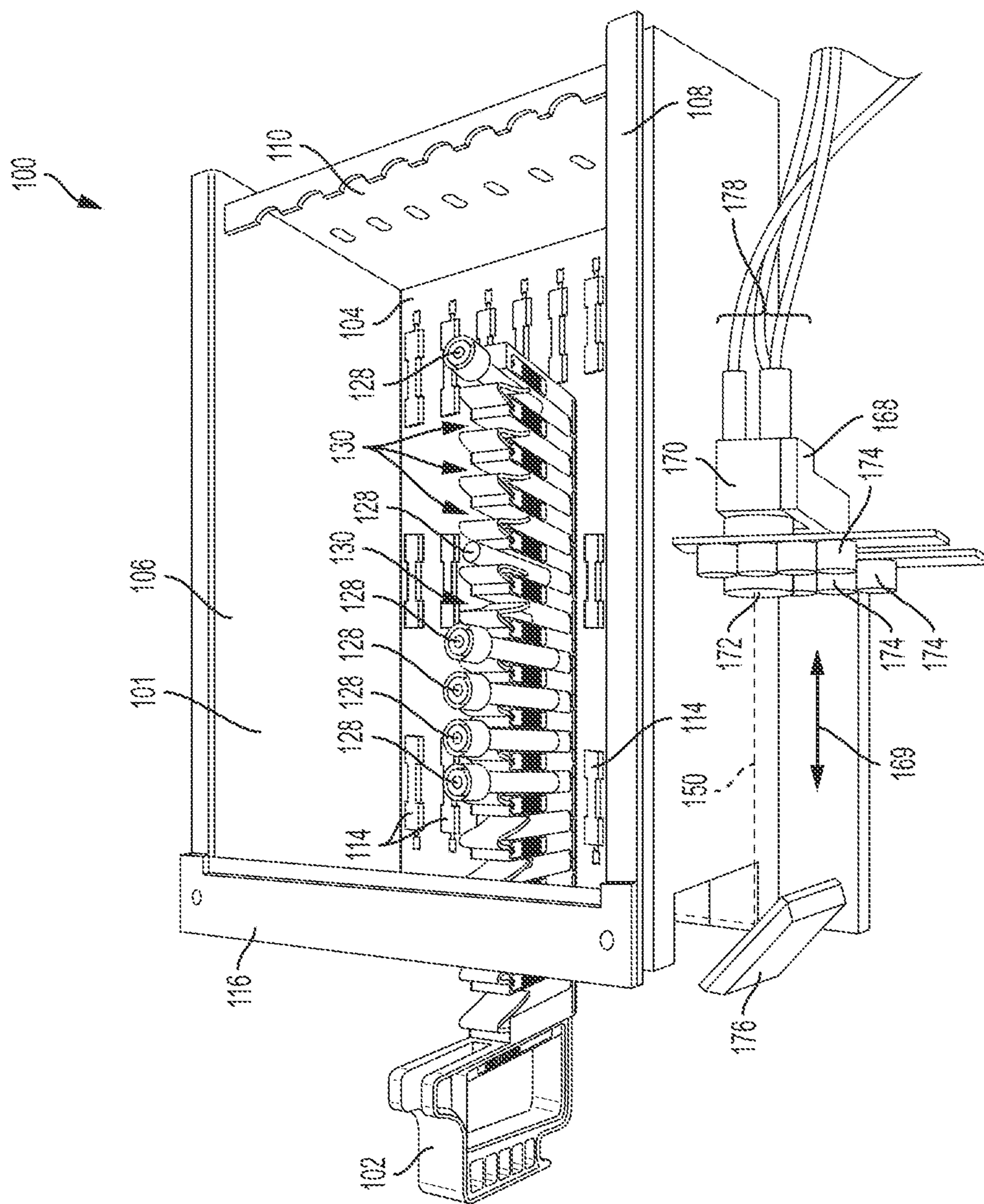
FIG. 17
