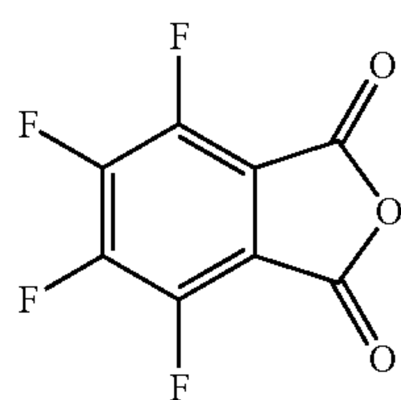
tetrafluorophthalic anhydride
