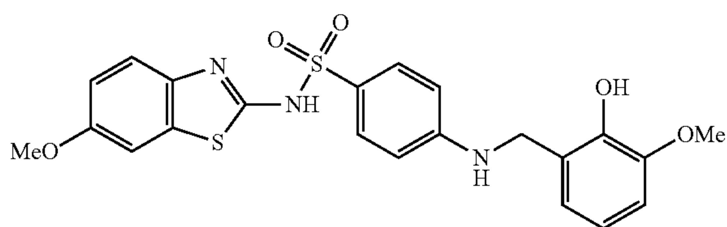
4-((2-hydroxy-3-methoxybenzyl)amino)-N-(6-methoxybenzo[d]thiazol-2-yl)benzenesulfonamide, TFA (62)
