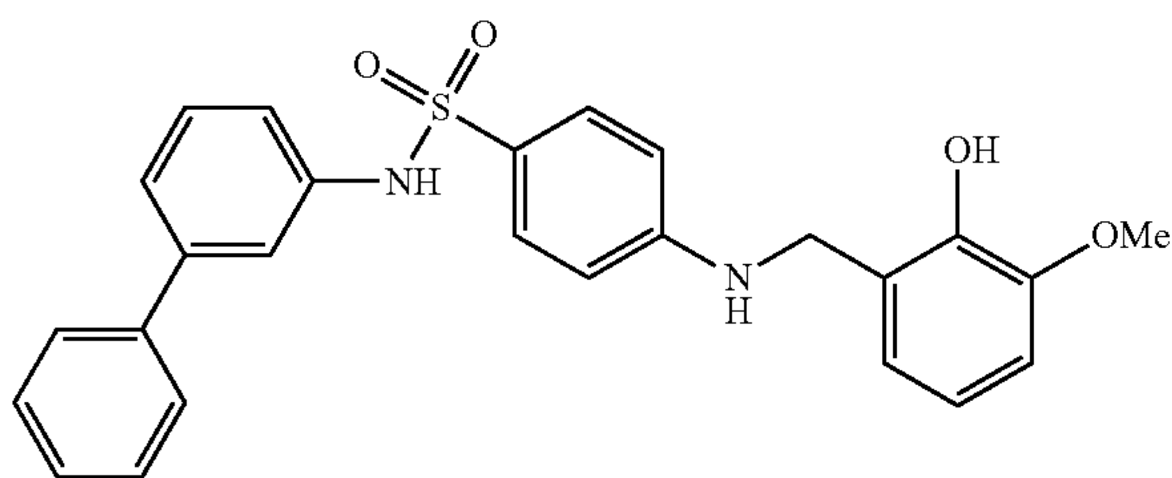
N-([1,1'-biphenyl]-3-yl)-4-((2-hydroxy-3-methoxybenzyl)amino)benzenesulfonamide (52)
