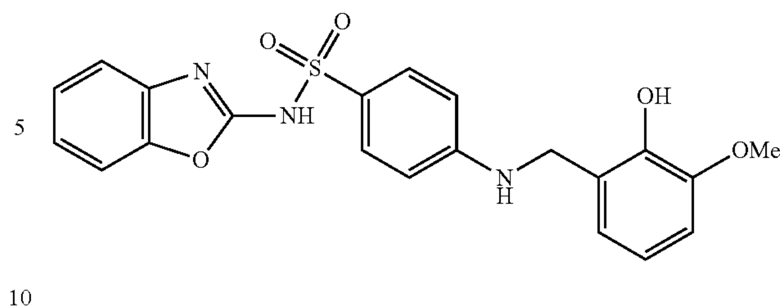
N-(benzo[d]oxazol-2-yl)-4-((2-hydroxy-3-methoxybenzyl)amino)benzenesulfonamide (36)
