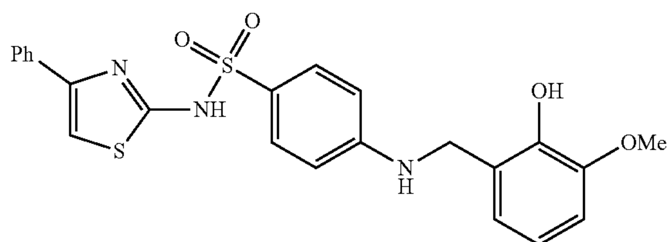
4-((2-hydroxy-3-methoxybenzyl)amino)-N-(4-phenylthiazol-2-yl)benzenesulfonamide, TFA (63)
