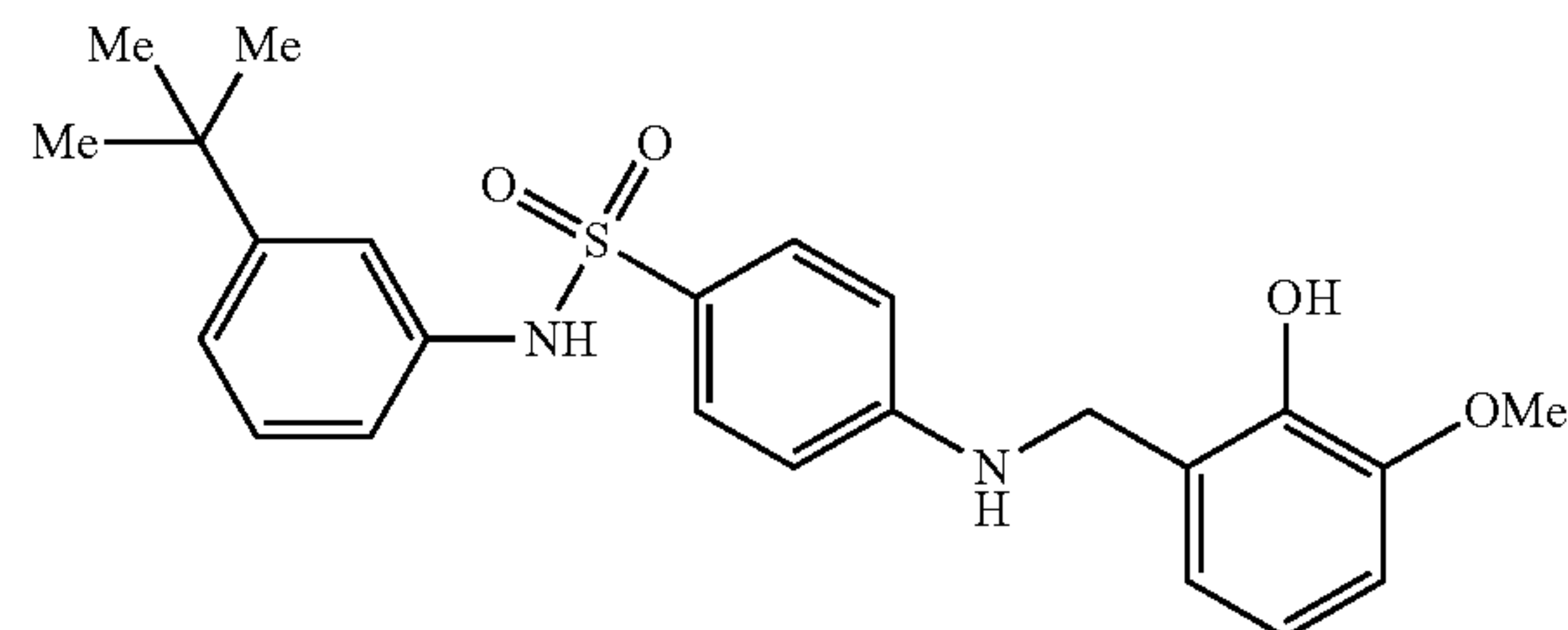
N-(3-(tert-butyl)phenyl)-4-((2-hydroxy-3-methoxybenzyl)amino)benzenesulfonamide, TFA (61)
