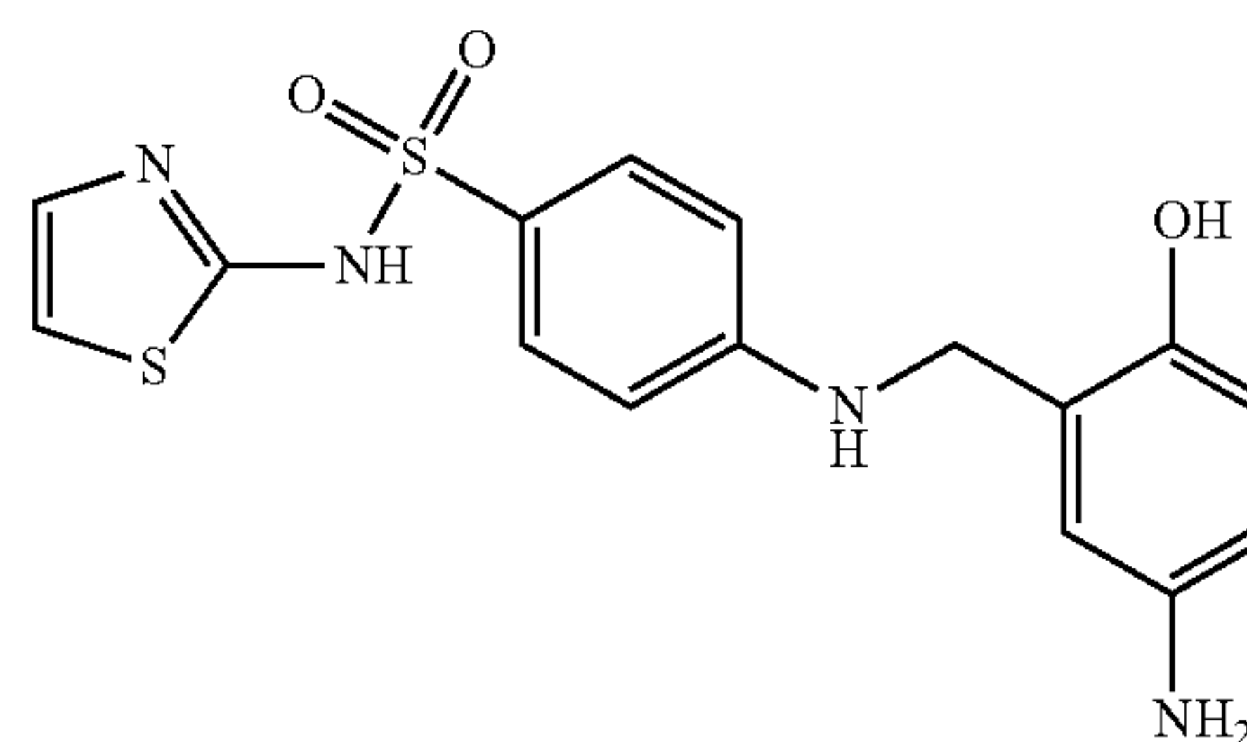
4-(5-amino-2-hydroxybenzylamino)-N-(thiazol-2-yl)benzenesulfonamide (31)
