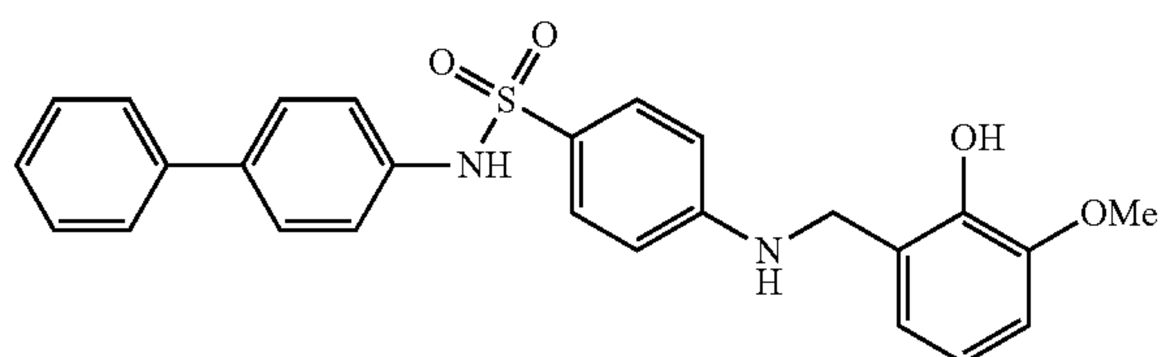
N-([1,1'-biphenyl]-4-yl)-4-((2-hydroxy-3-methoxybenzyl)amino)benzenesulfonamide (51)
