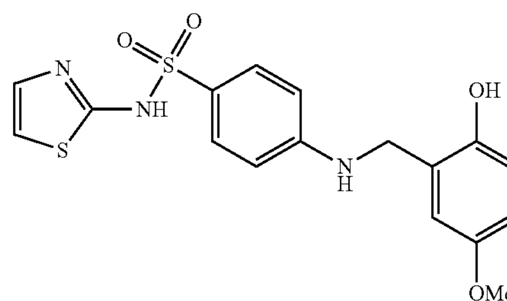
4-(2-hydroxy-5-methoxybenzylamino)-N-(thiazol-2-yl)benzenesulfonamide (30)
