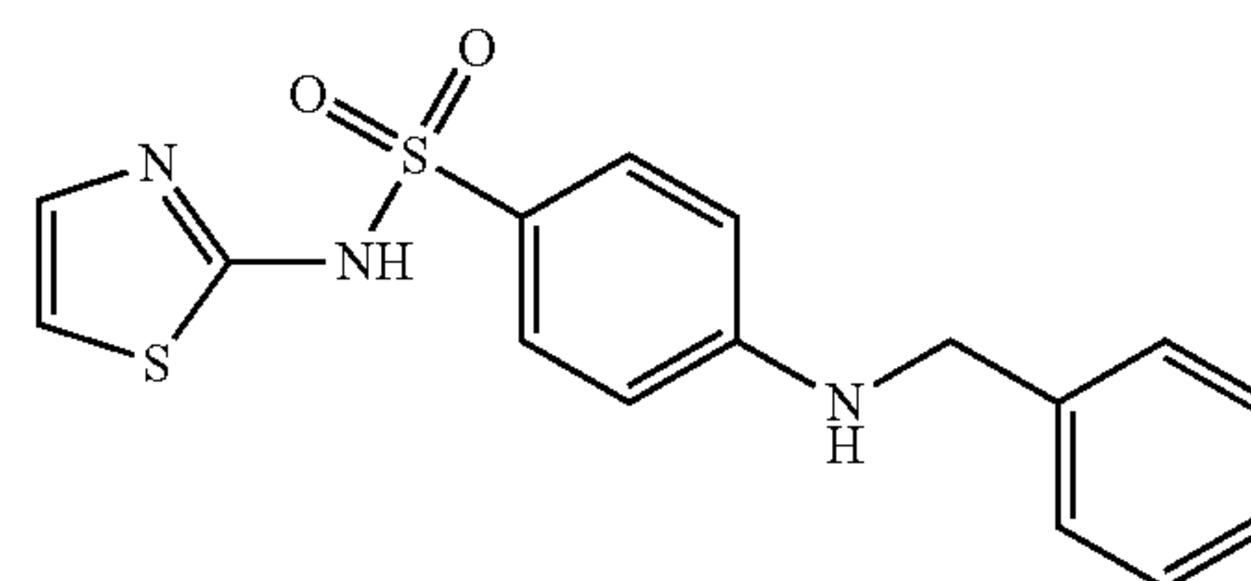
4-(benzylamino)-N-(thiazol-2-yl)benzenesulfonamide TFA (8)
