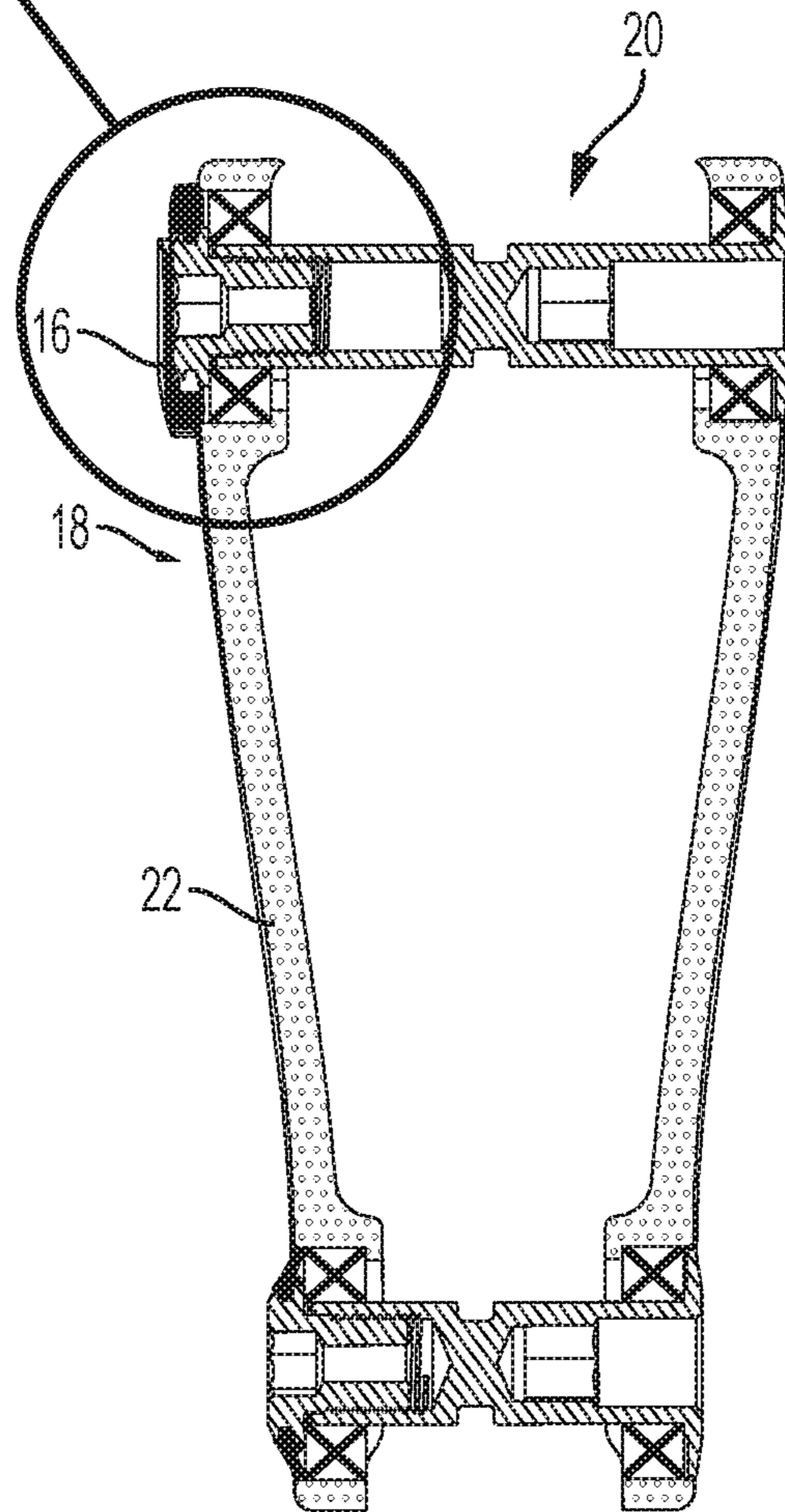
SECTION A-A
