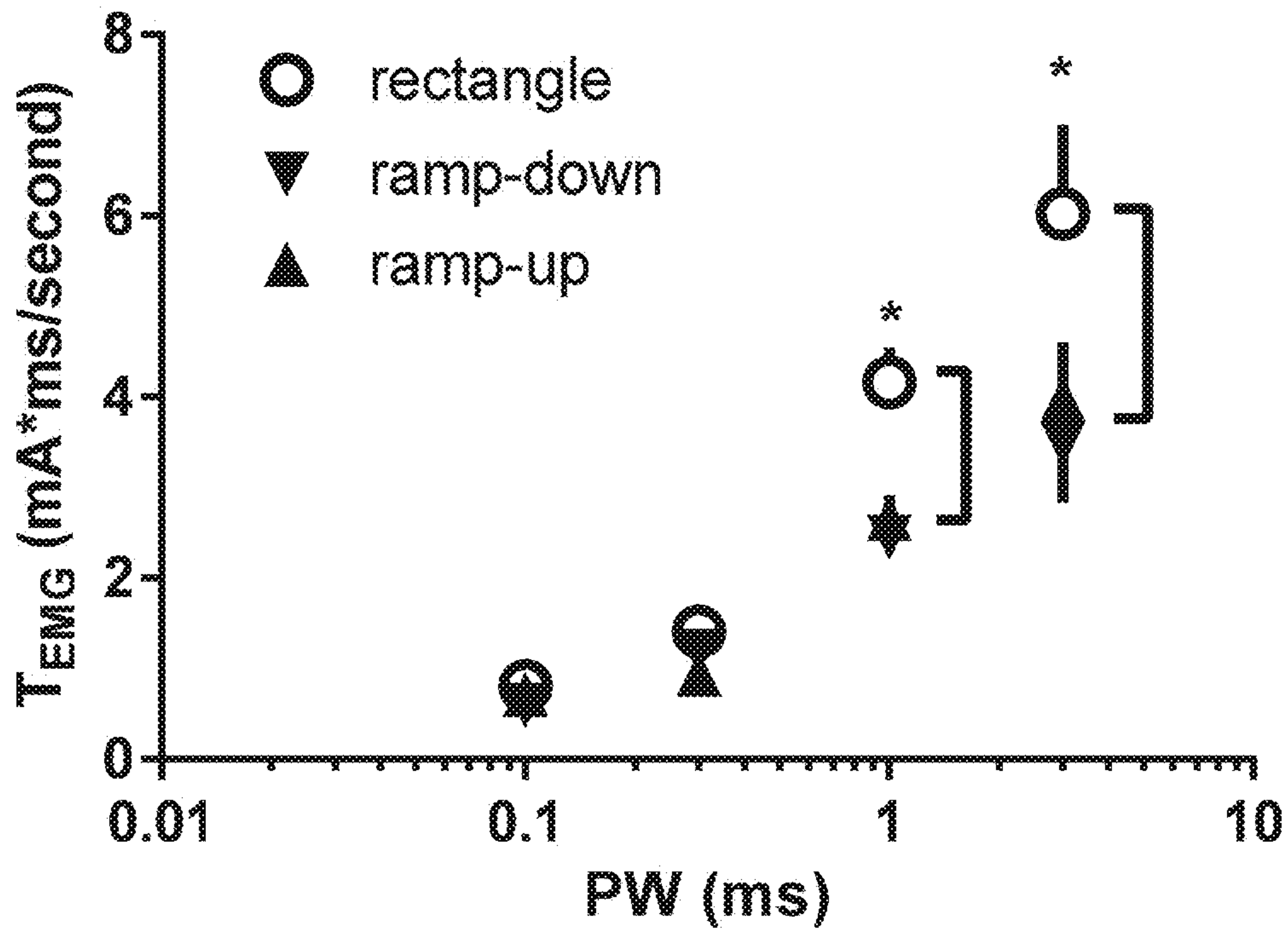
FIG. 11C
