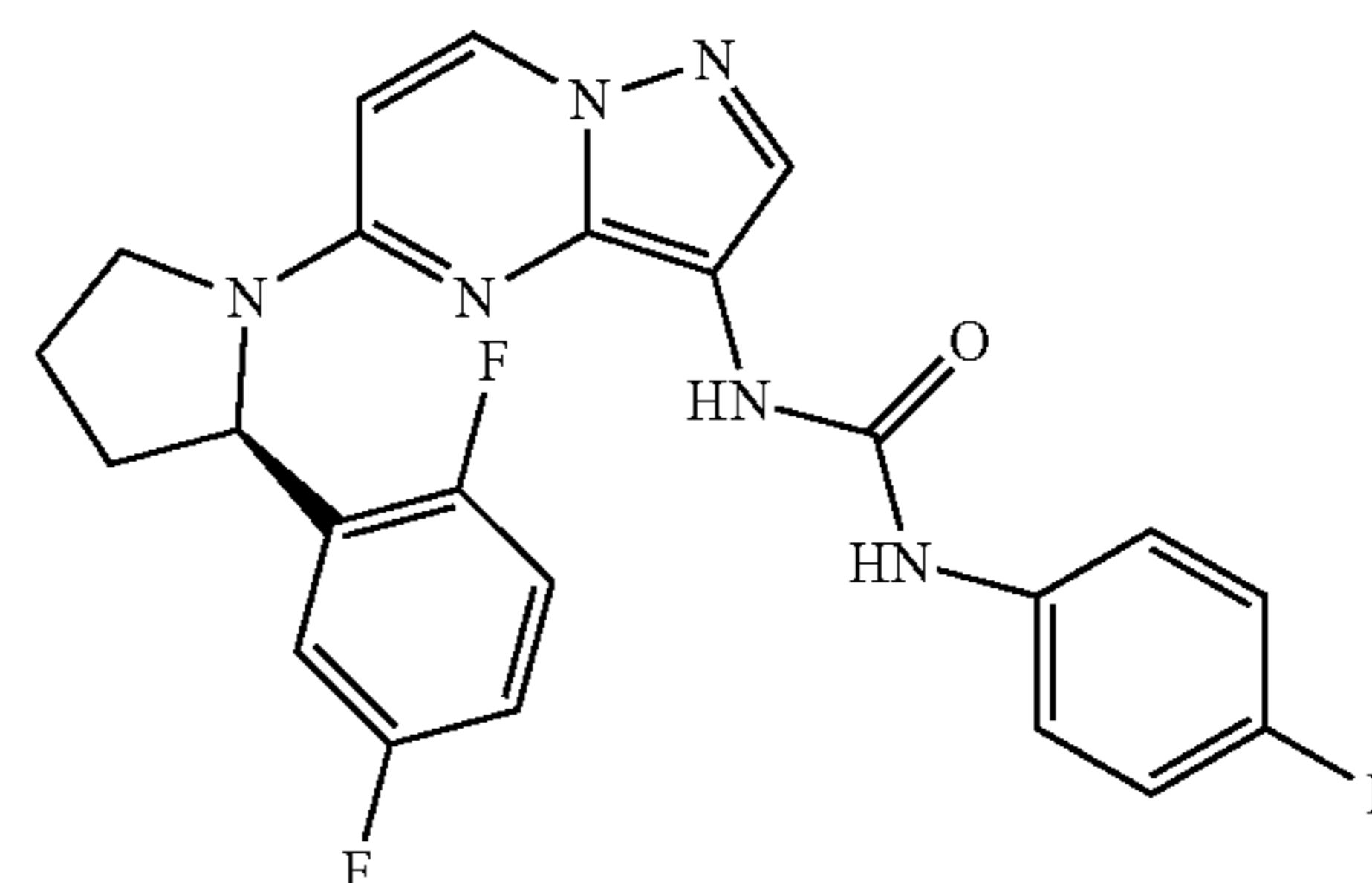
(R)-1-(5-(2-(2,5-difluorophenyl)pyrrolidin-1-yl)pyrazolo[1,5-a]pyrimidin-3-yl)-3-(4-fluorophenyl)urea
