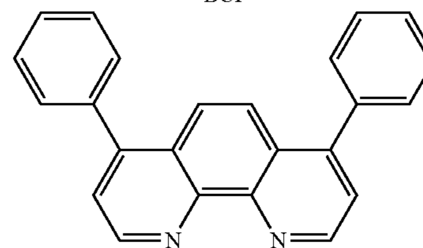
BCP
