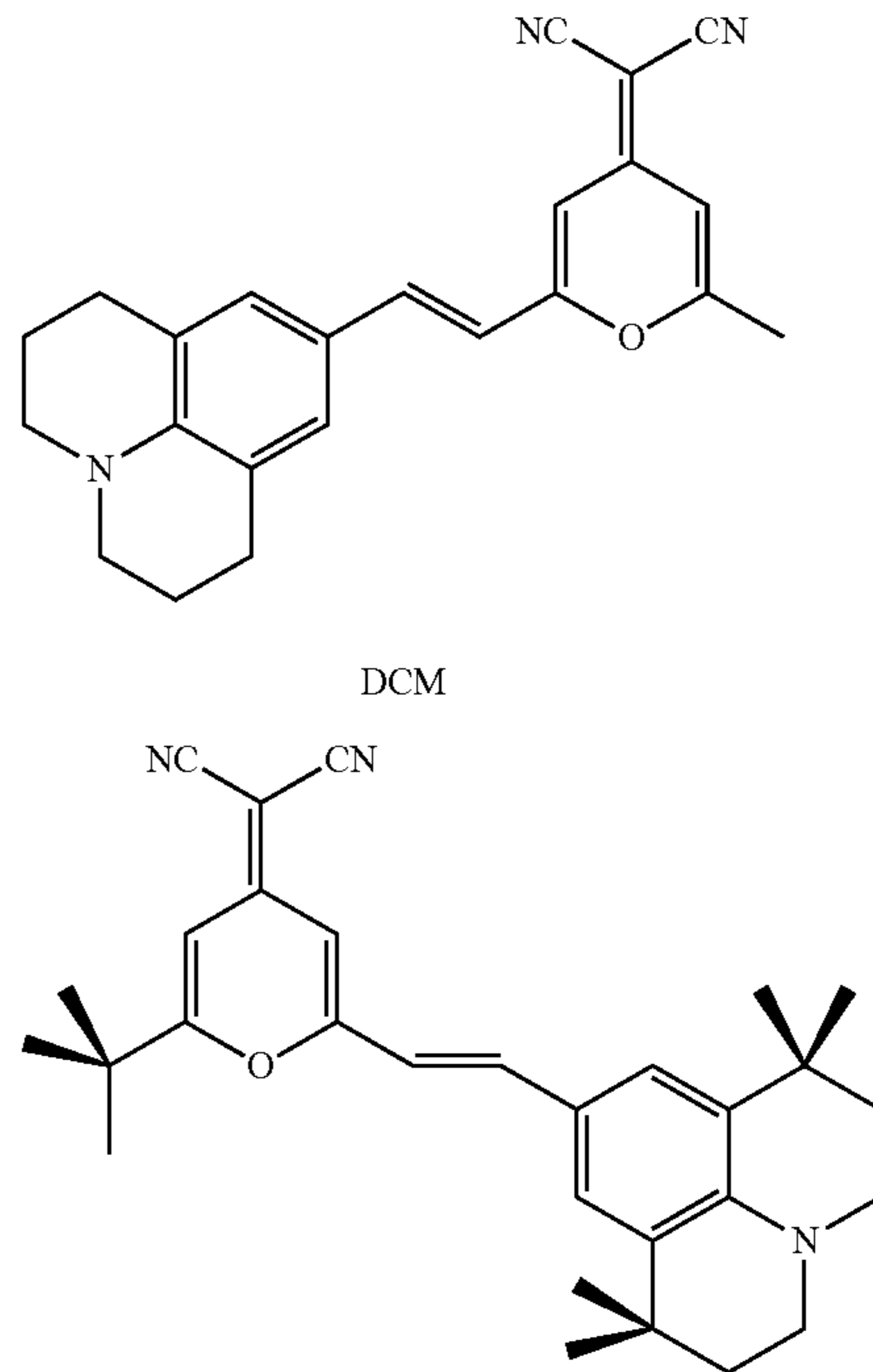
DCJTb
