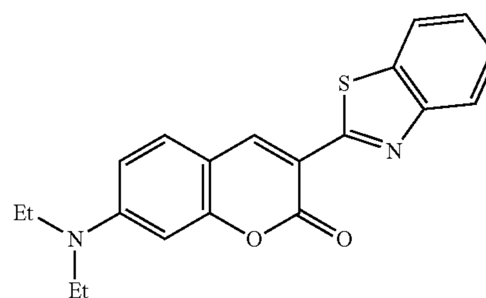
Coumarin 6
