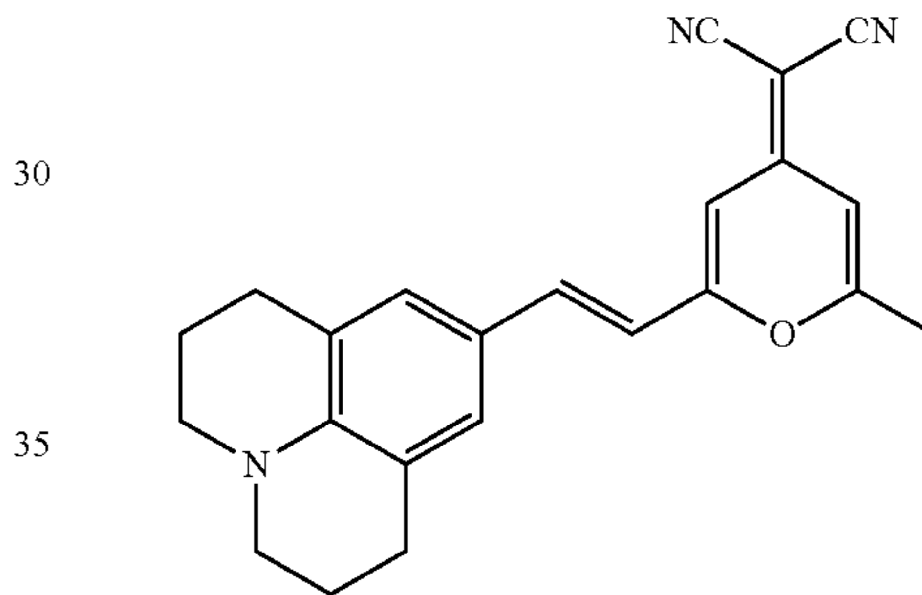
DCM
