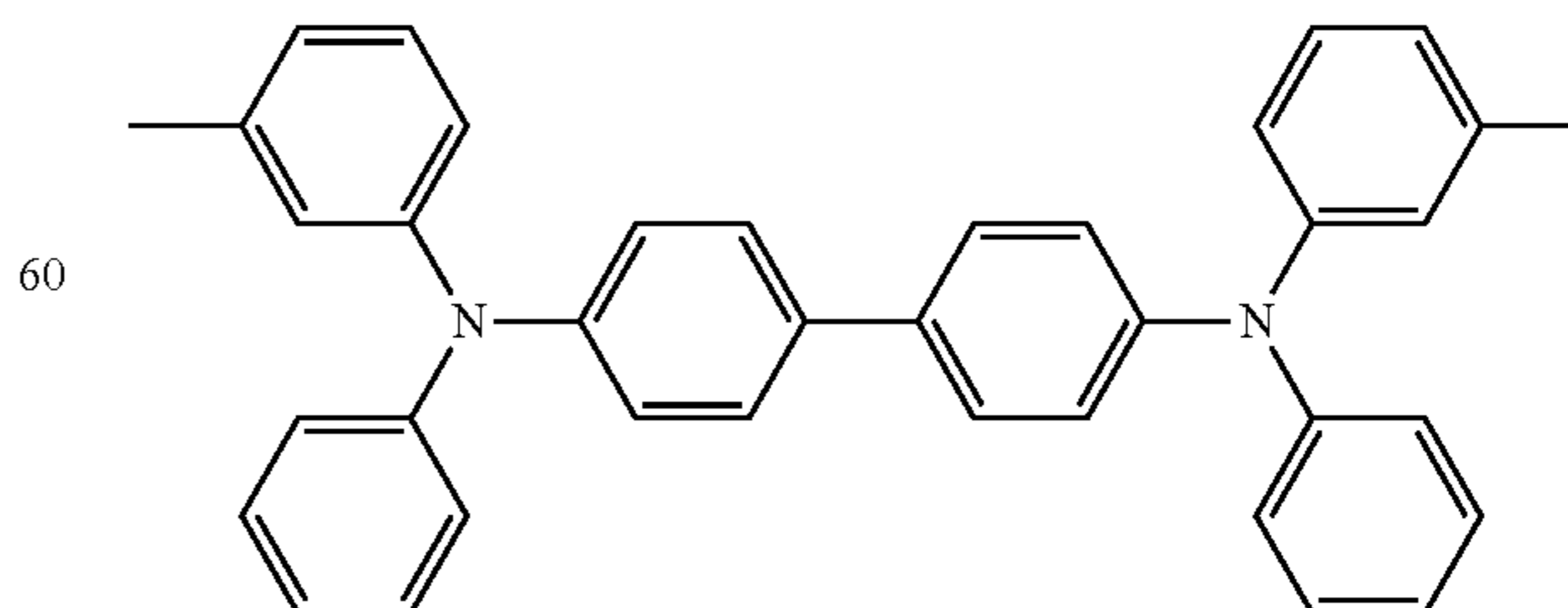
TPD
