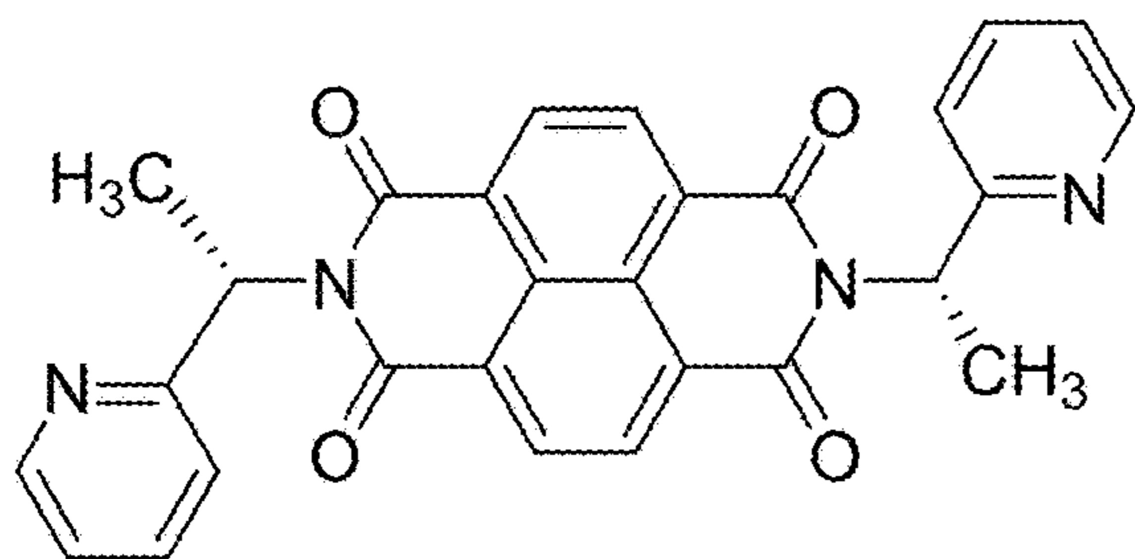
(S)-2-PyENDI
