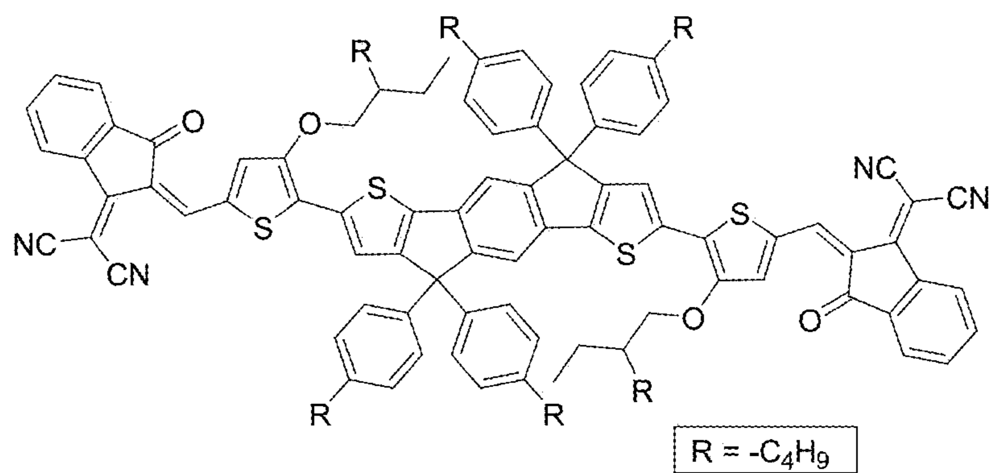
IEICO
