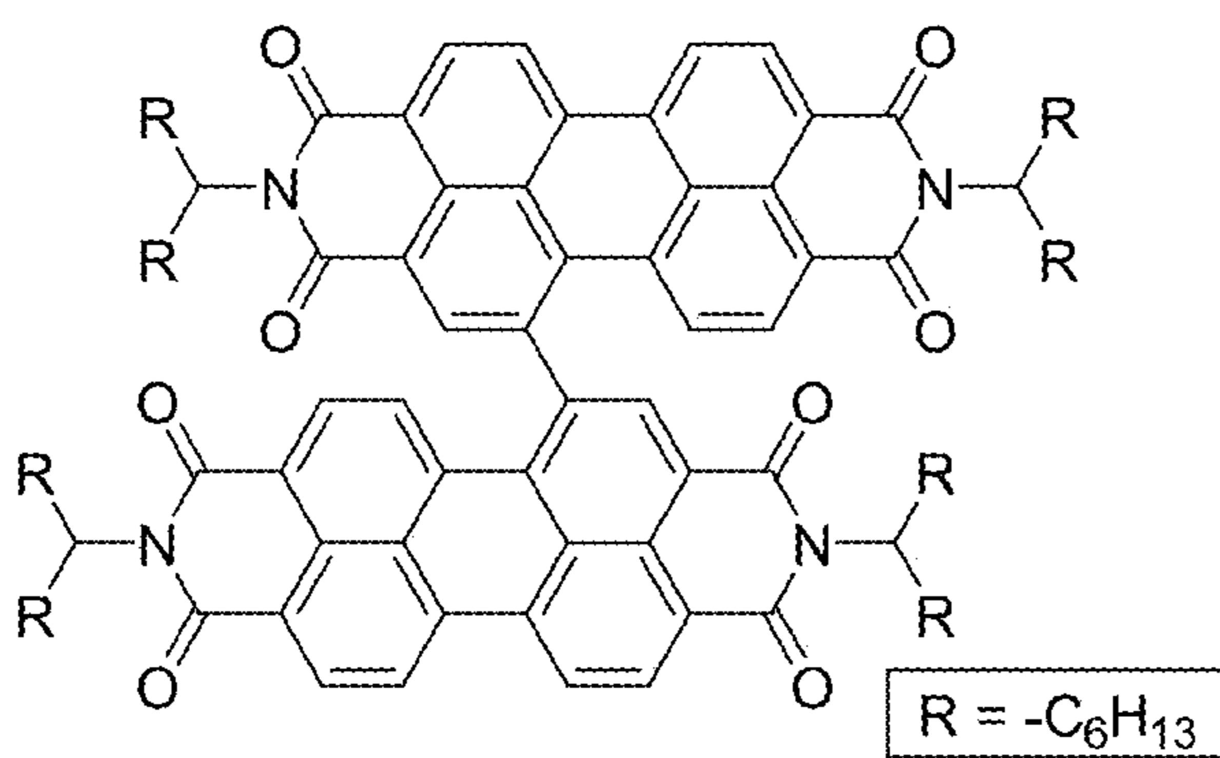
Di-PDI
