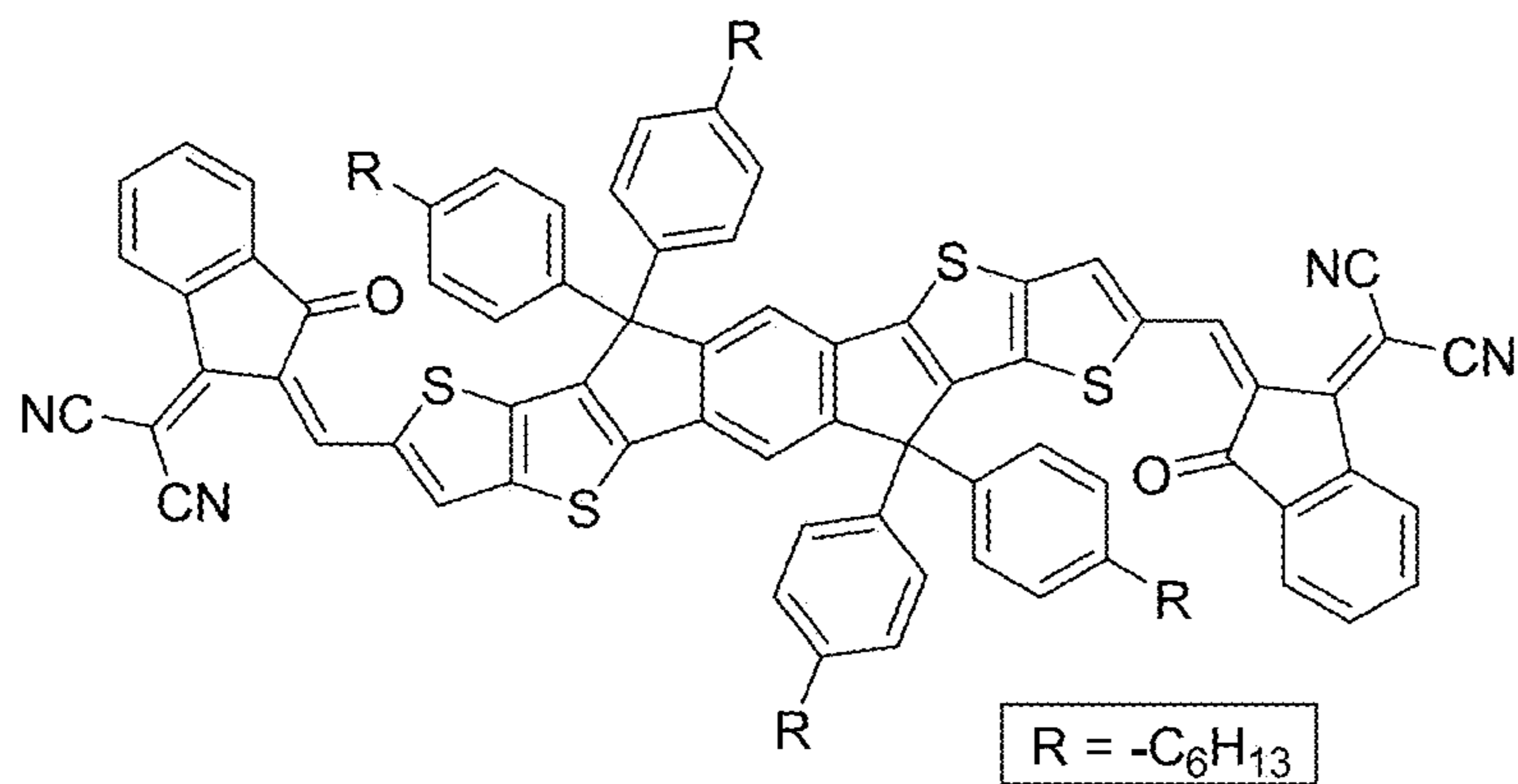
ITIC
