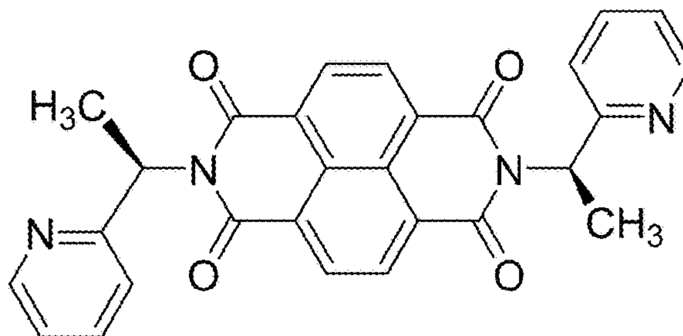
(R)-2-PyENDI
