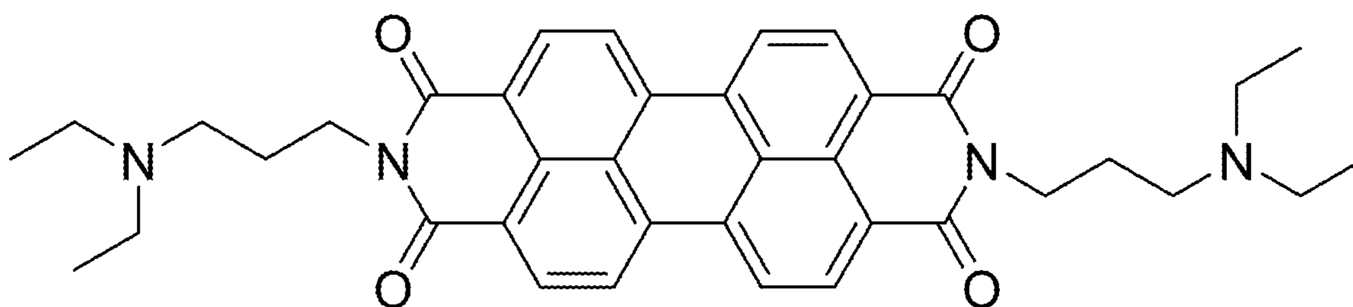
DEAPPDI
