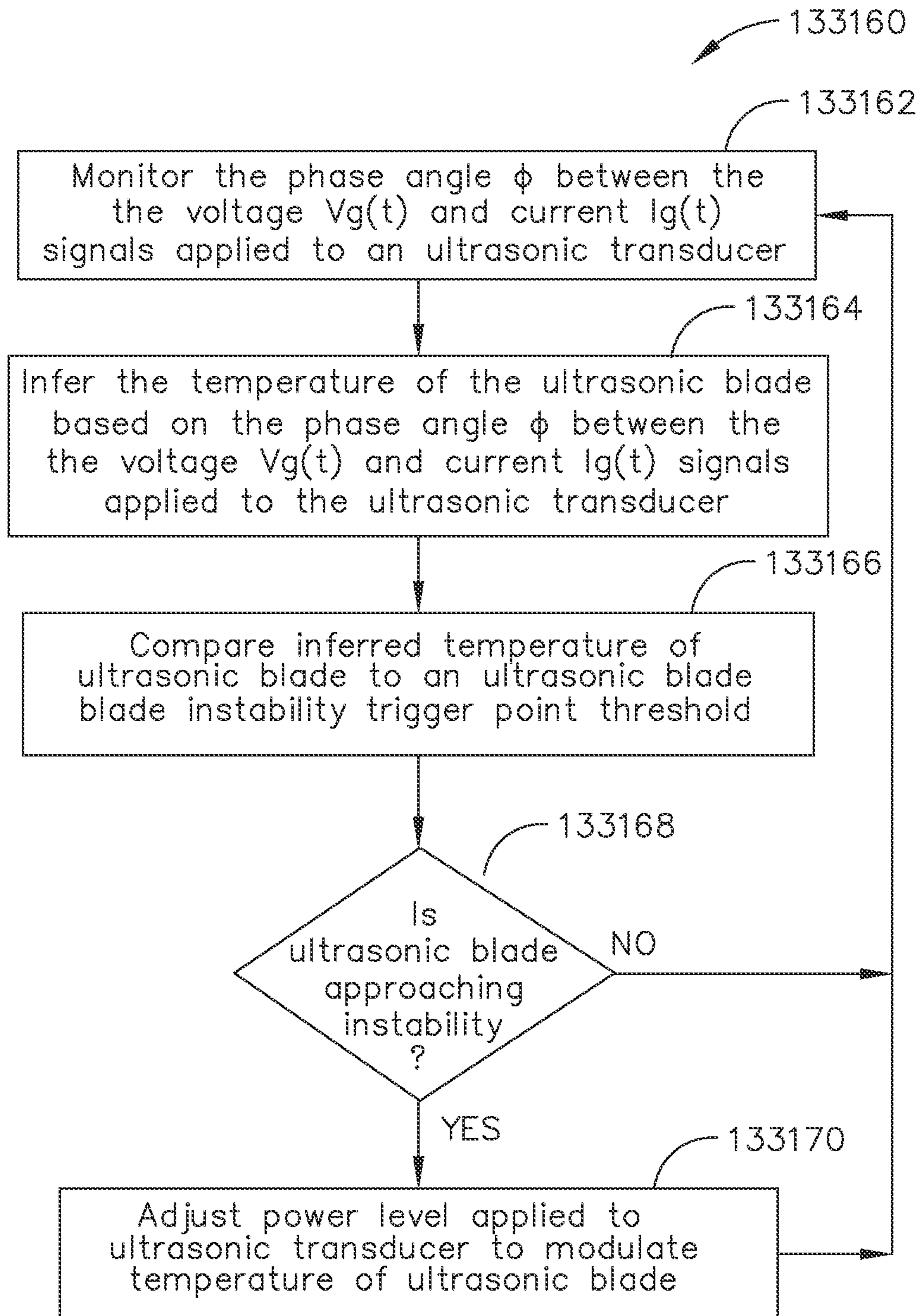
FIG. 32
