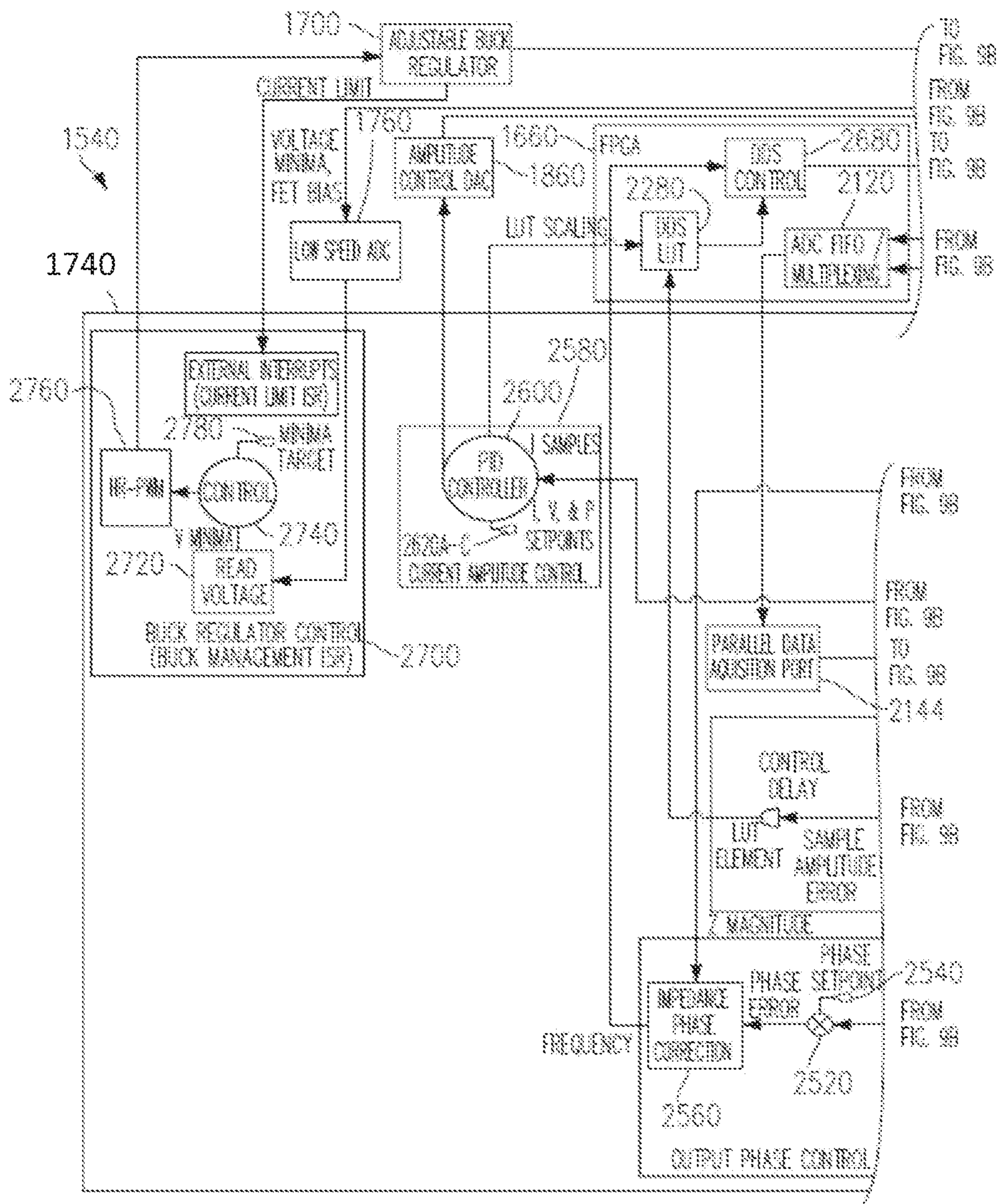
FIG. 9A
