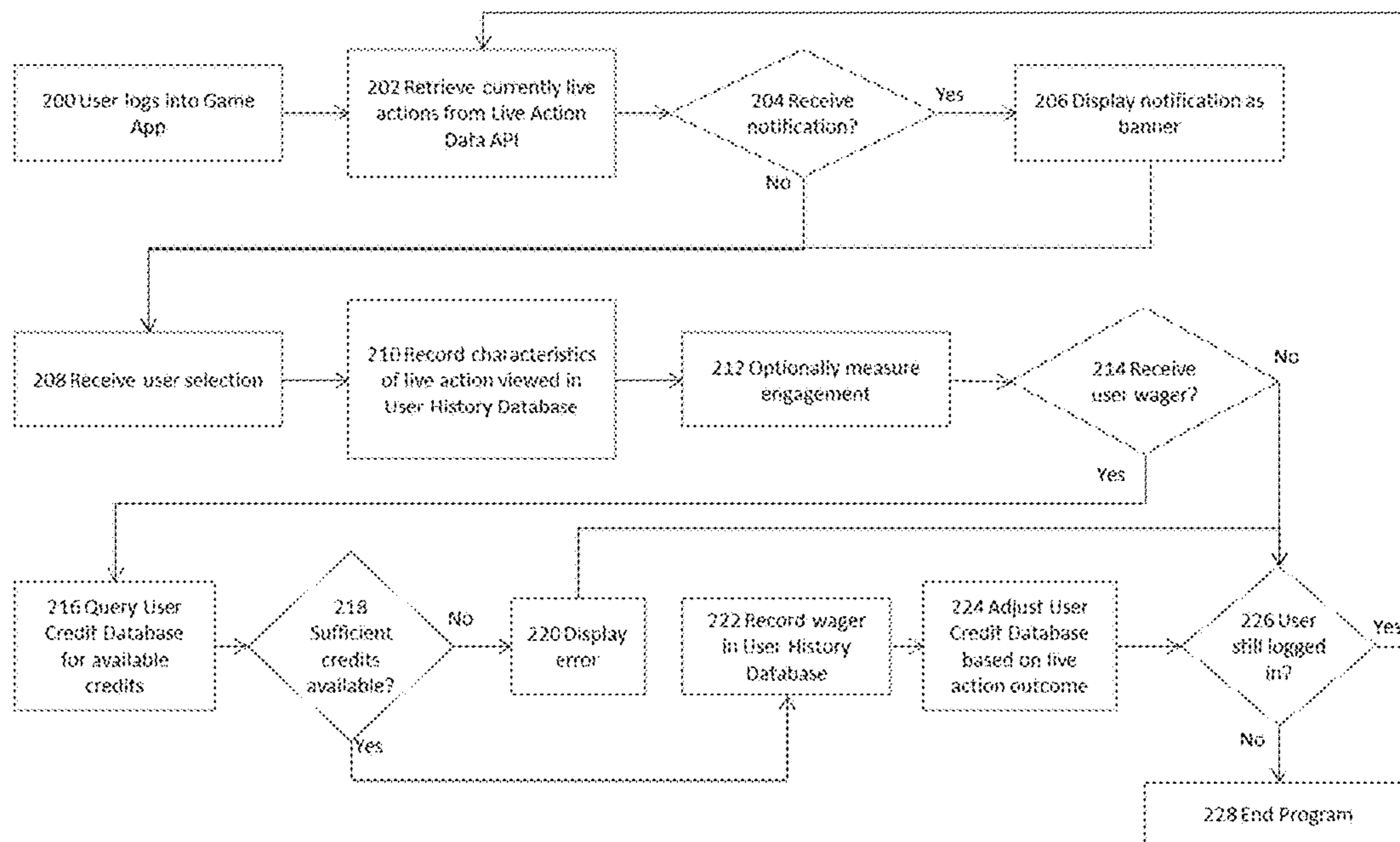
Fig. 2 Betting Module
