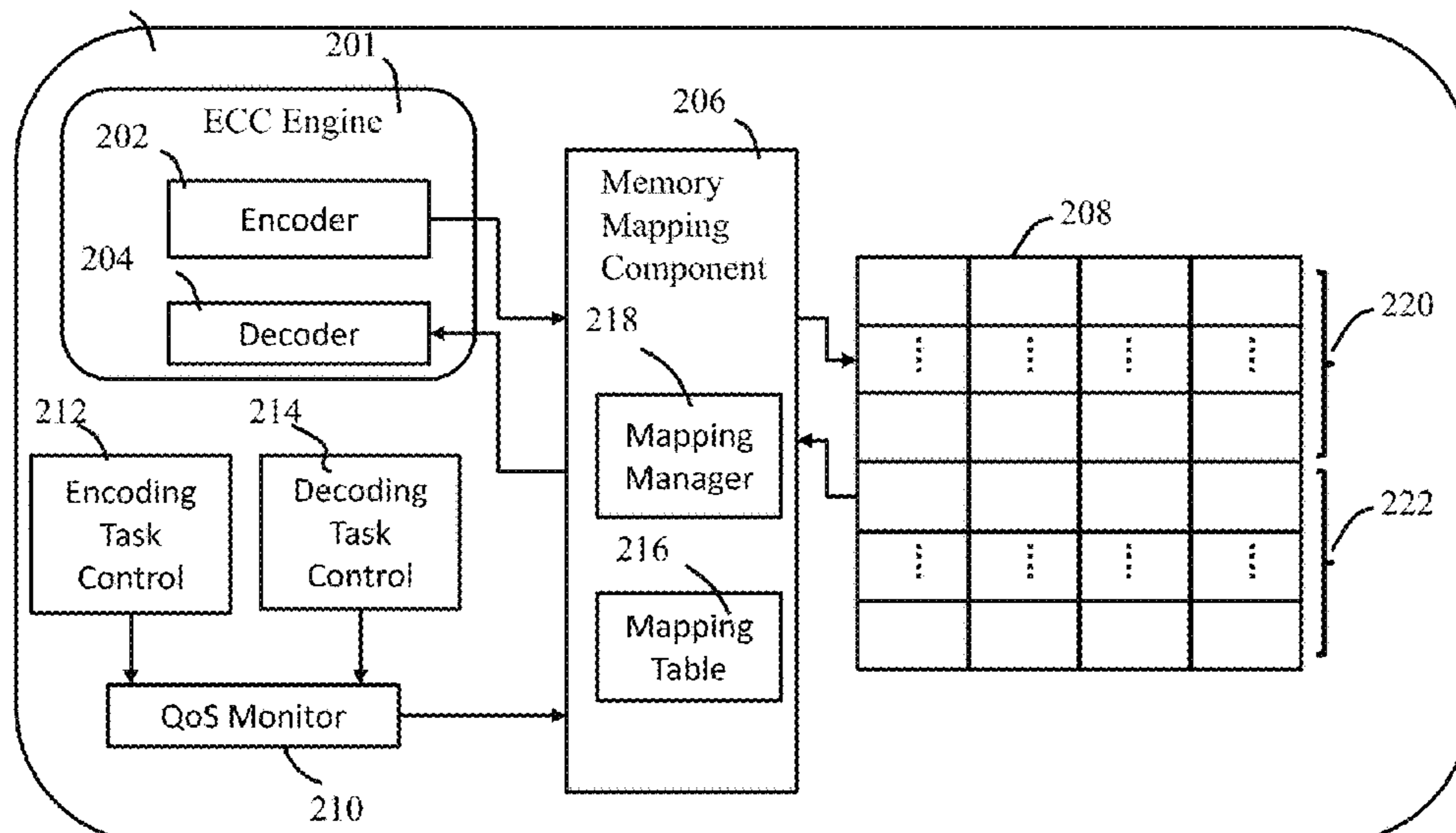
ECC Processor 200
