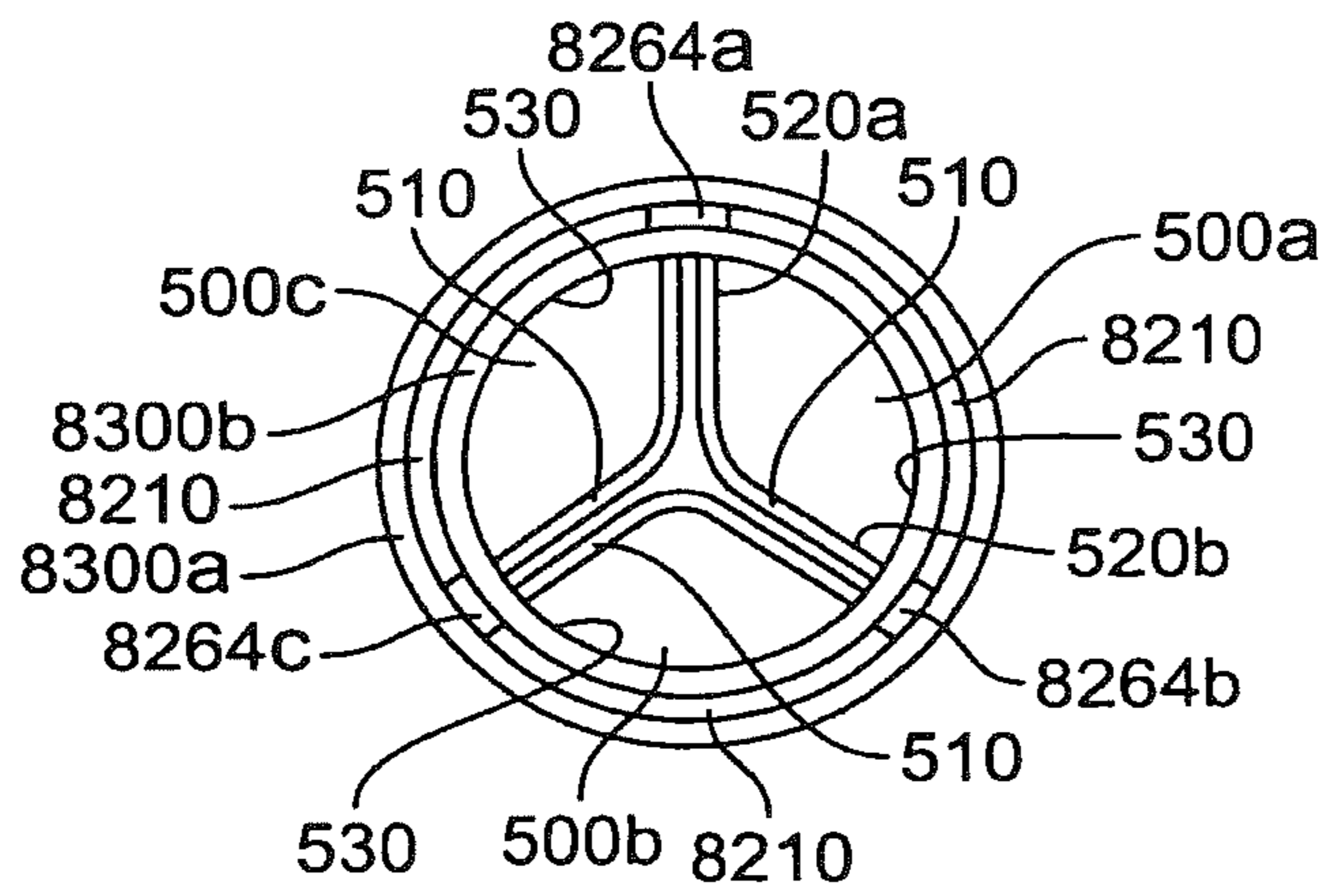
FIG. 30
