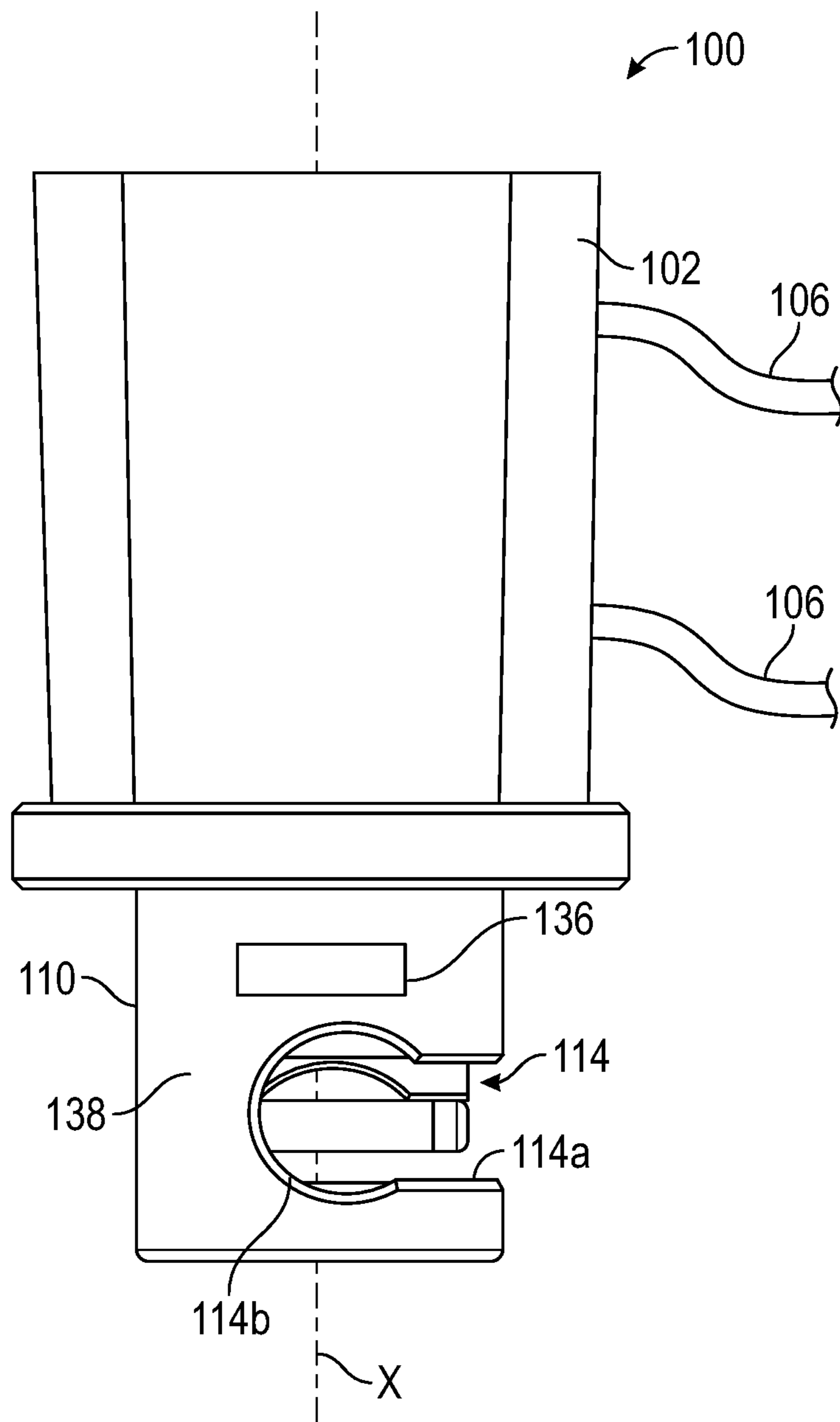
FIG. 2
