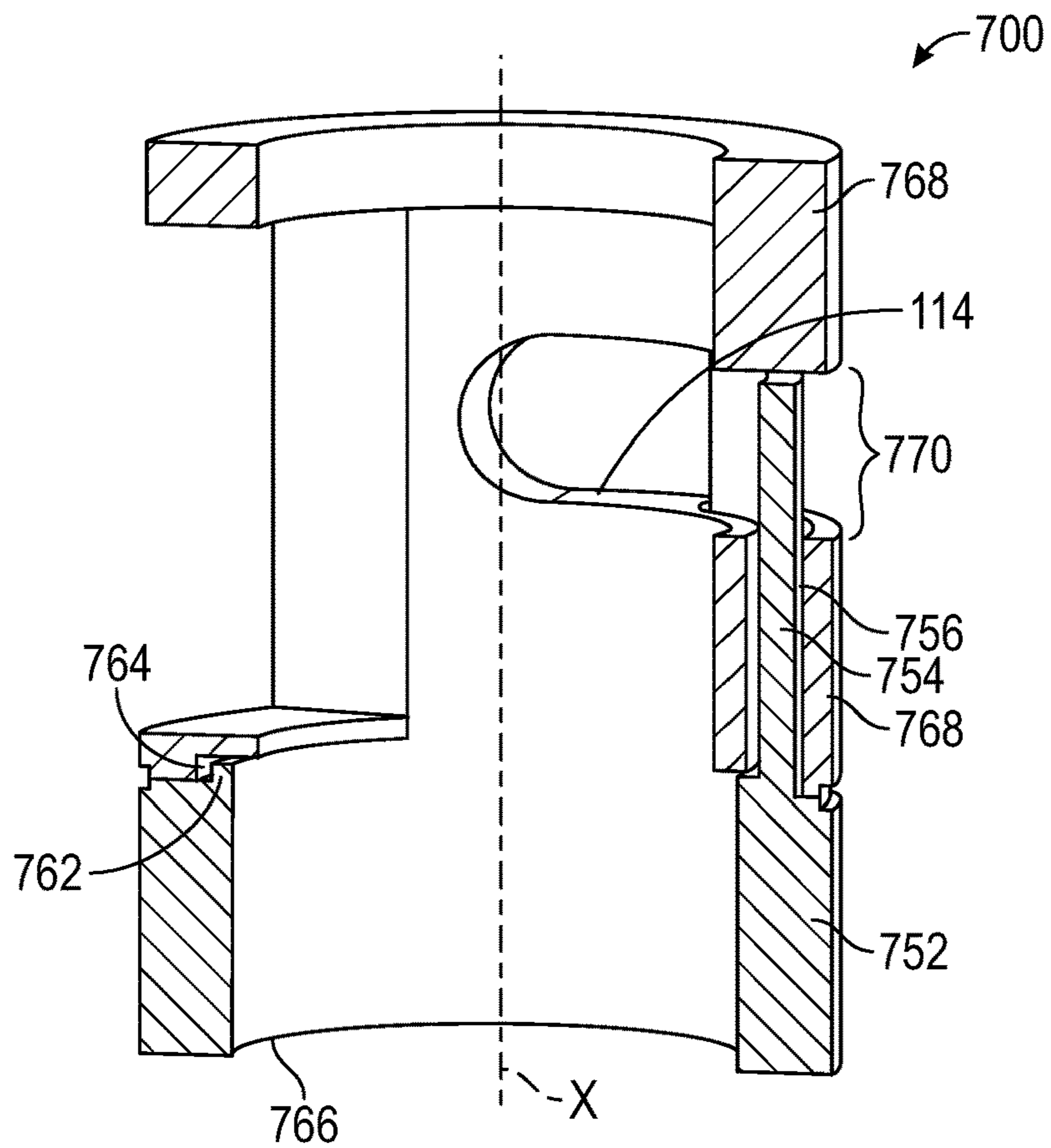
FIG. 23
