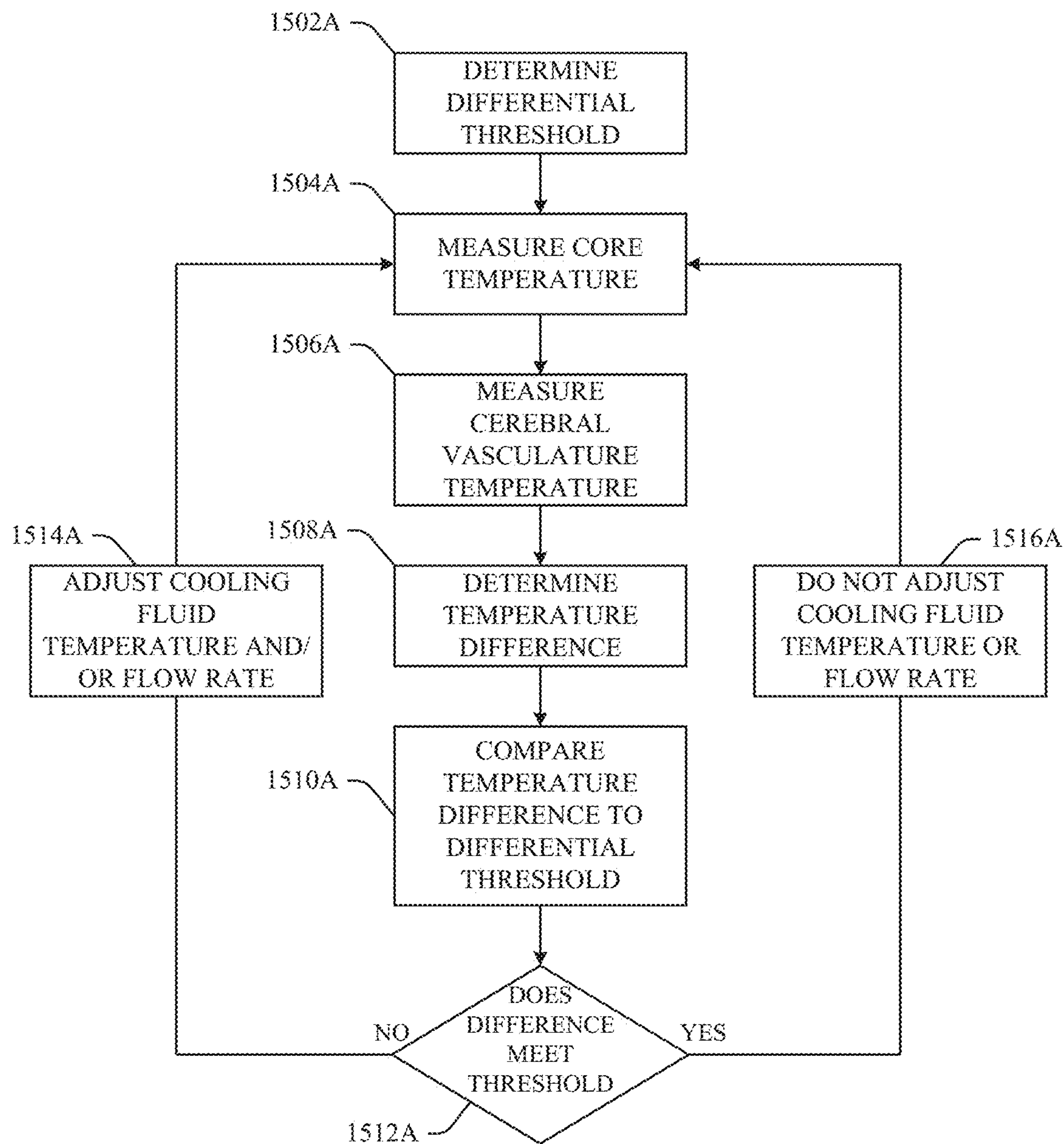
FIG. 15A
