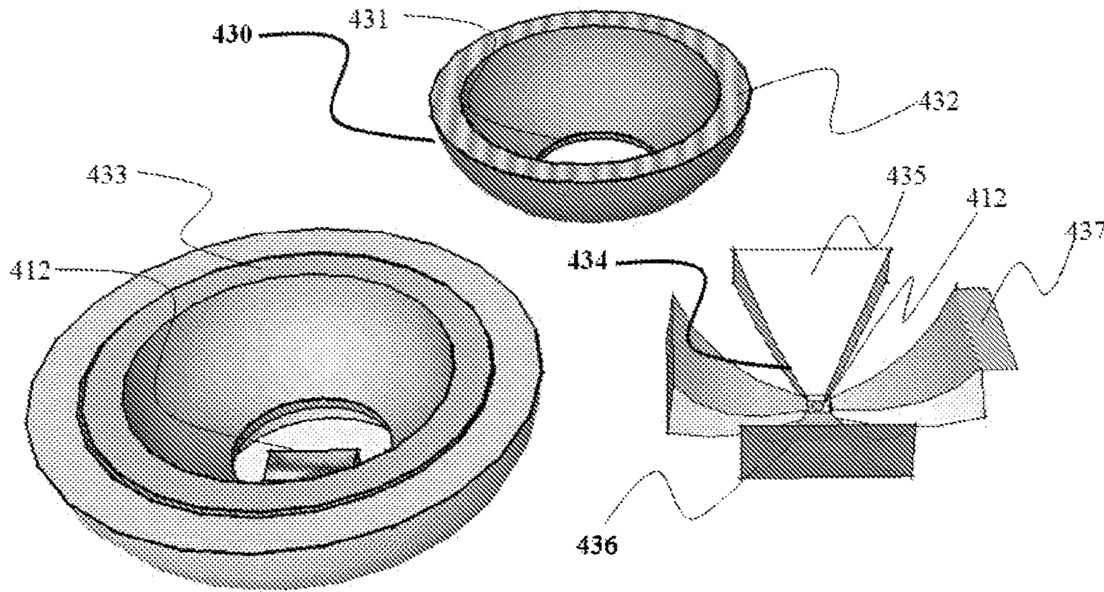
FIG. 19
