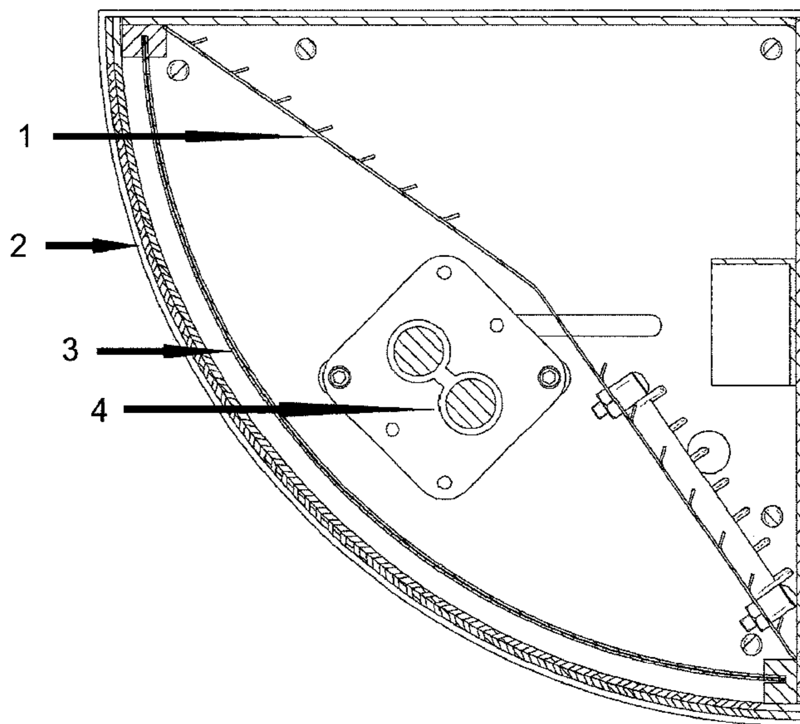
SECTION A-A
