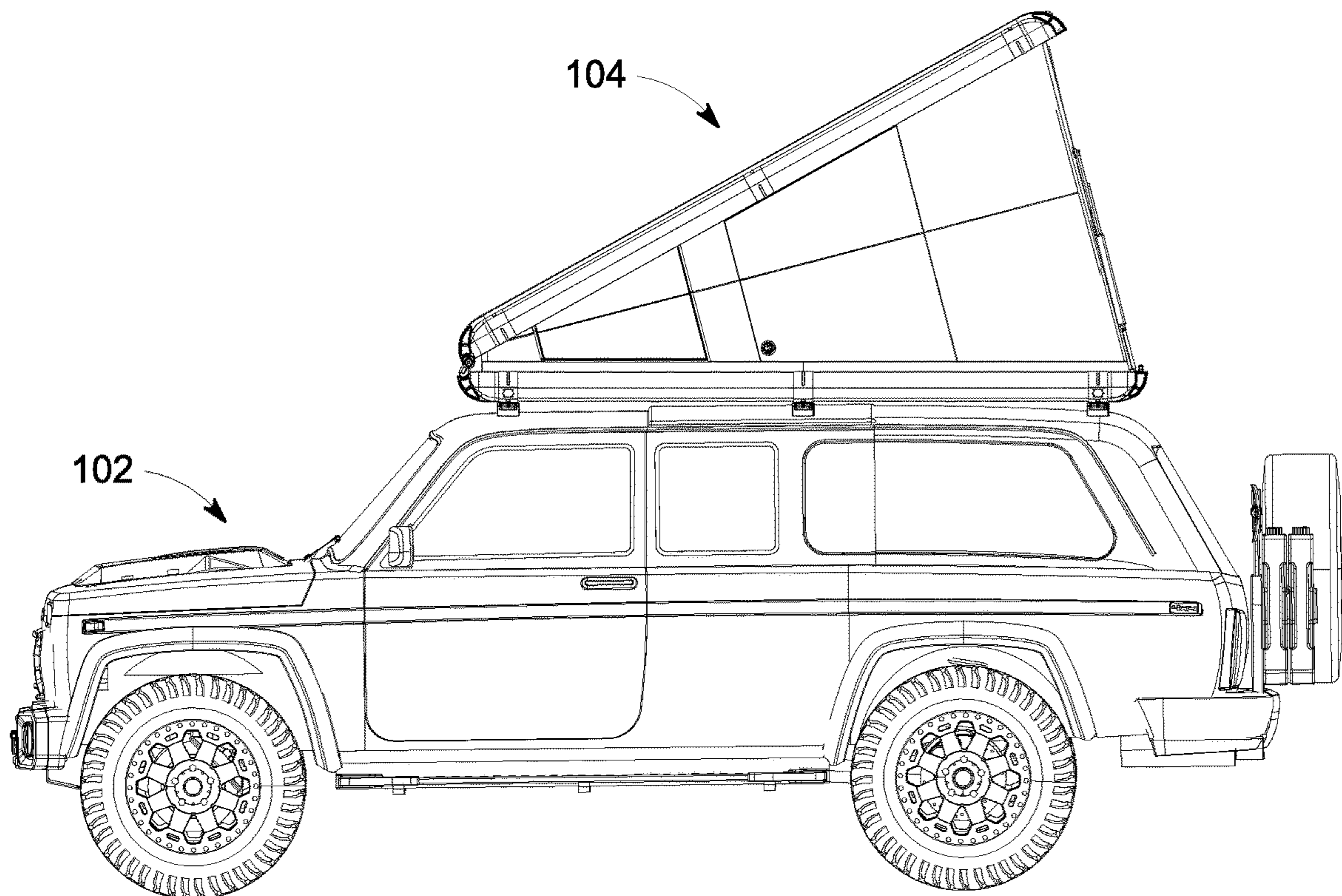
FIG. 43
