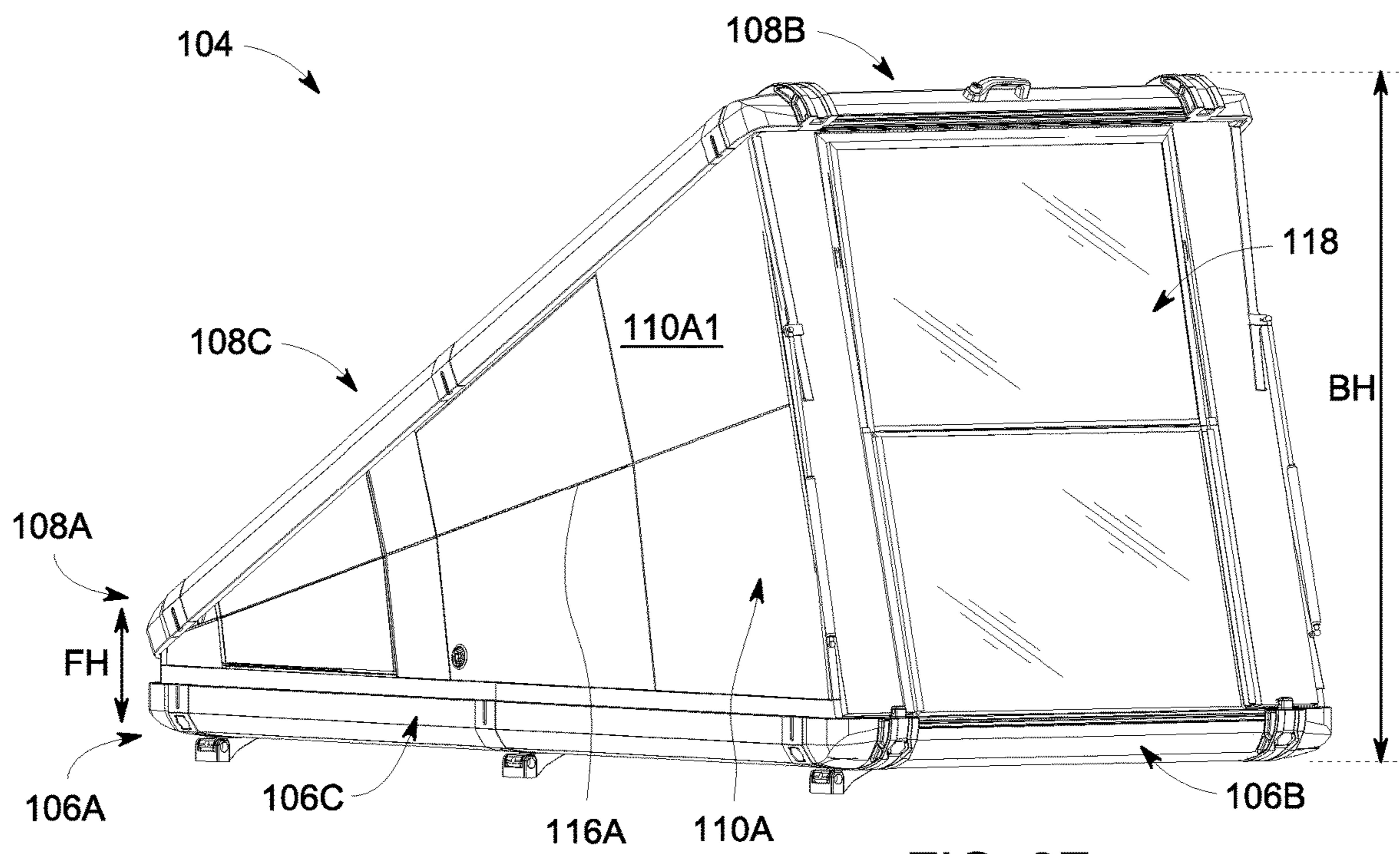
FIG. 2F
