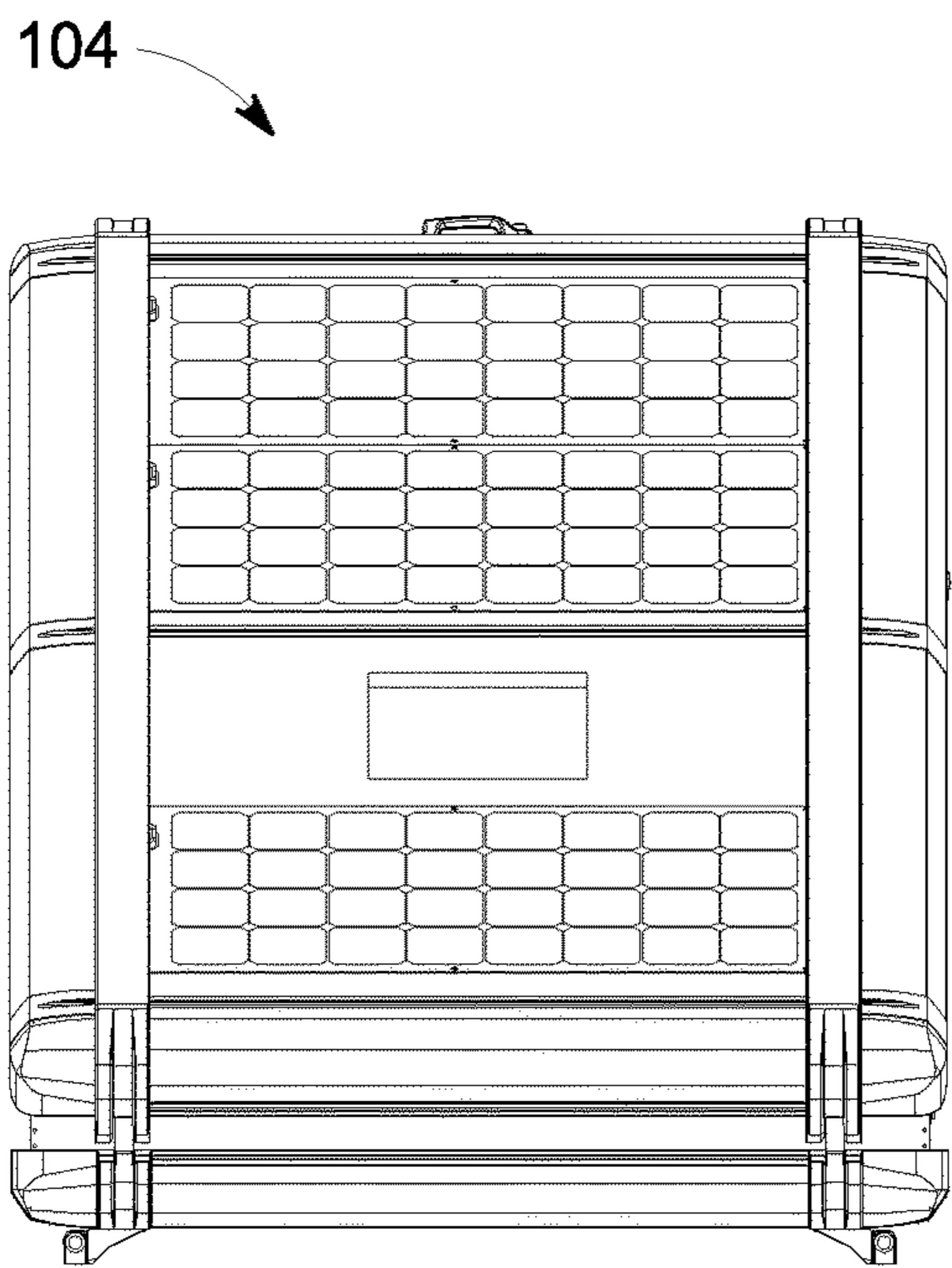
FIG. 41
