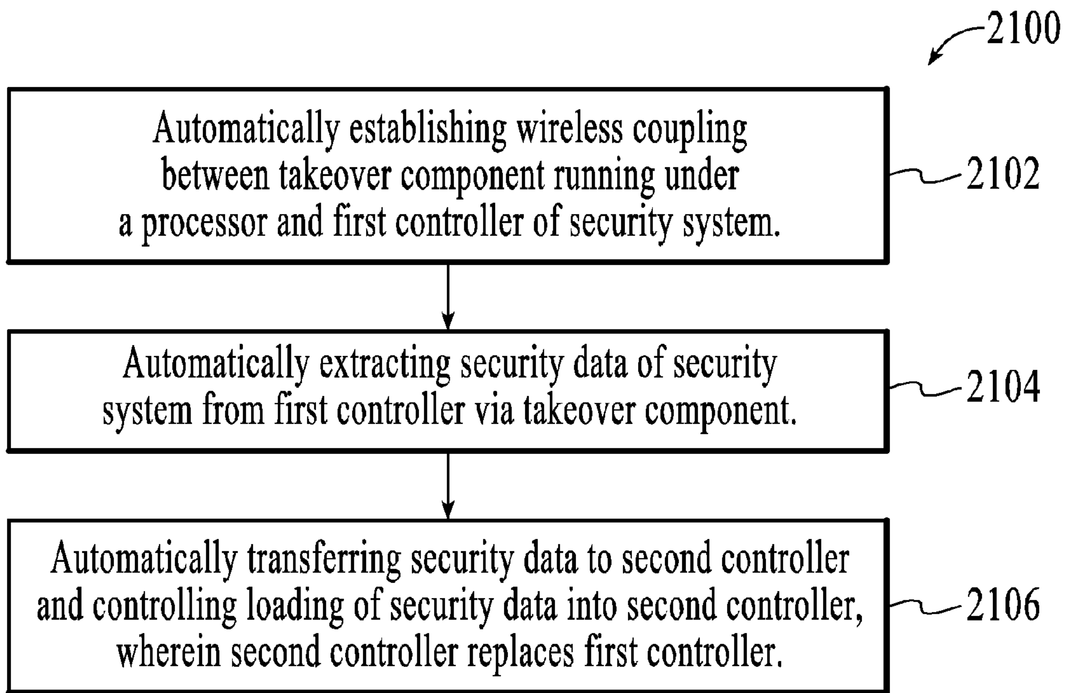
FIG.21
