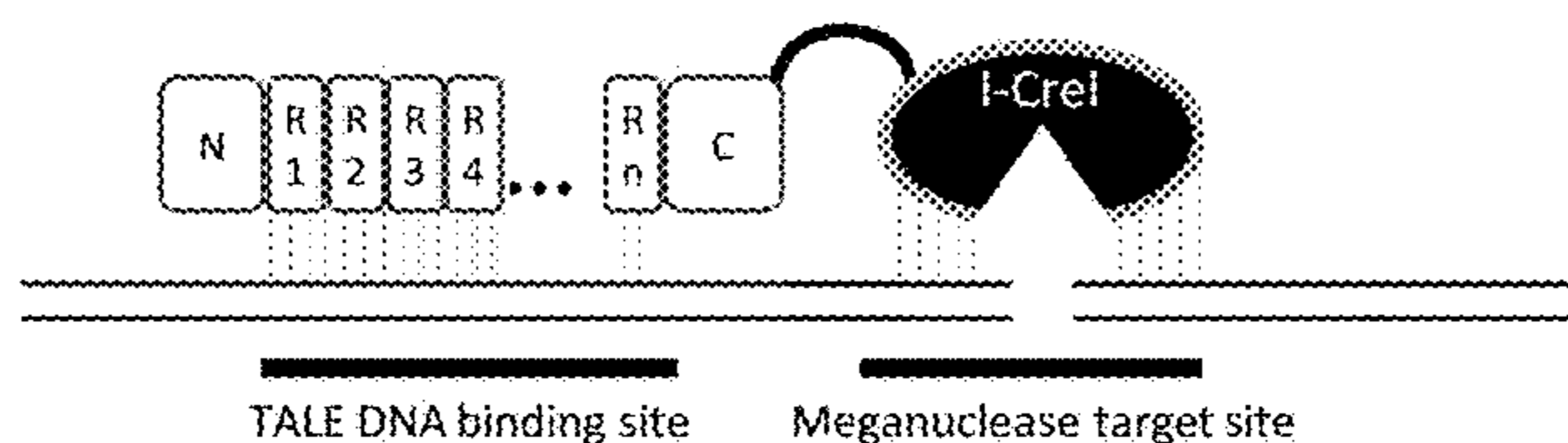
TALE::Crel prototype
