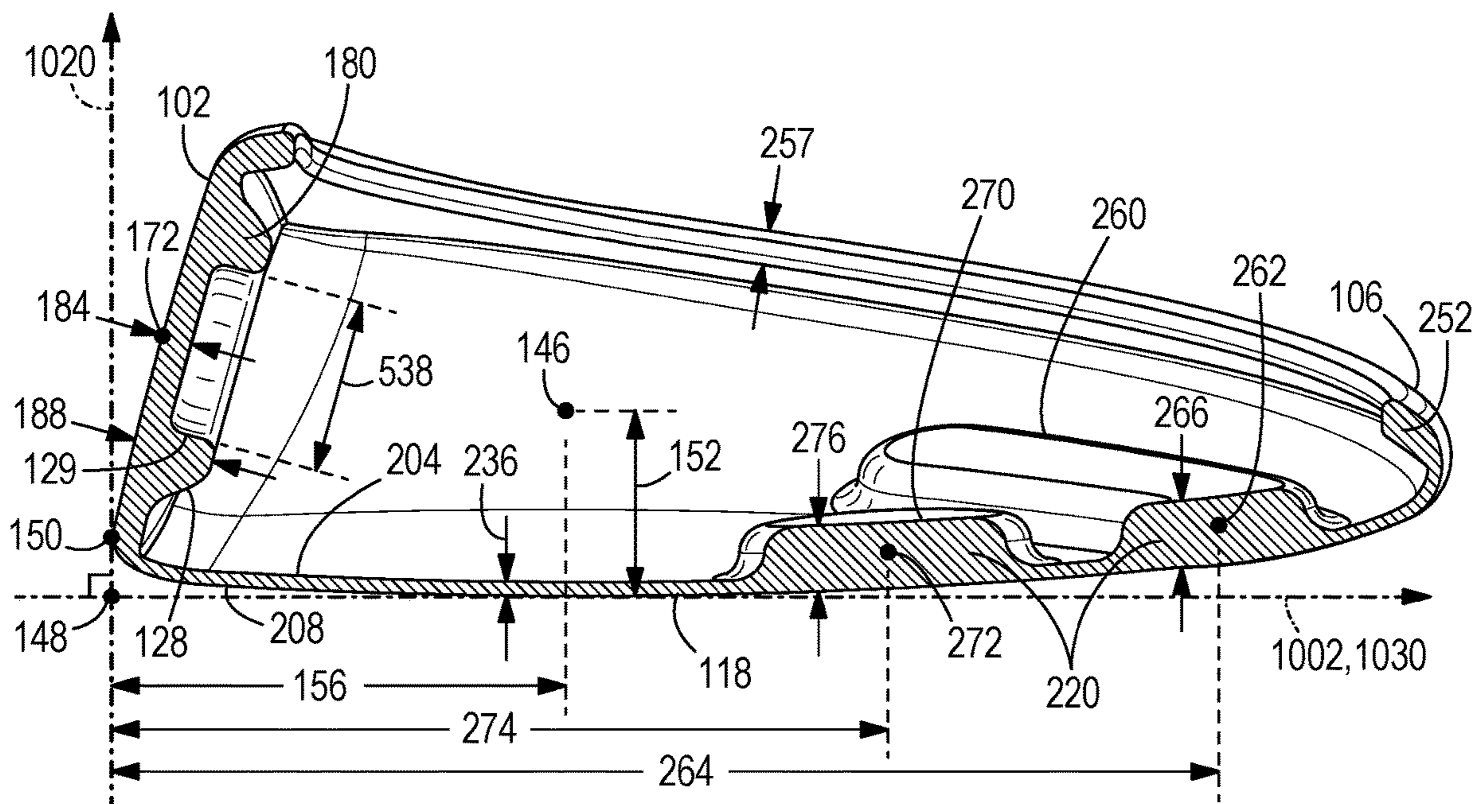
FIG. 6 Section A-A
