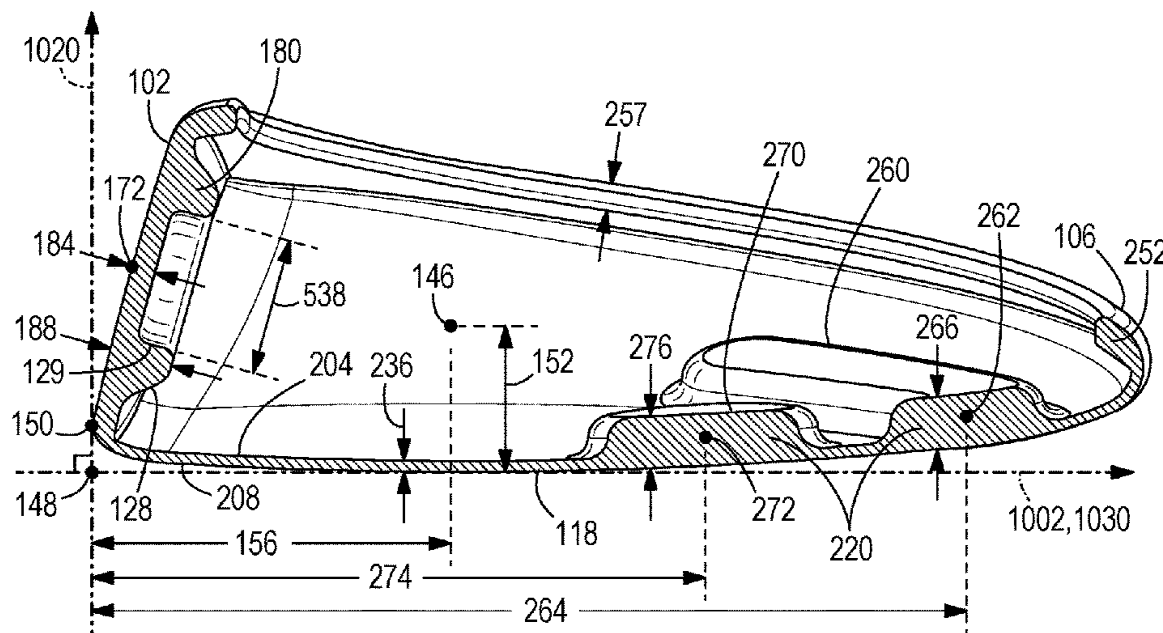
Section A-A
