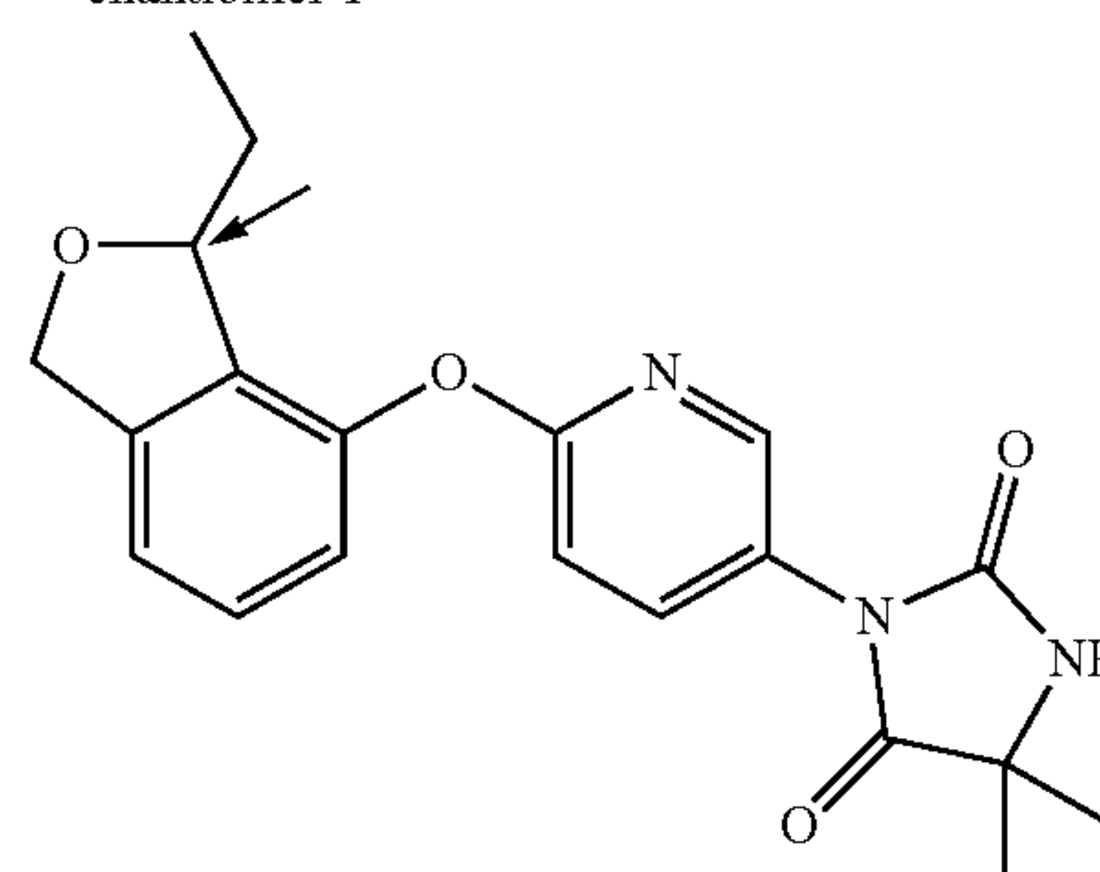
enantiomer 1
