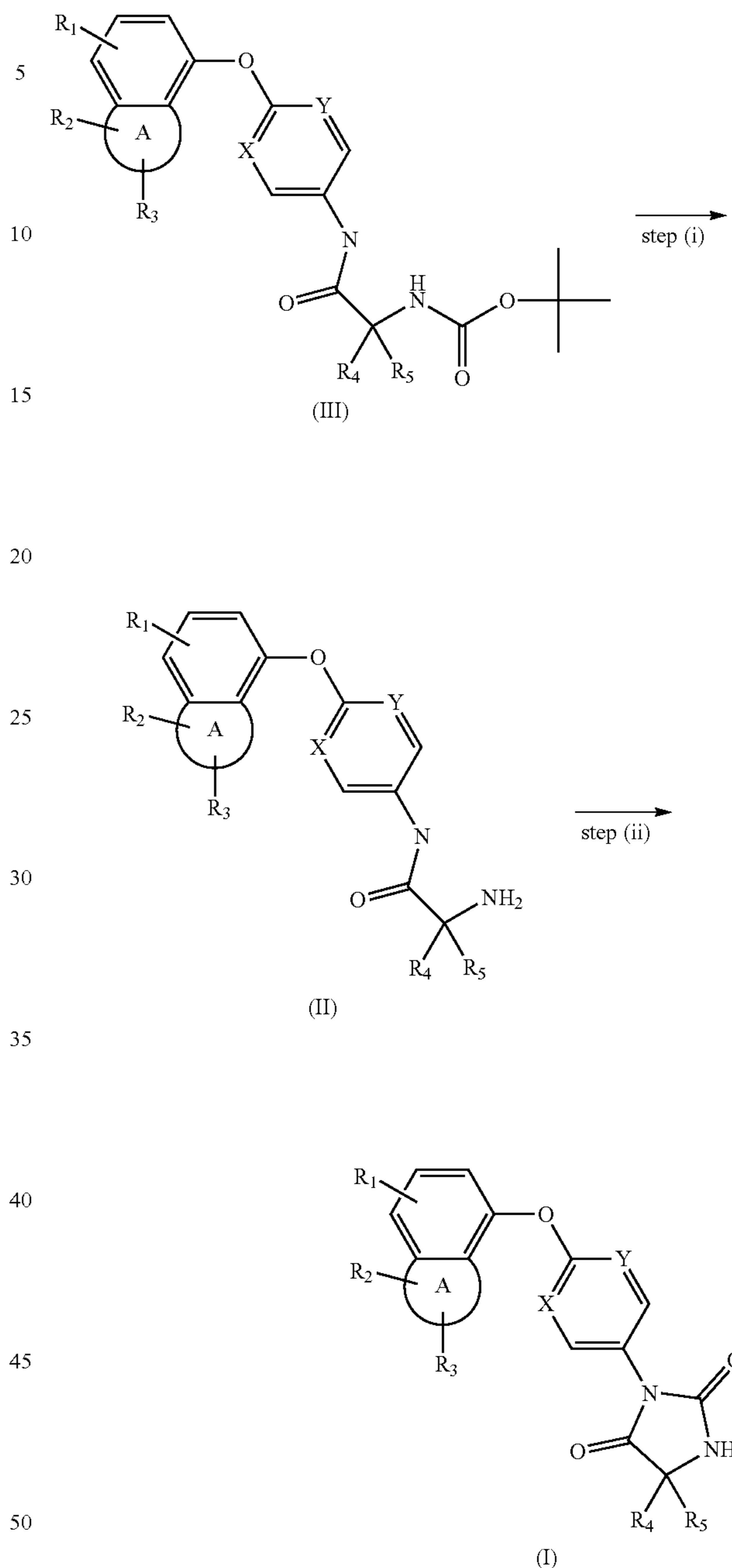
Scheme 1a
