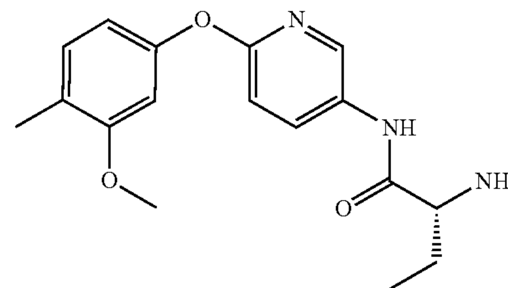
(2R)-2-amino-N-(6-{{[4-methyl-3-(methoxy)phenyl]oxy}}-3-pyridinyl)butanamide
