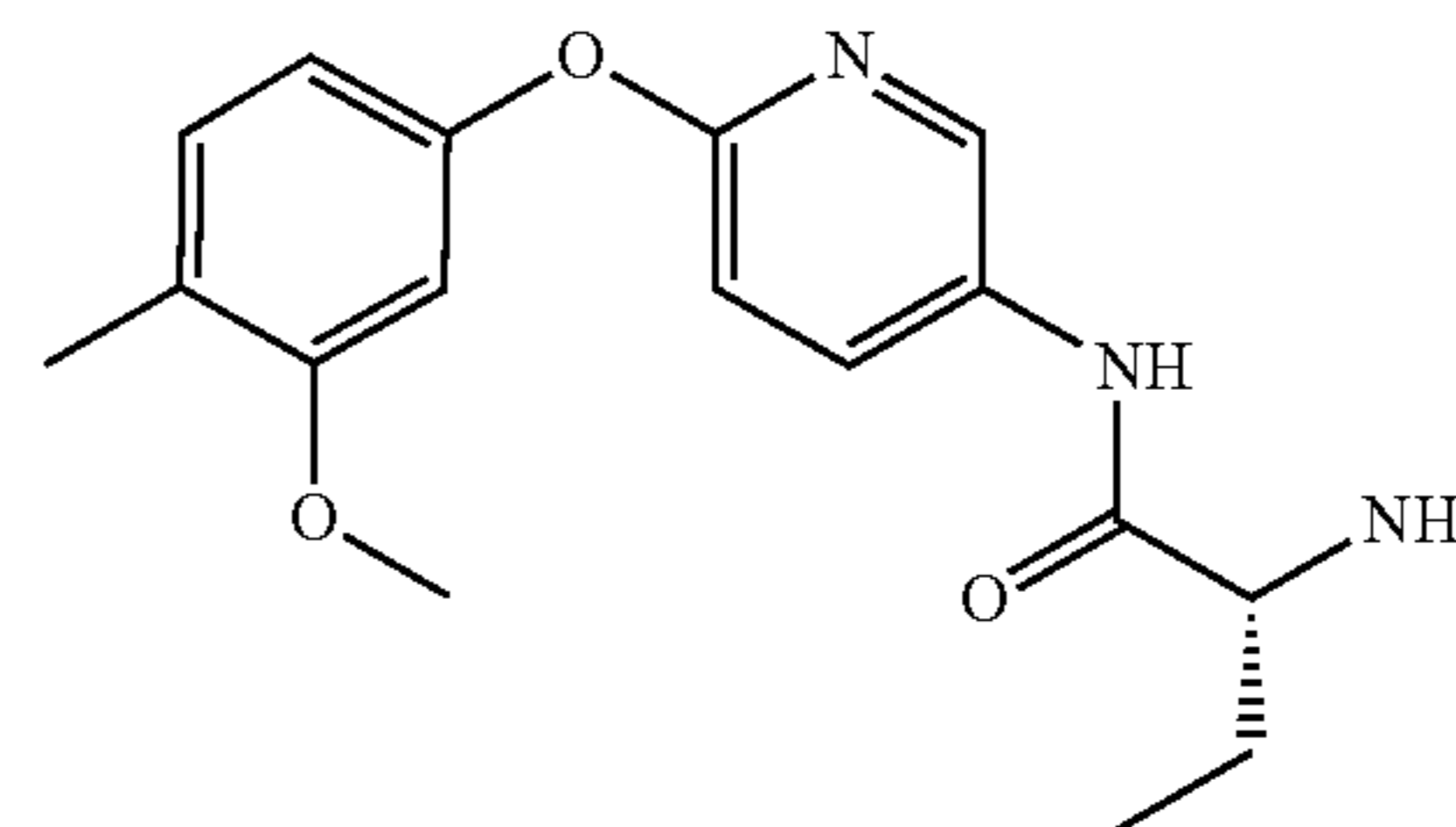
(2R)-2-amino-N-(6-{{[4-methyl-3-(methoxy)phenyl]oxy}}-3-pyridinyl)butanamide
