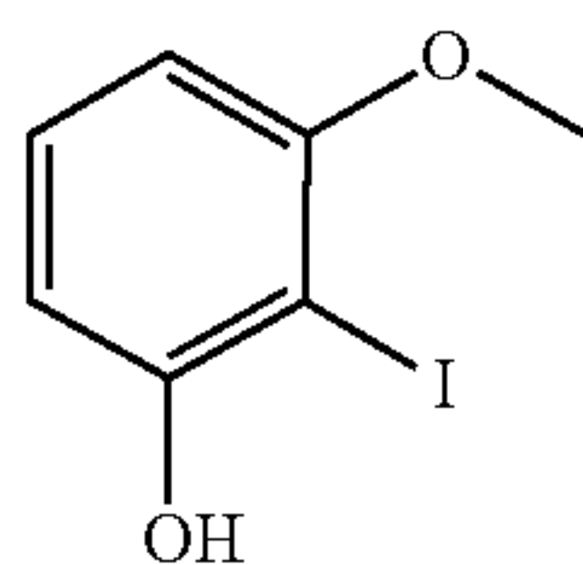
2-iodo-3-(methoxy)phenol
