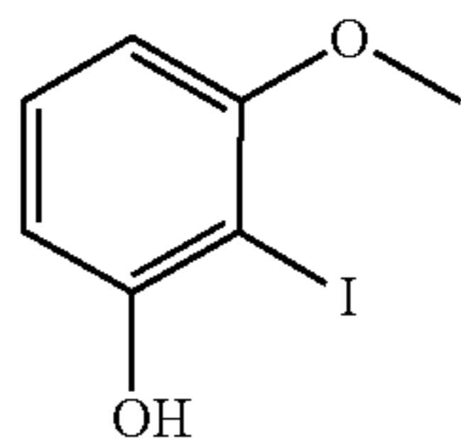
2-iodo-3-(methoxy)phenol
