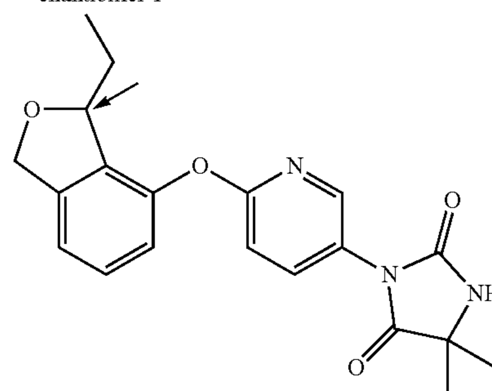
enantiomer 1
