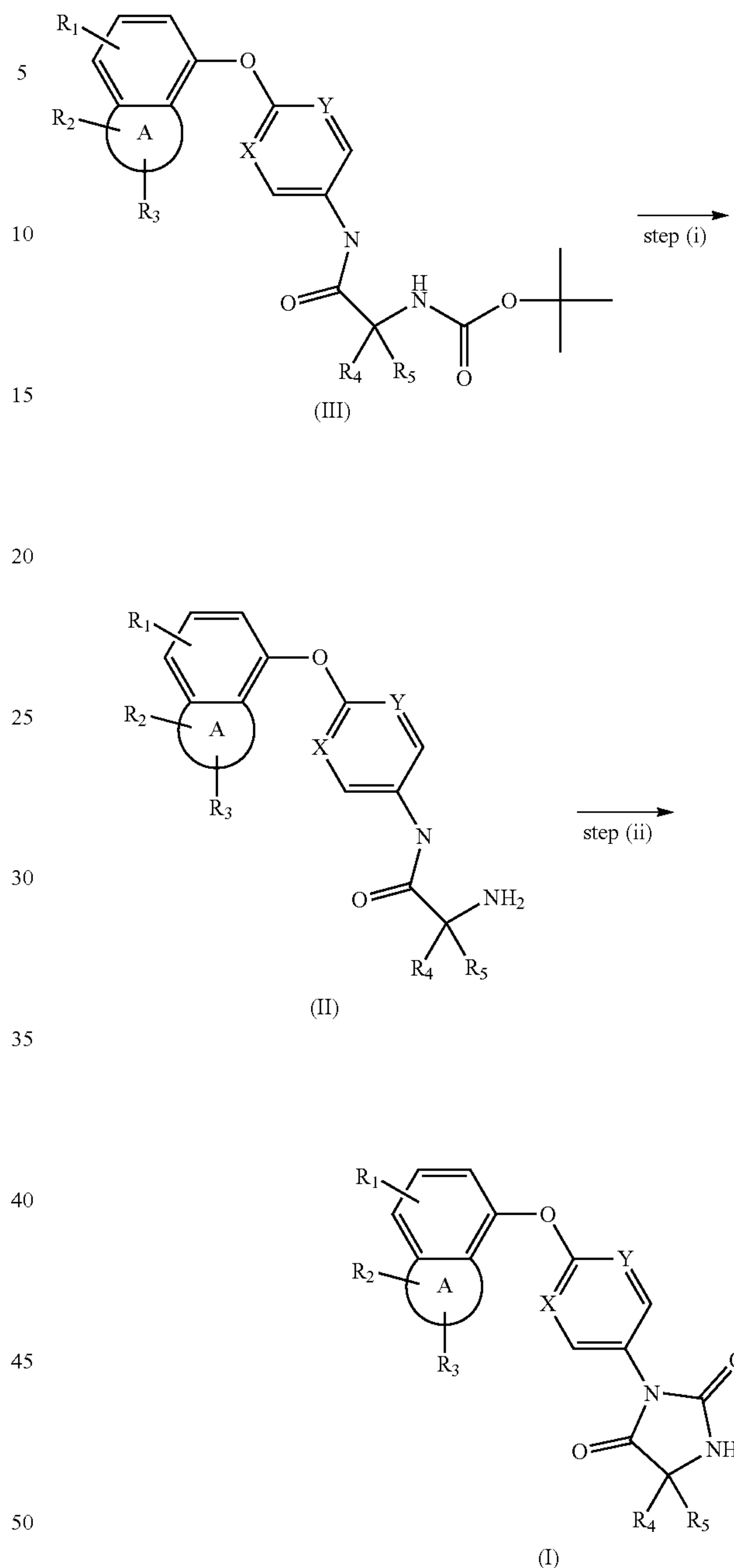
Scheme 1a
