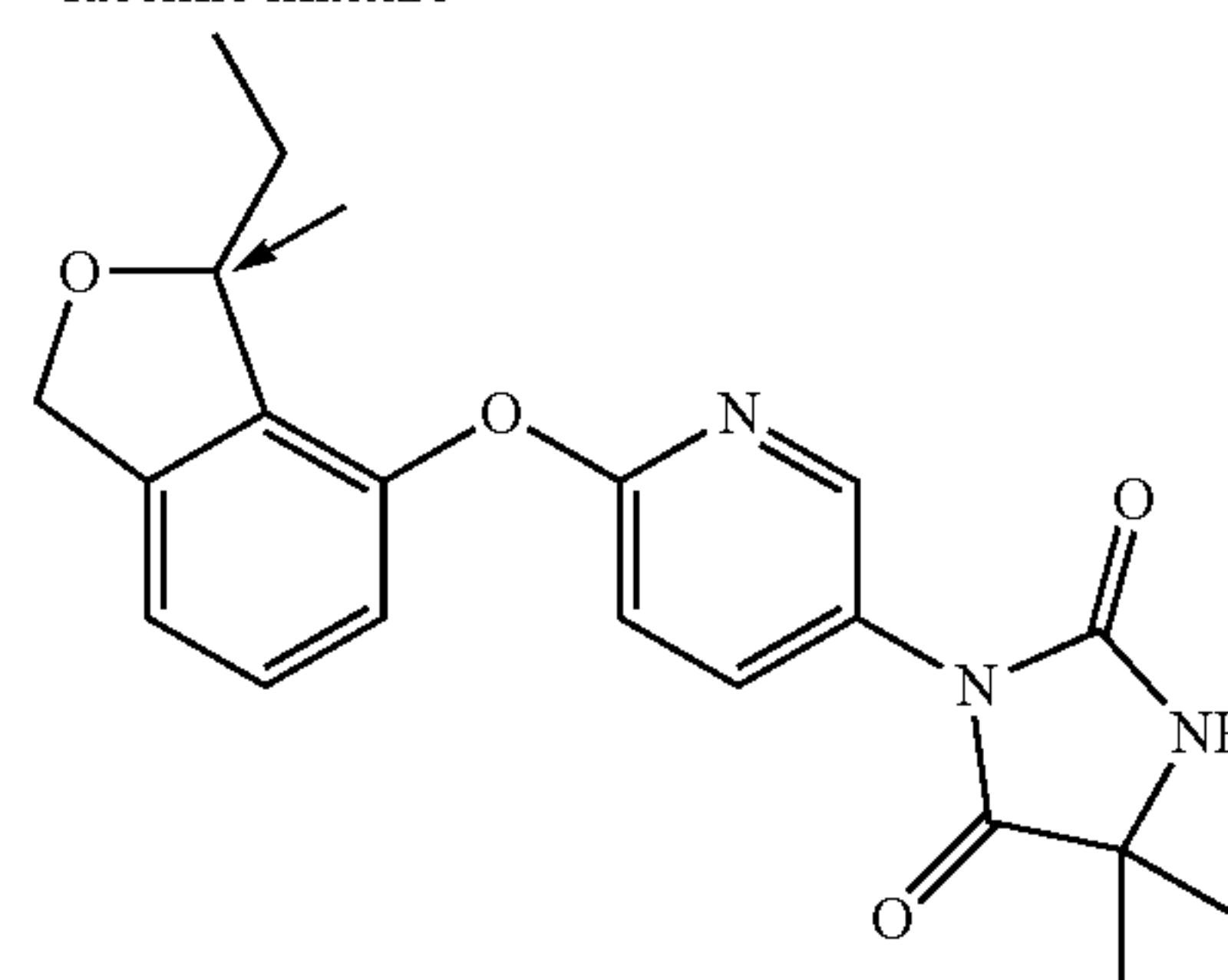
enantiomer 1
