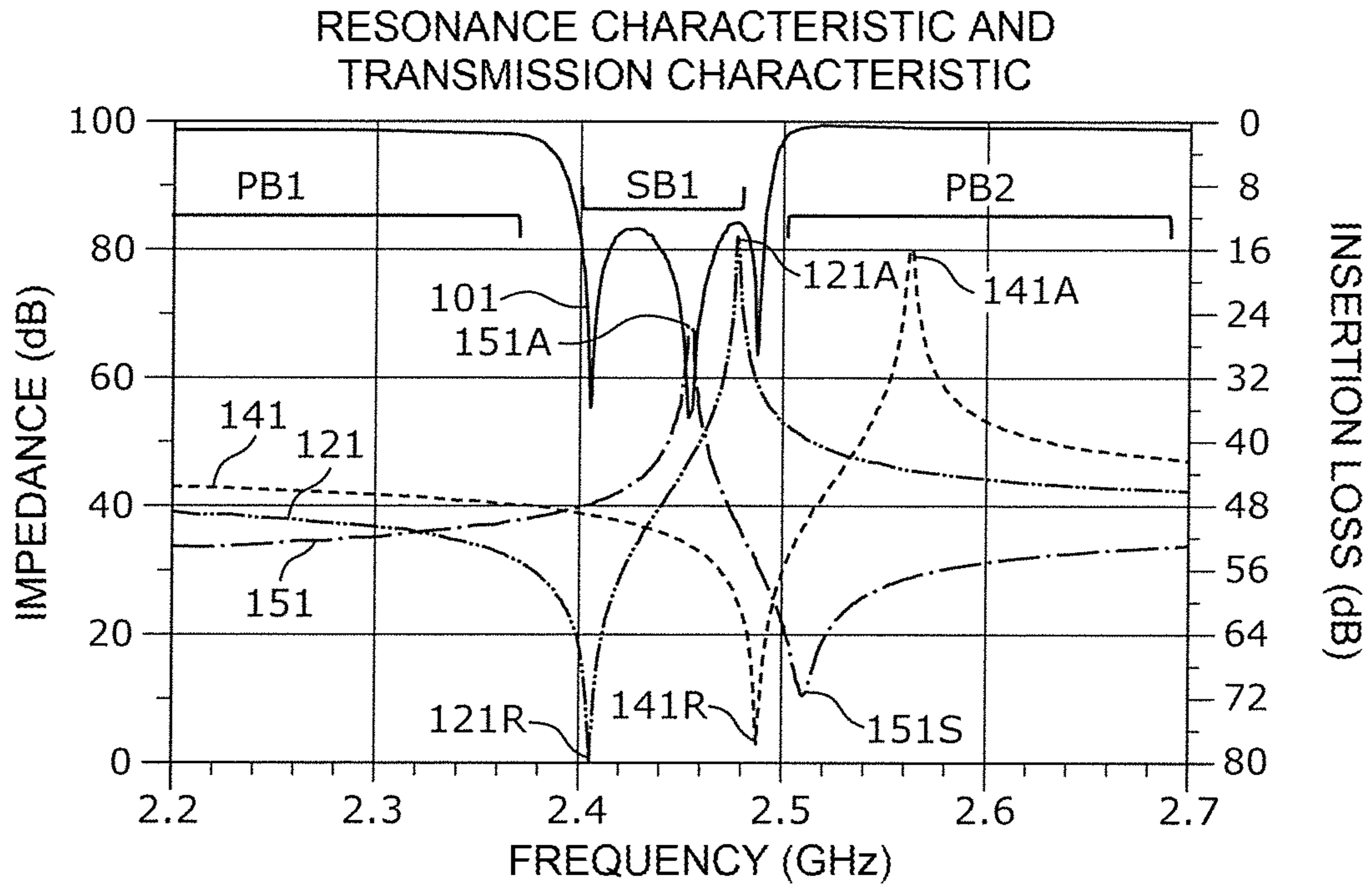
FIG. 5A
