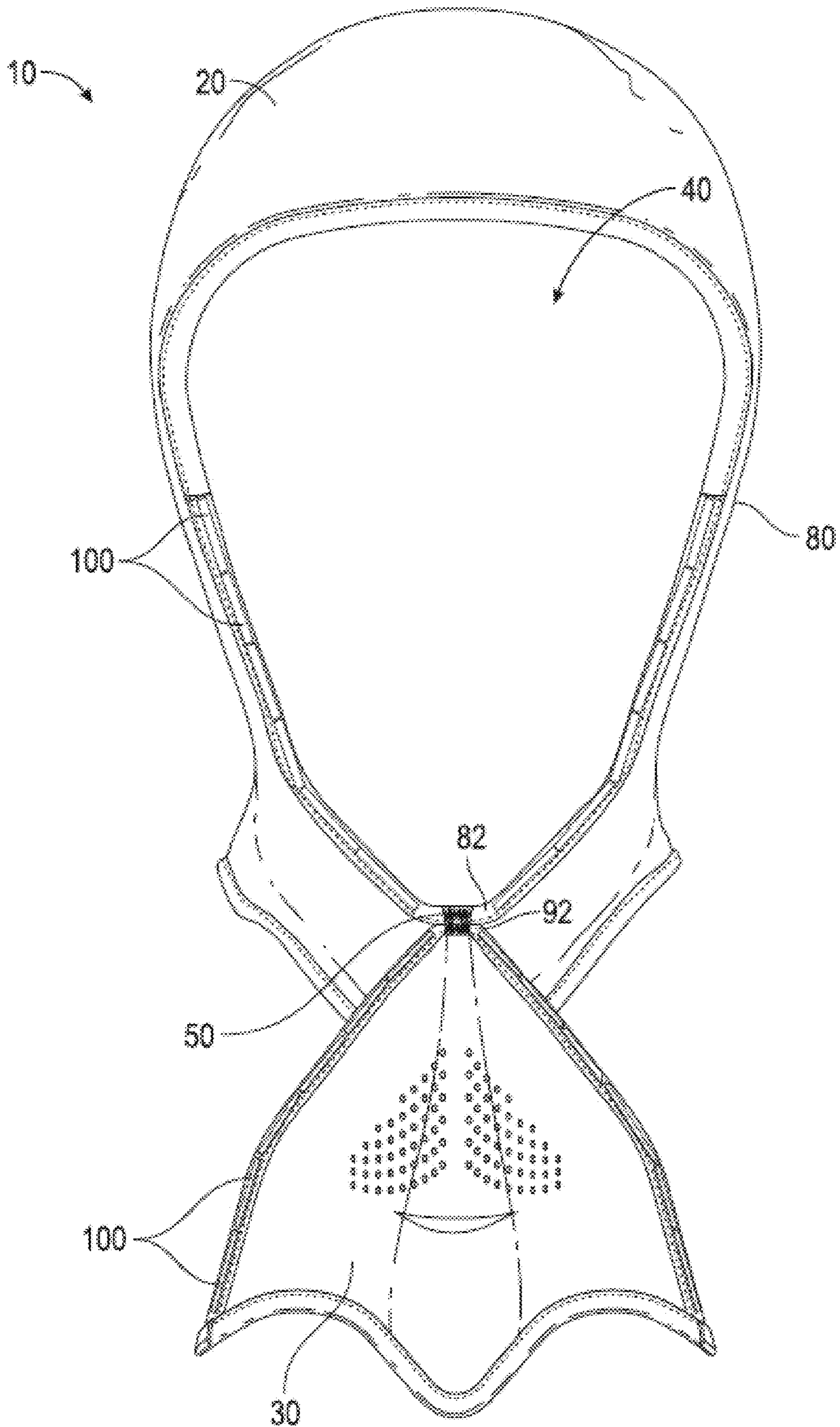
FIG. 2A
