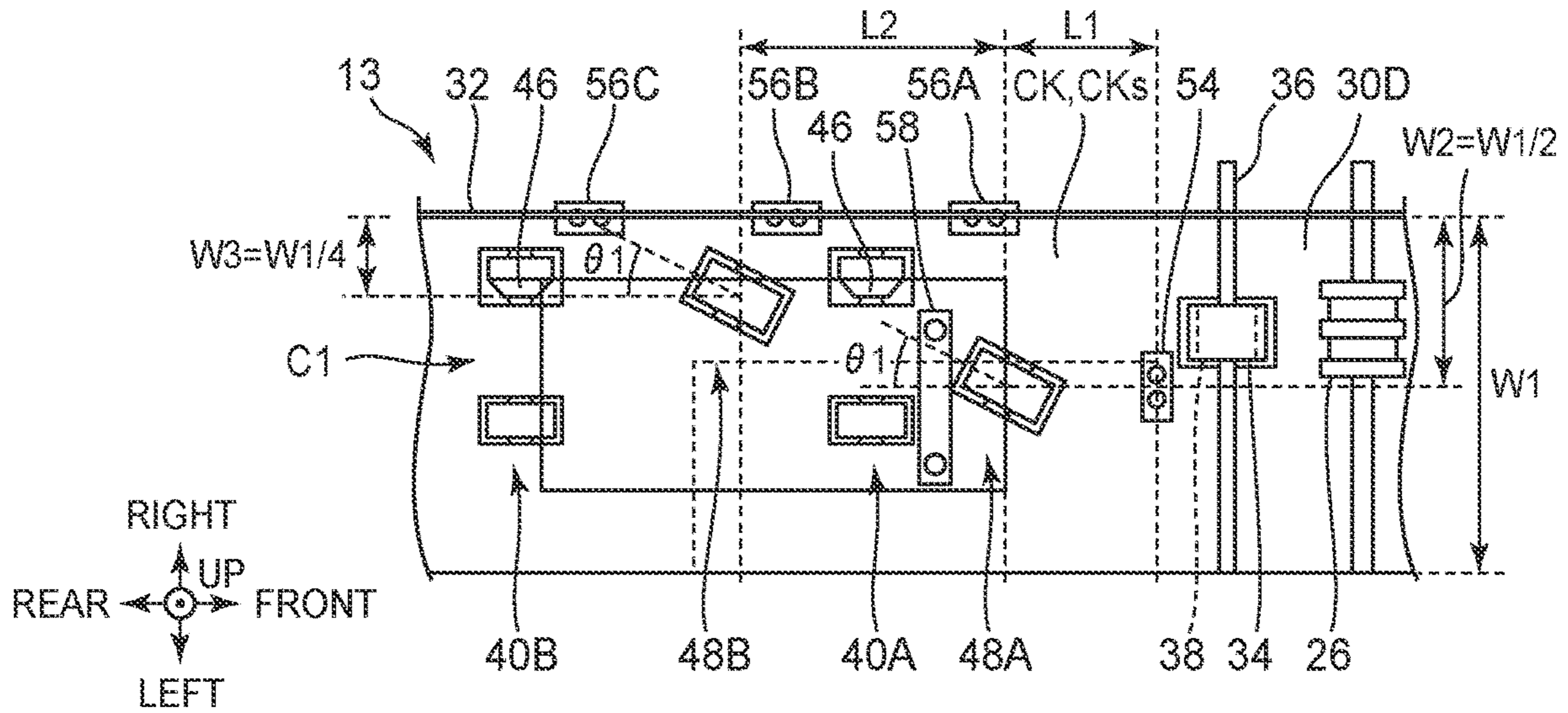
FIG. 10
