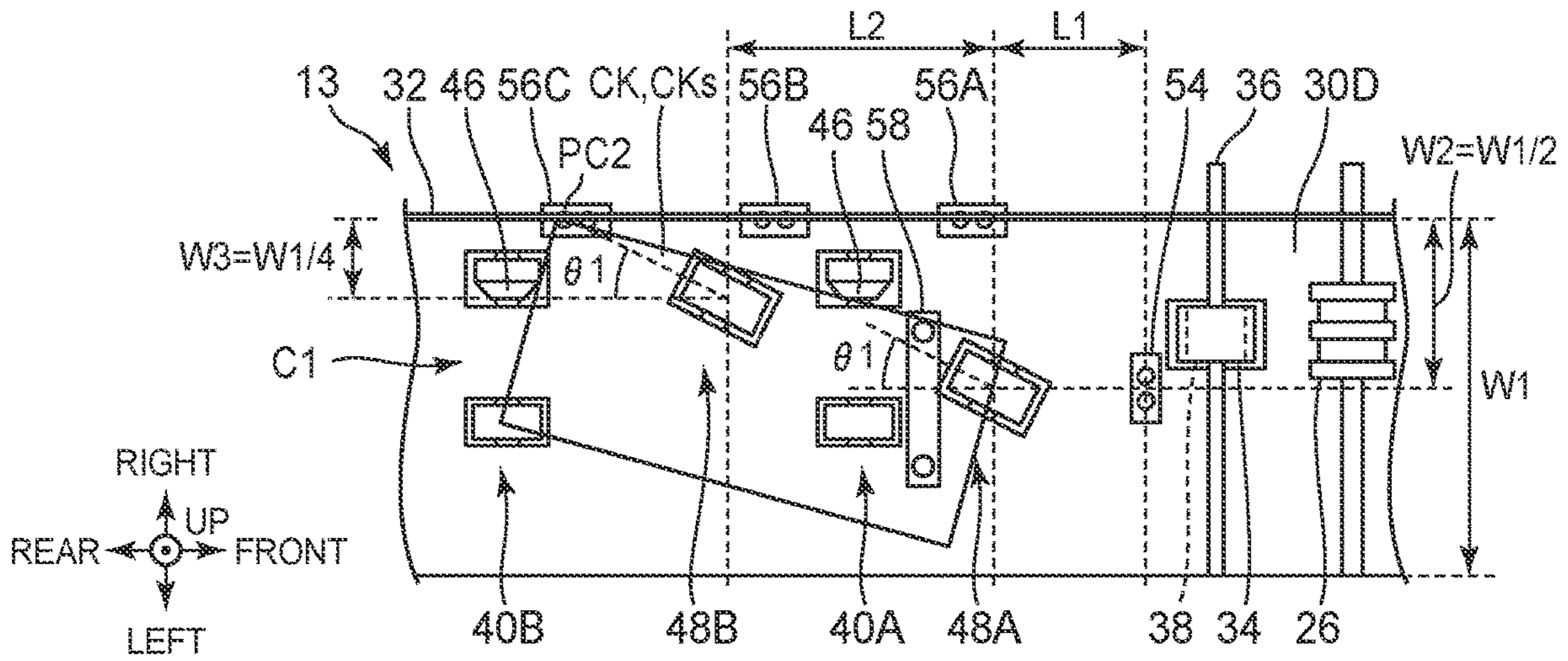
FIG. 16
