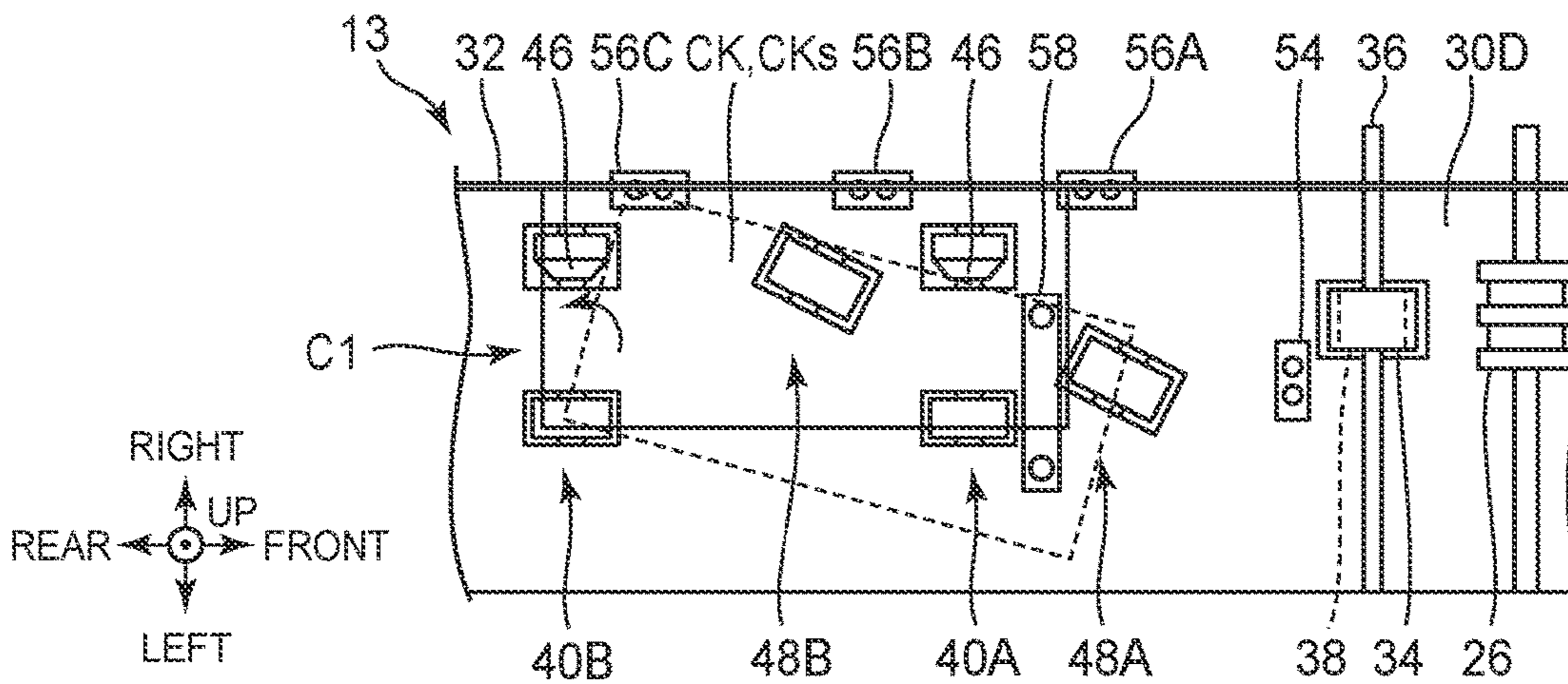
FIG. 18
