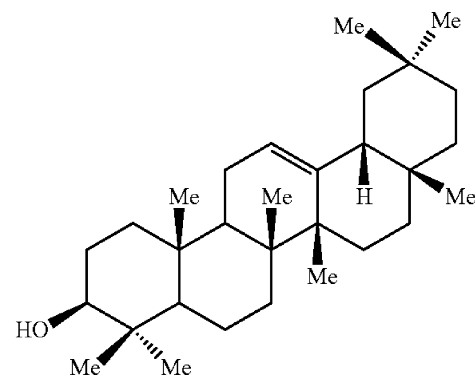
Beta-amyrin
