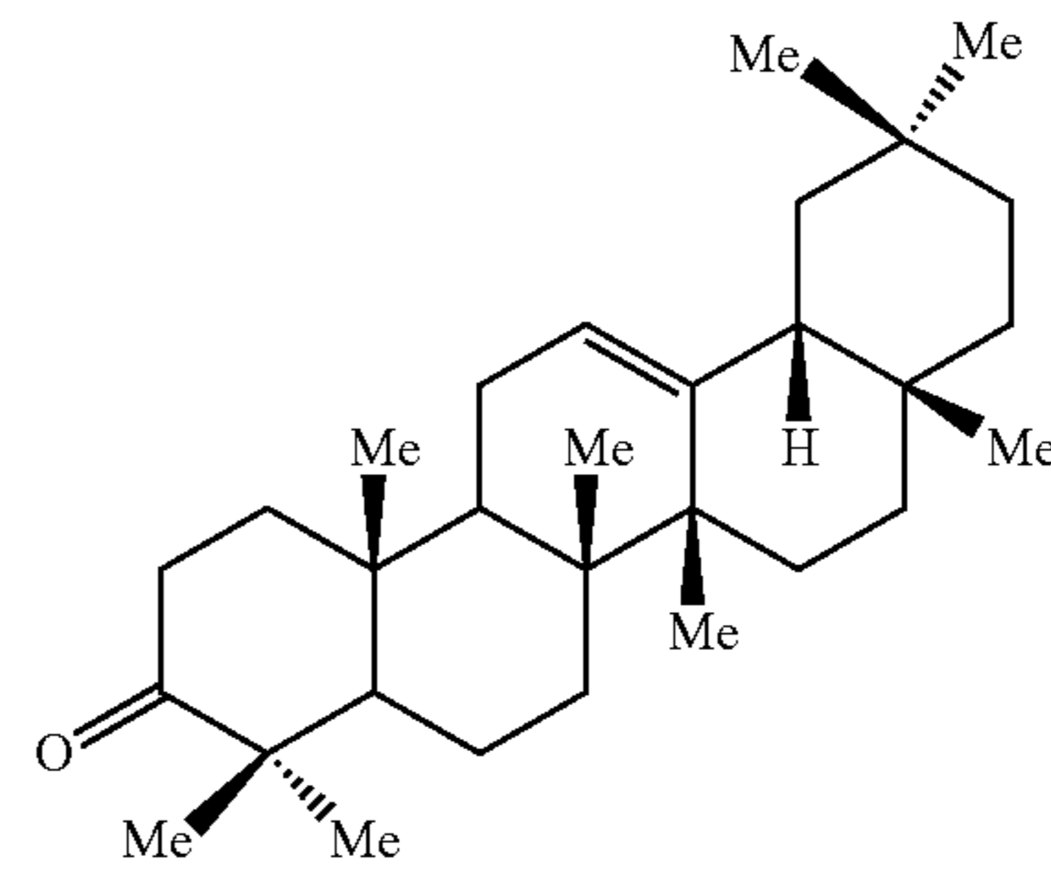
Beta-amyrone
