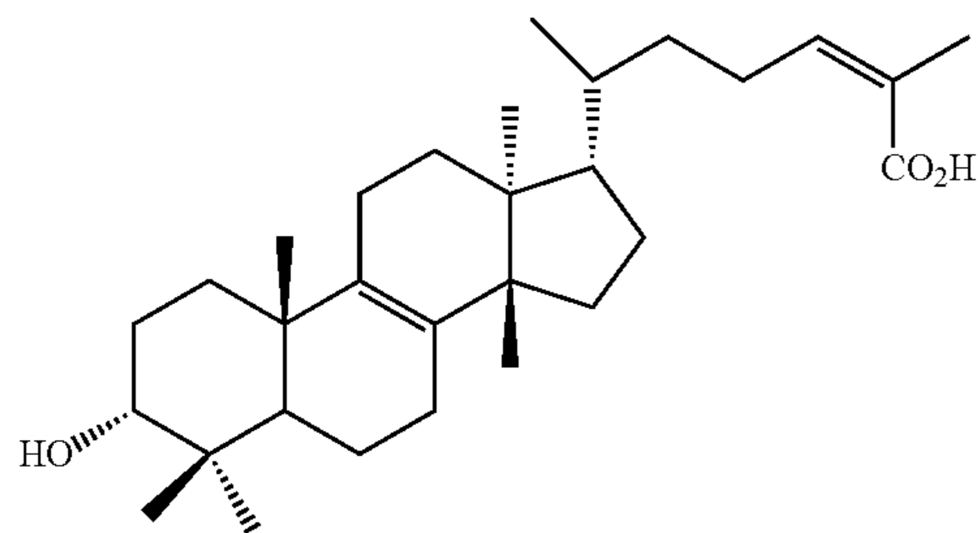
epi-IMLA
