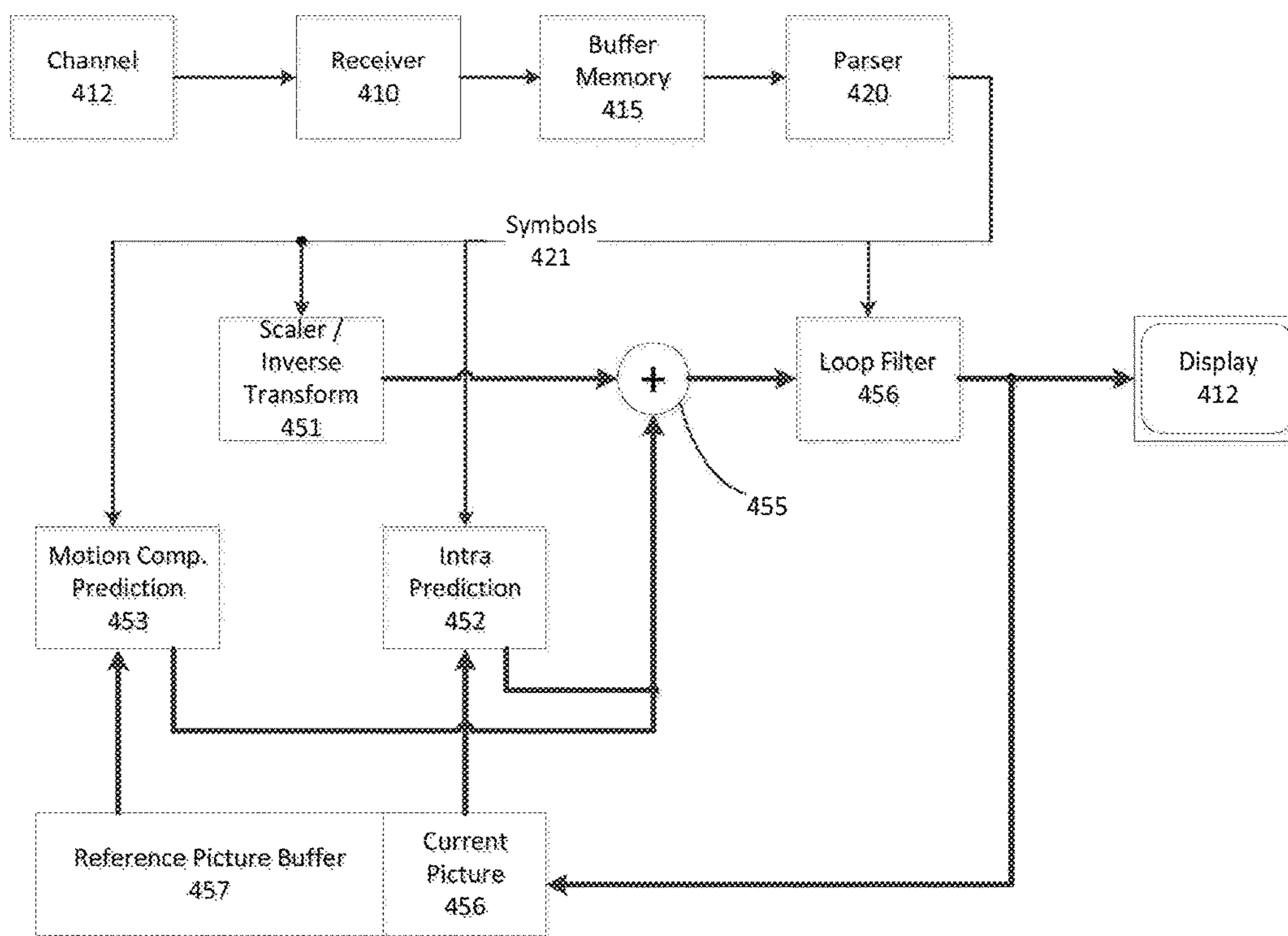
FIG. 4 Decoder 310
