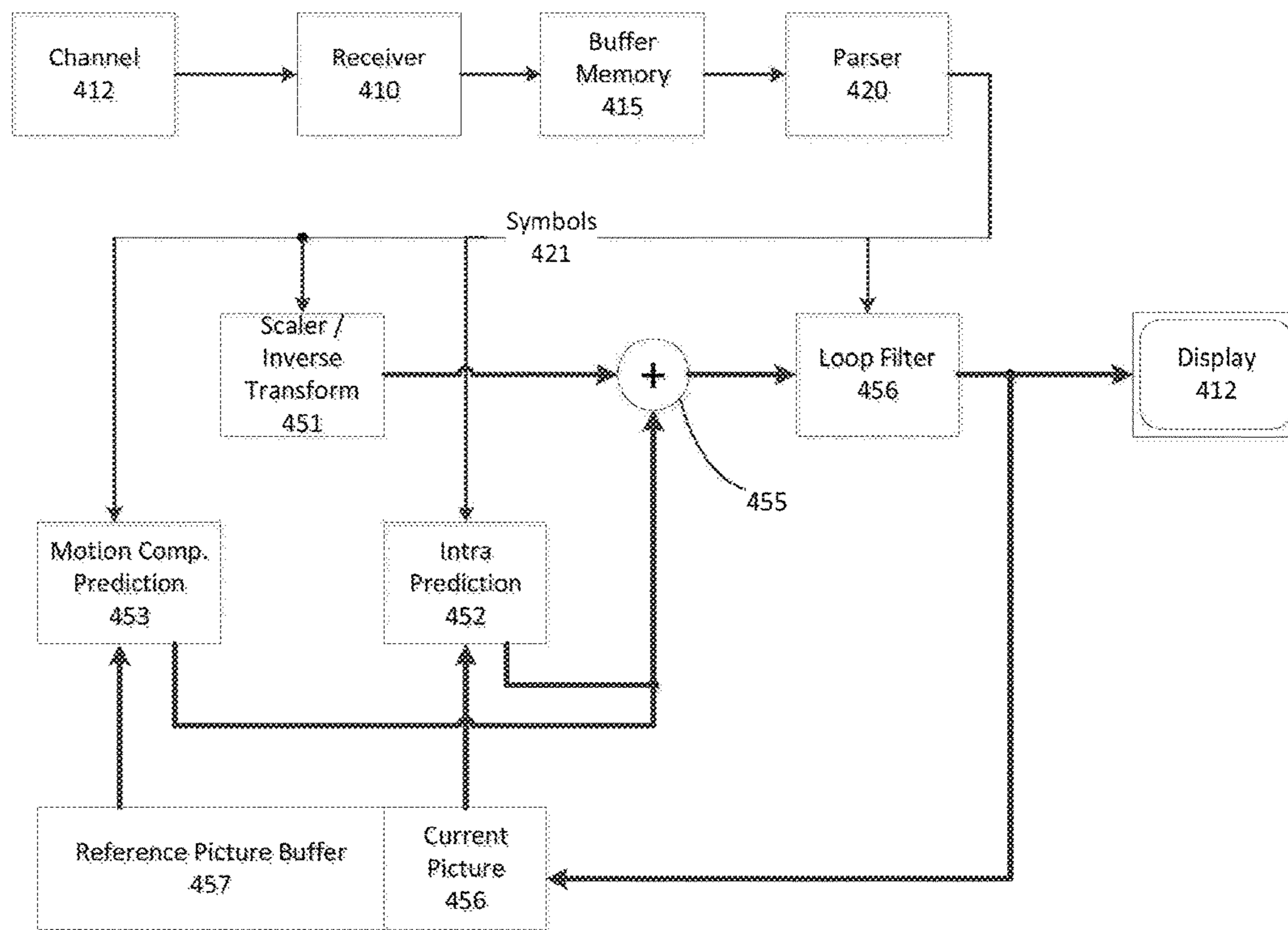
FIG. 4 Decoder 310
