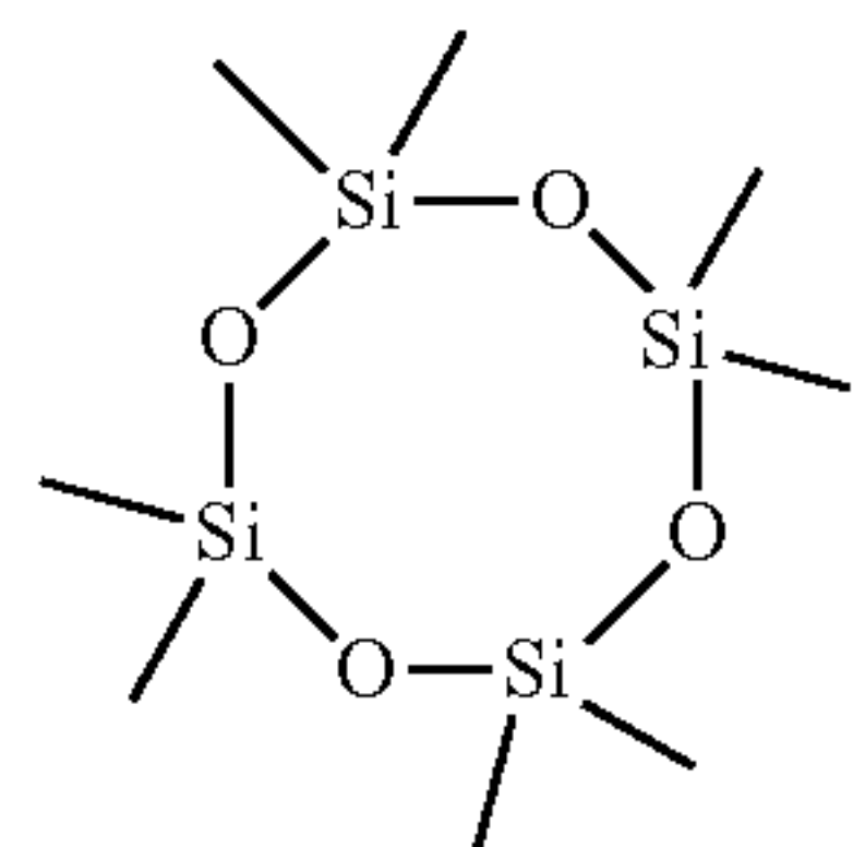
Octamethylcyclotetrasiloxane
