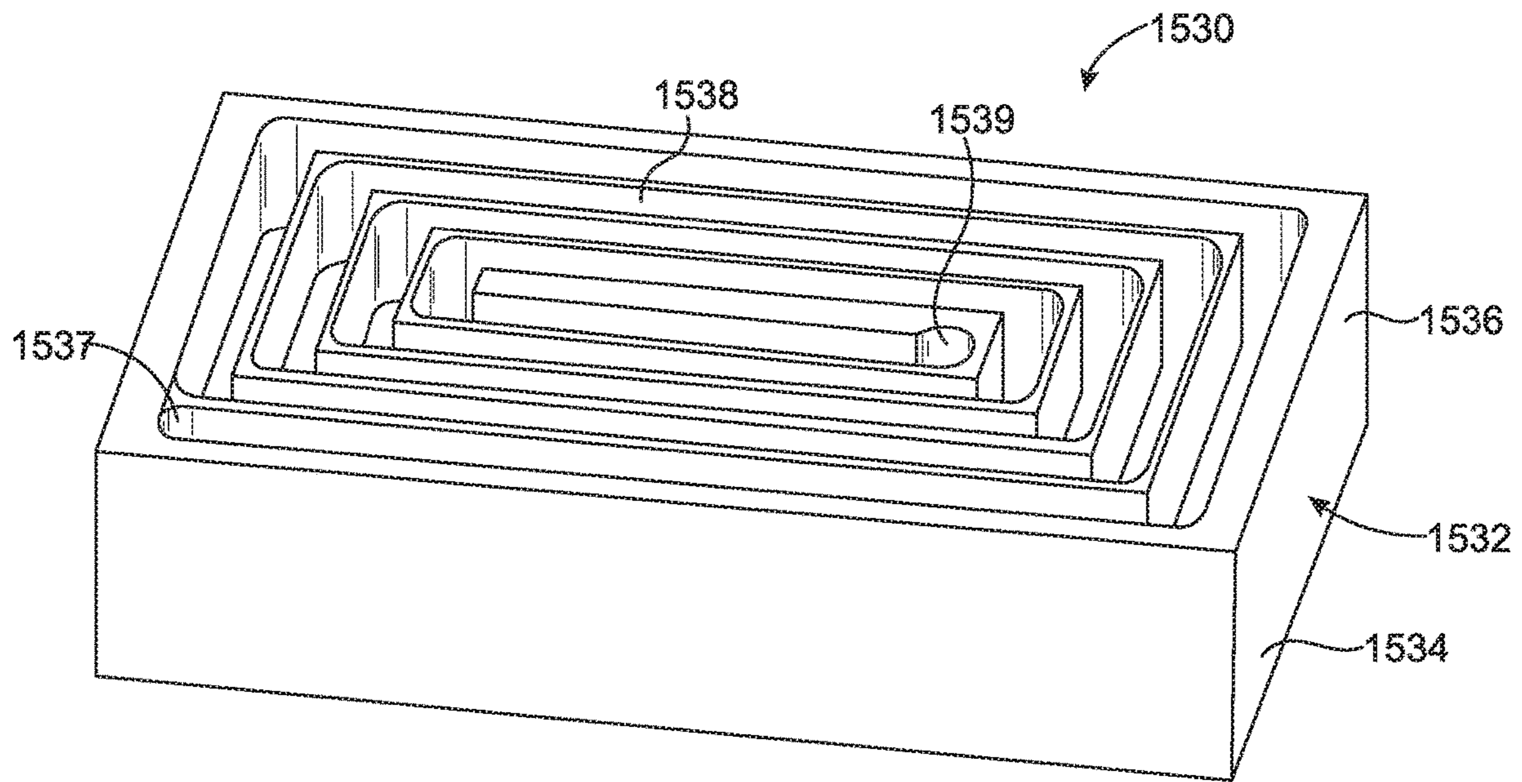
FIG. 13A
