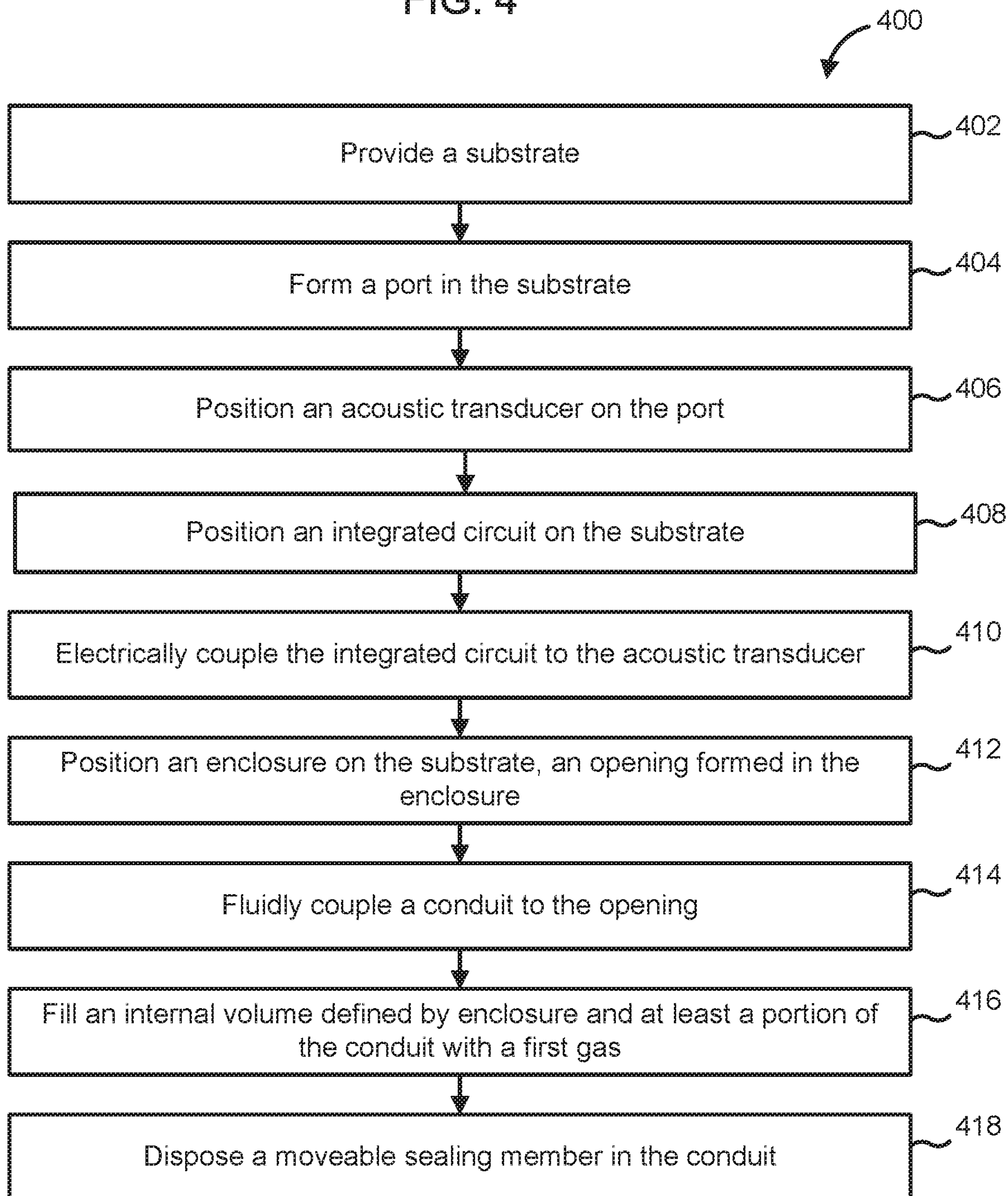
FIG. 4
