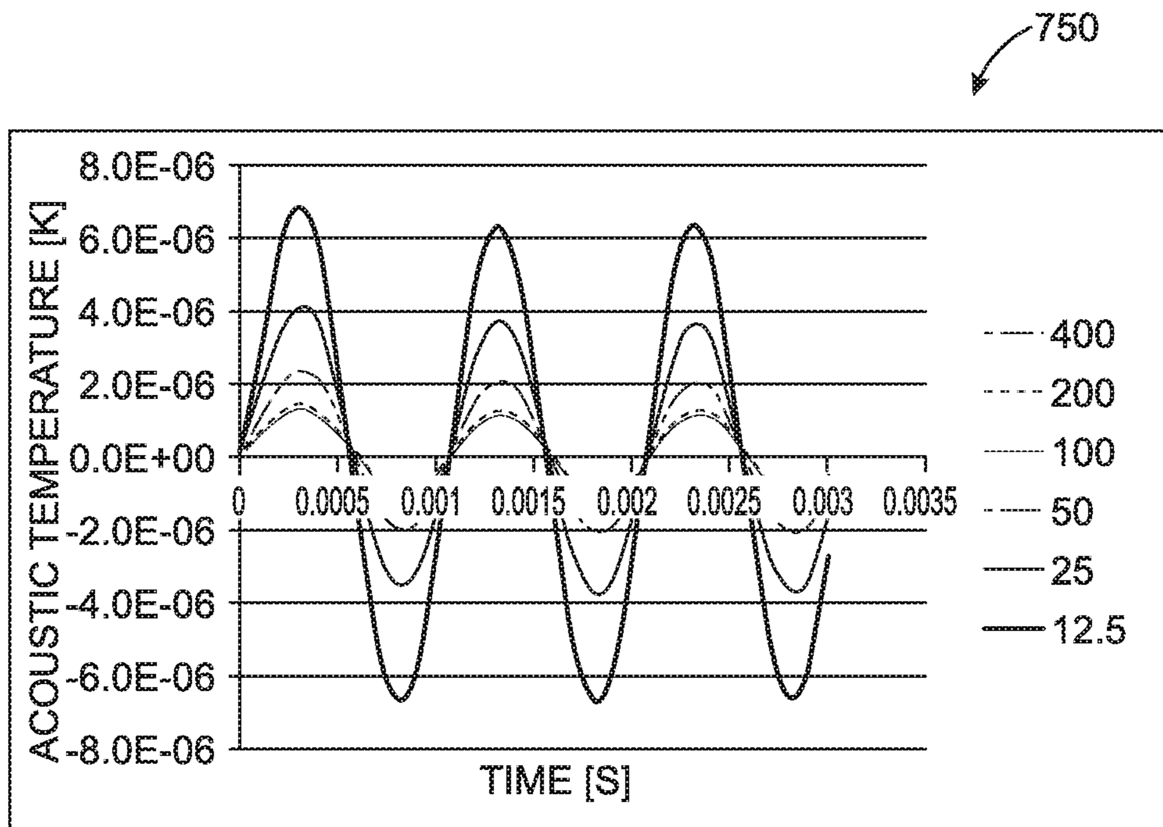
FIG. 7B
