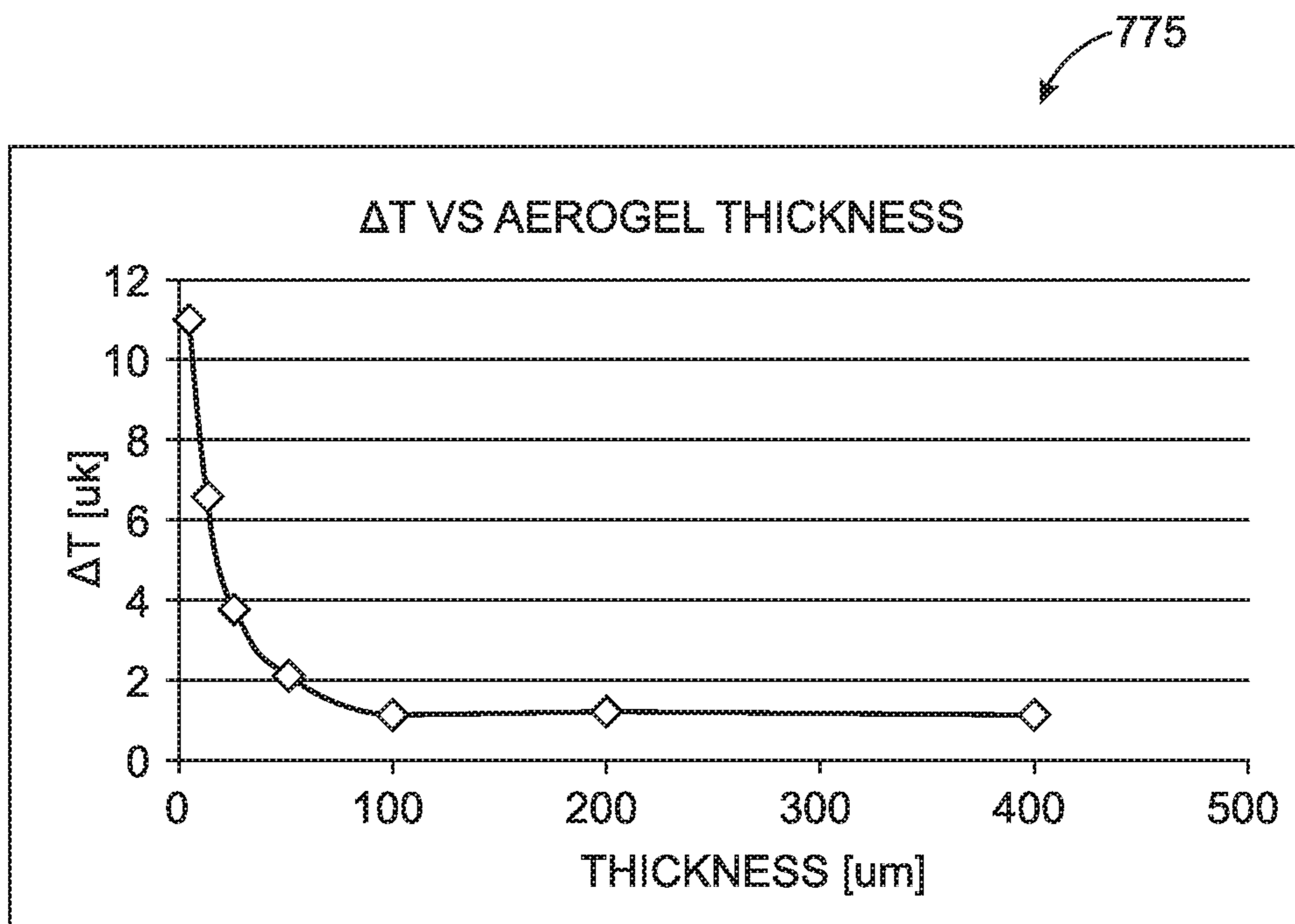
FIG. 7C
