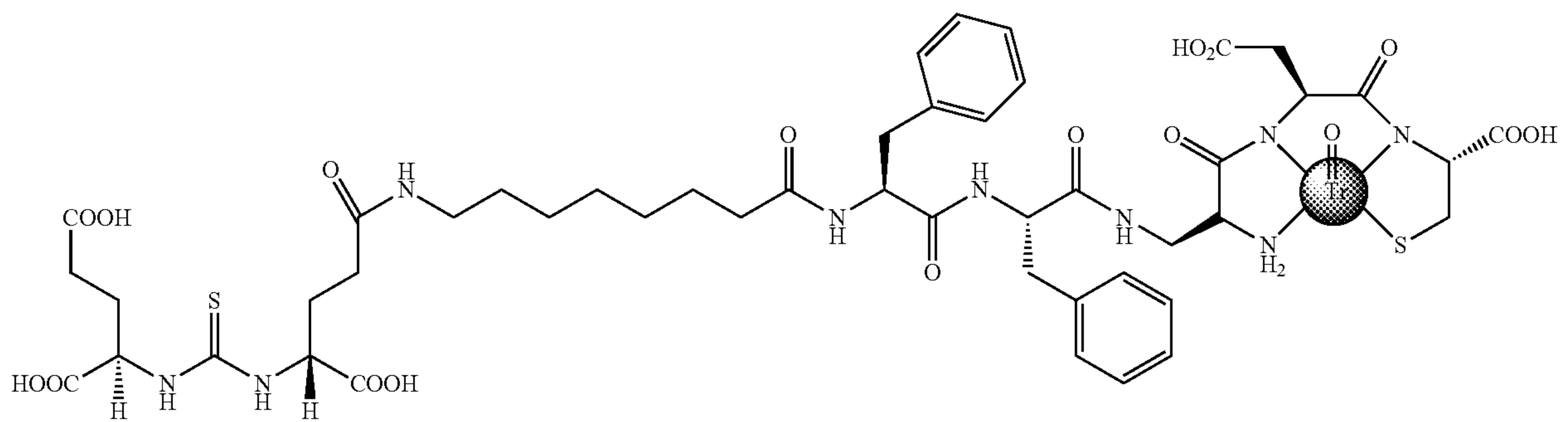
(15 atom linker)
