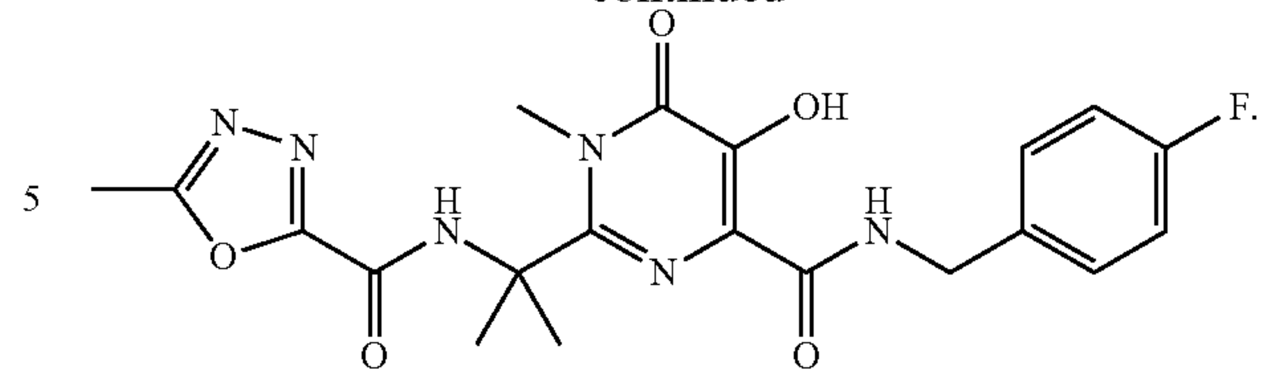
raltegravir (RAL)
