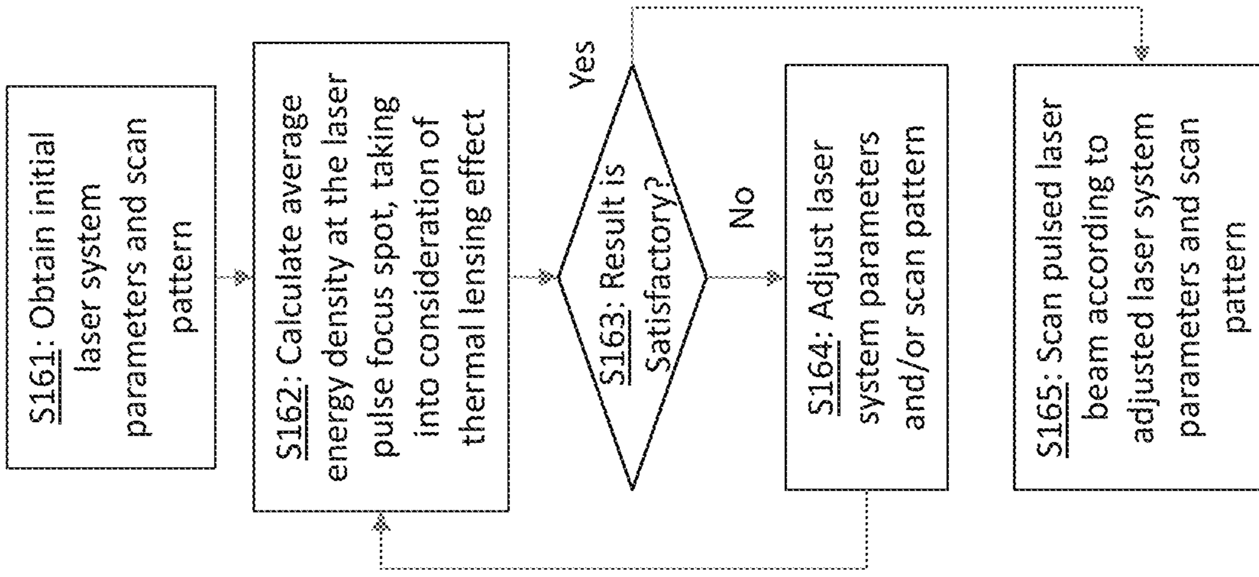
FIG. 16
