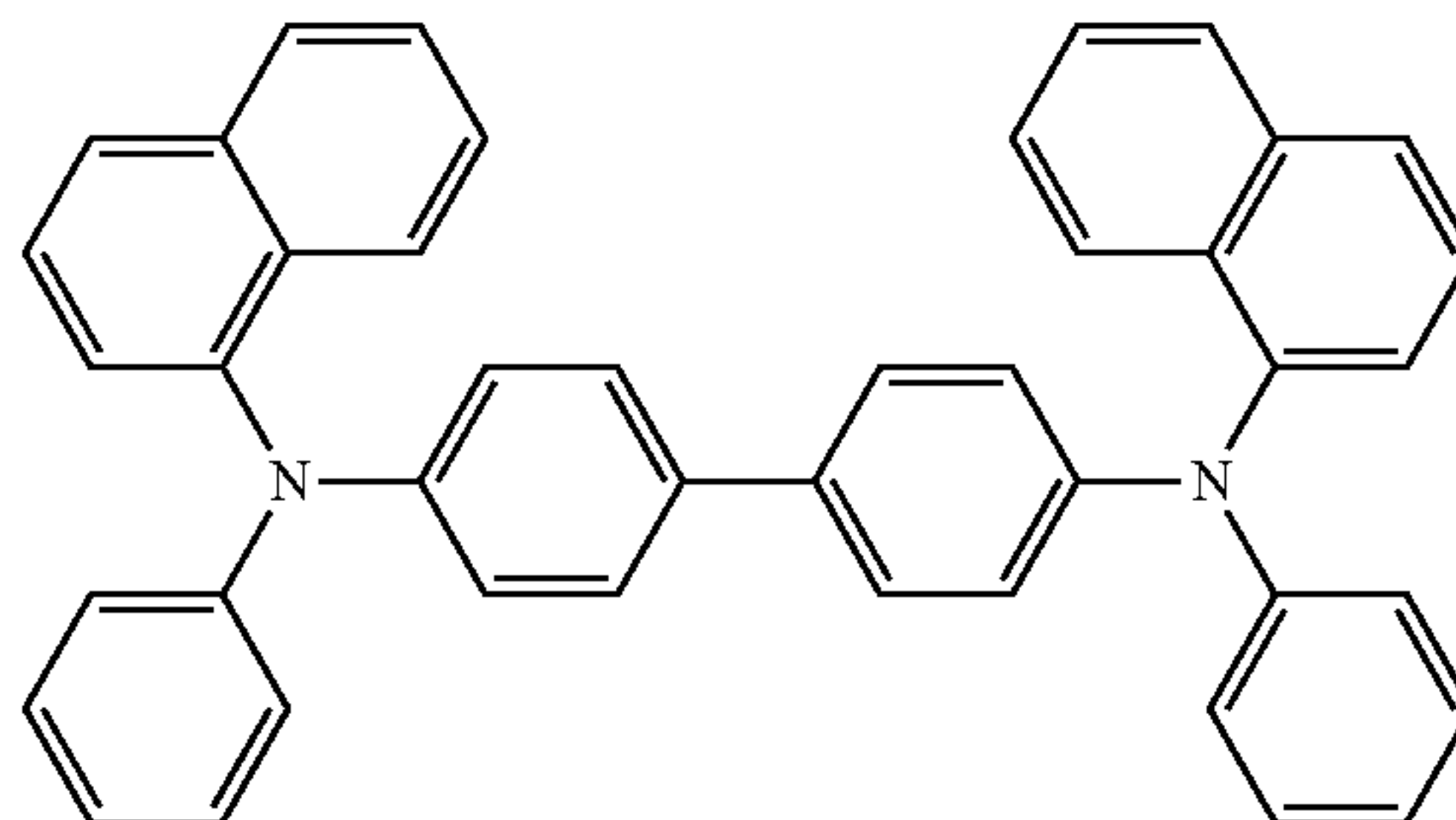
N 4 ,N 4' -di(naphthalen-1-yl)-N 4 ,N 4' -diphenyl-[1,1'-biphenyl]-4,4'-diamine
