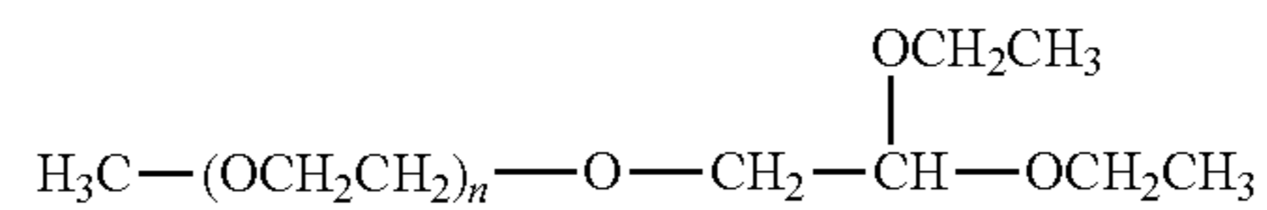
mPEG Acetal
