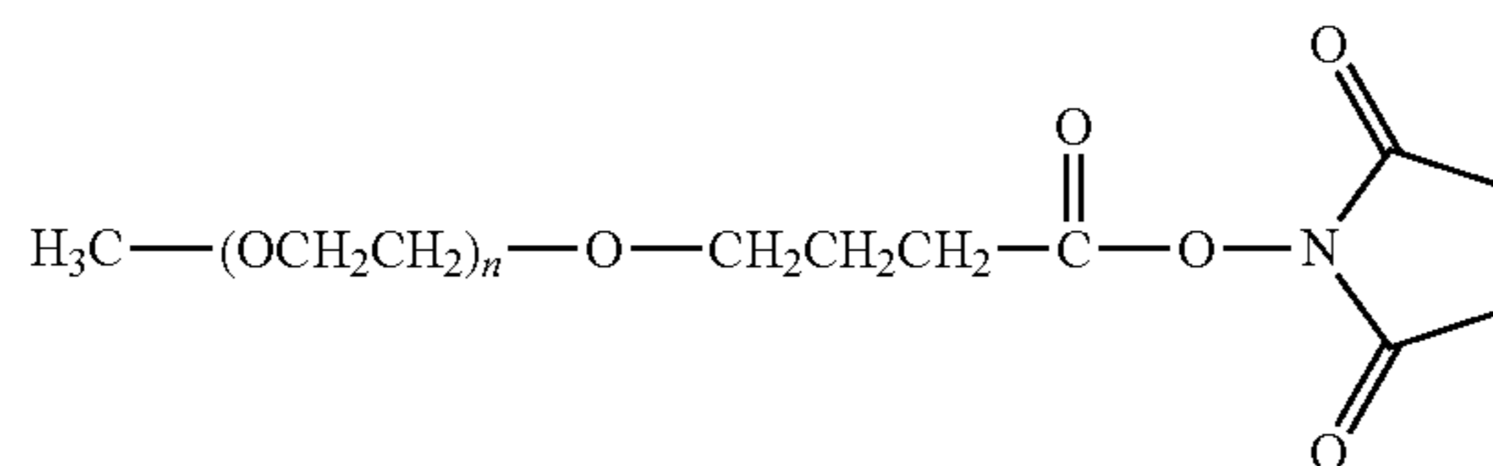
mPEG-Succinimidyl Butanoate
