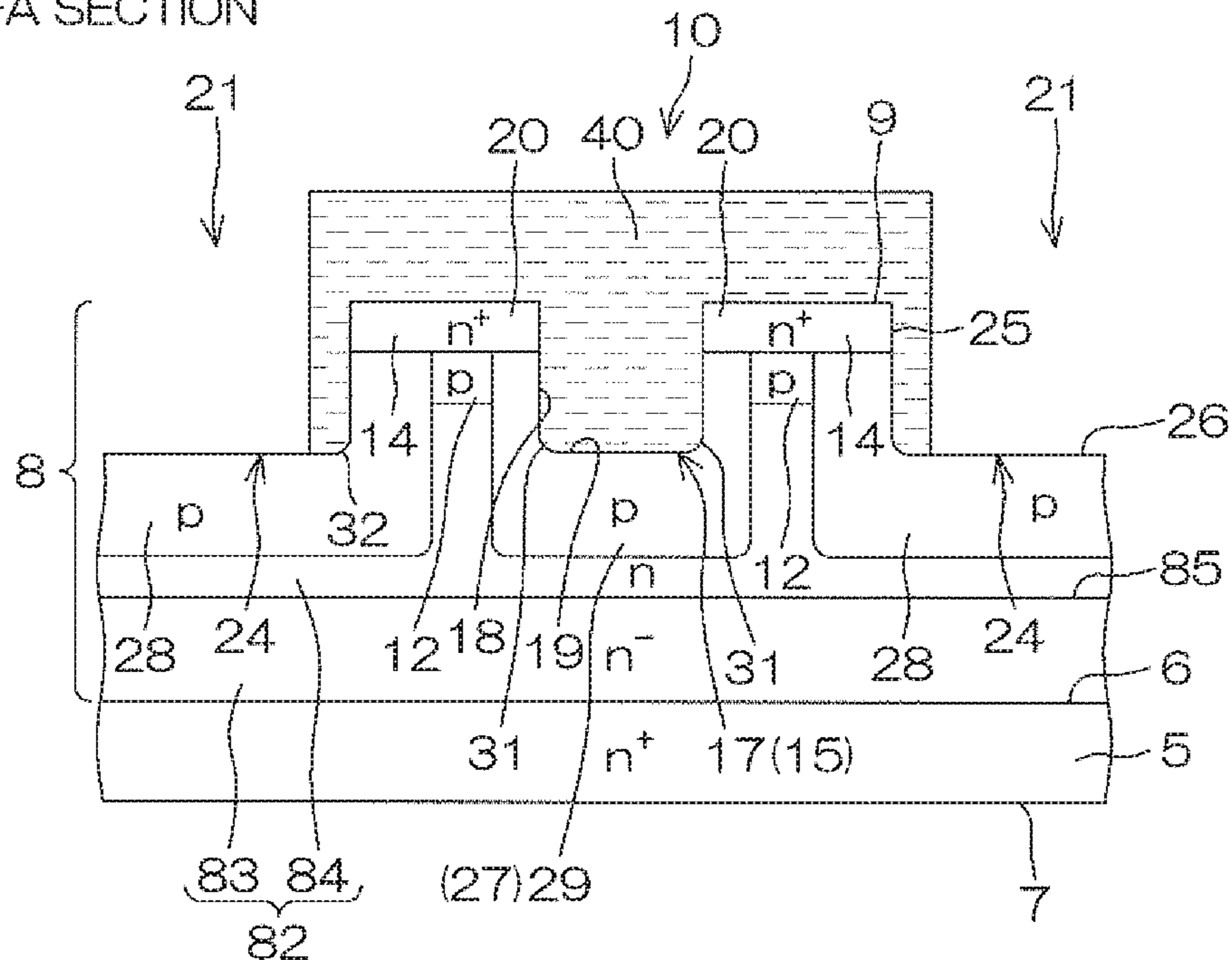
A-A SECTION
