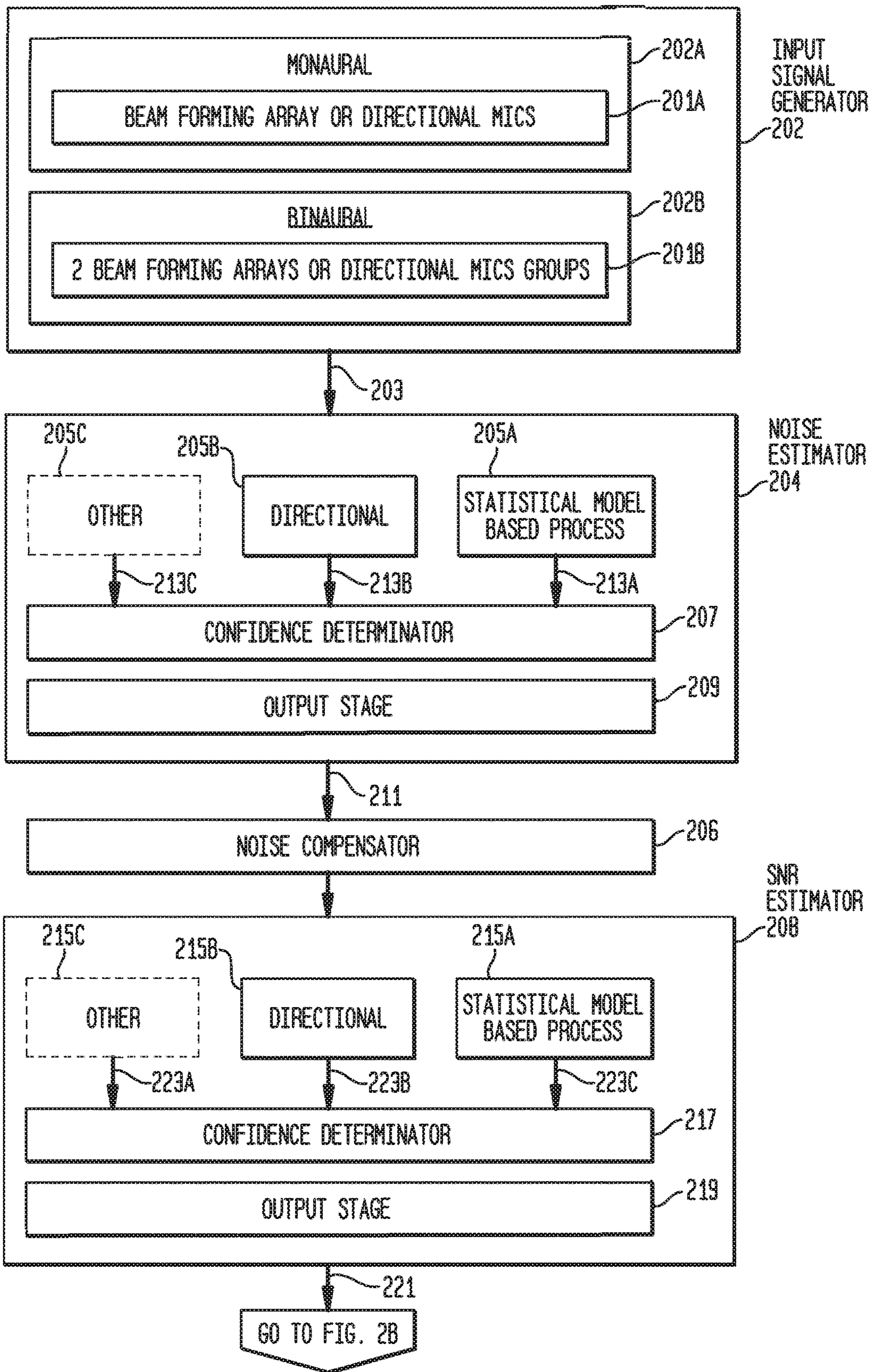
FIG. 2A
