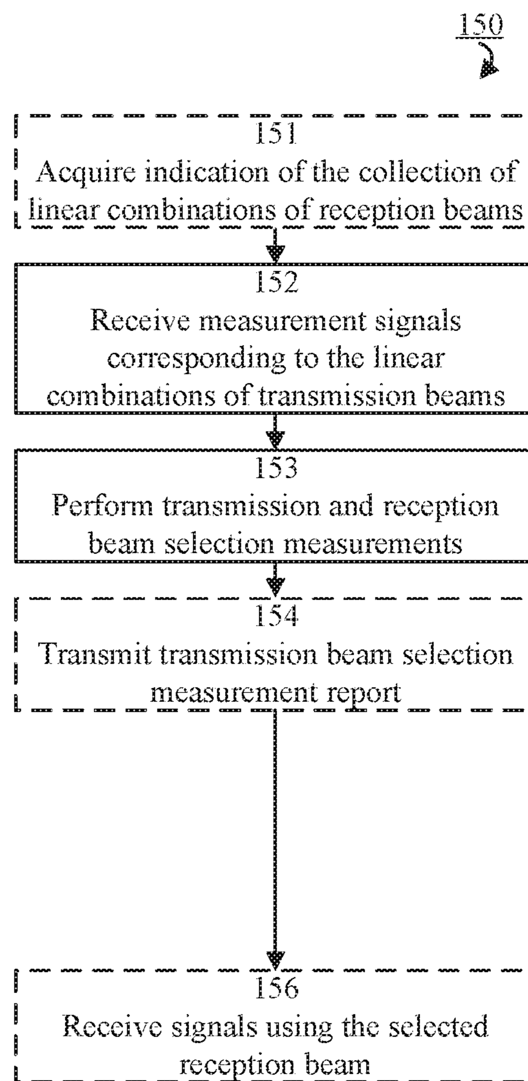
FIG. 1B
