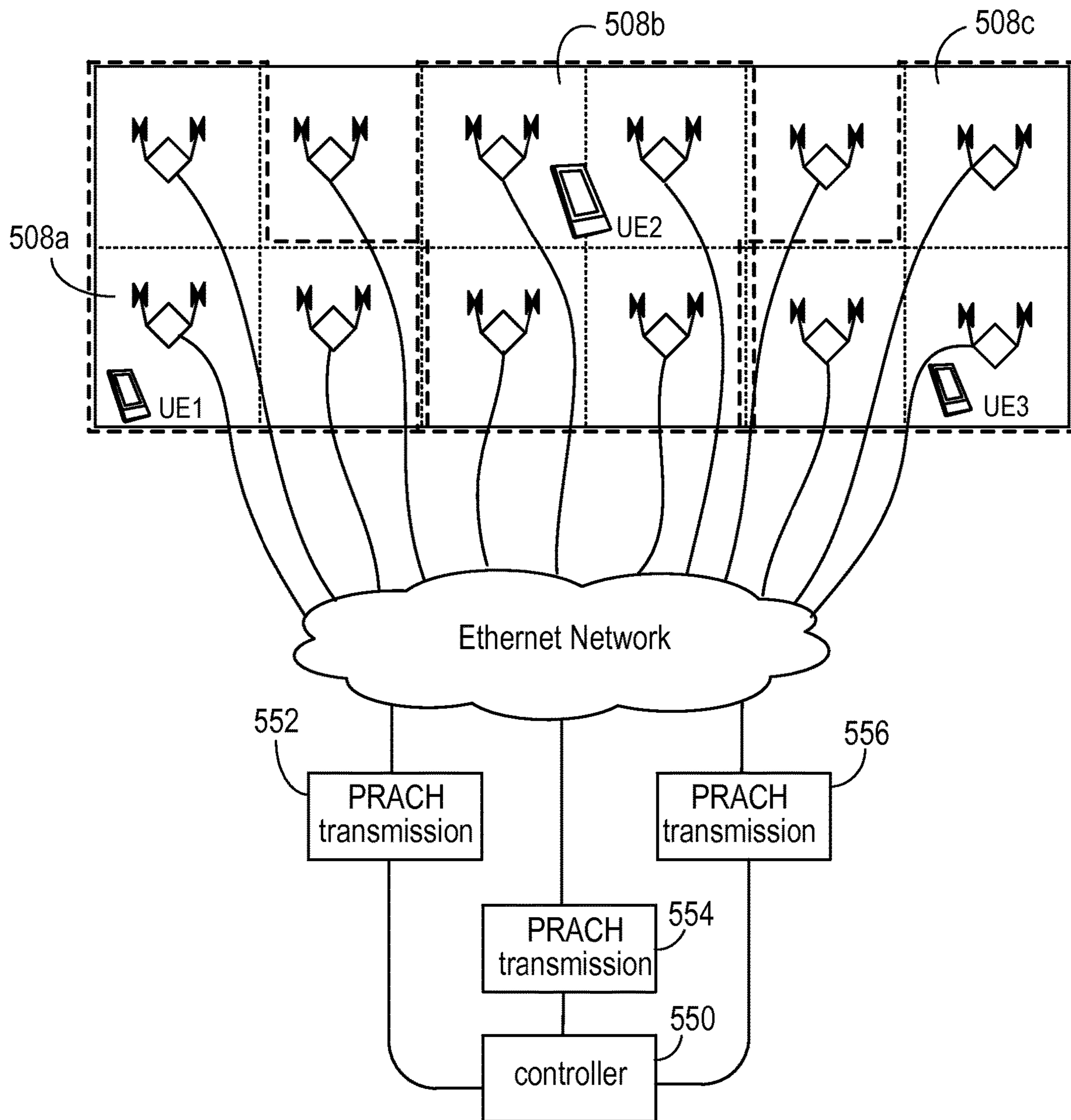
FIG. 5B
