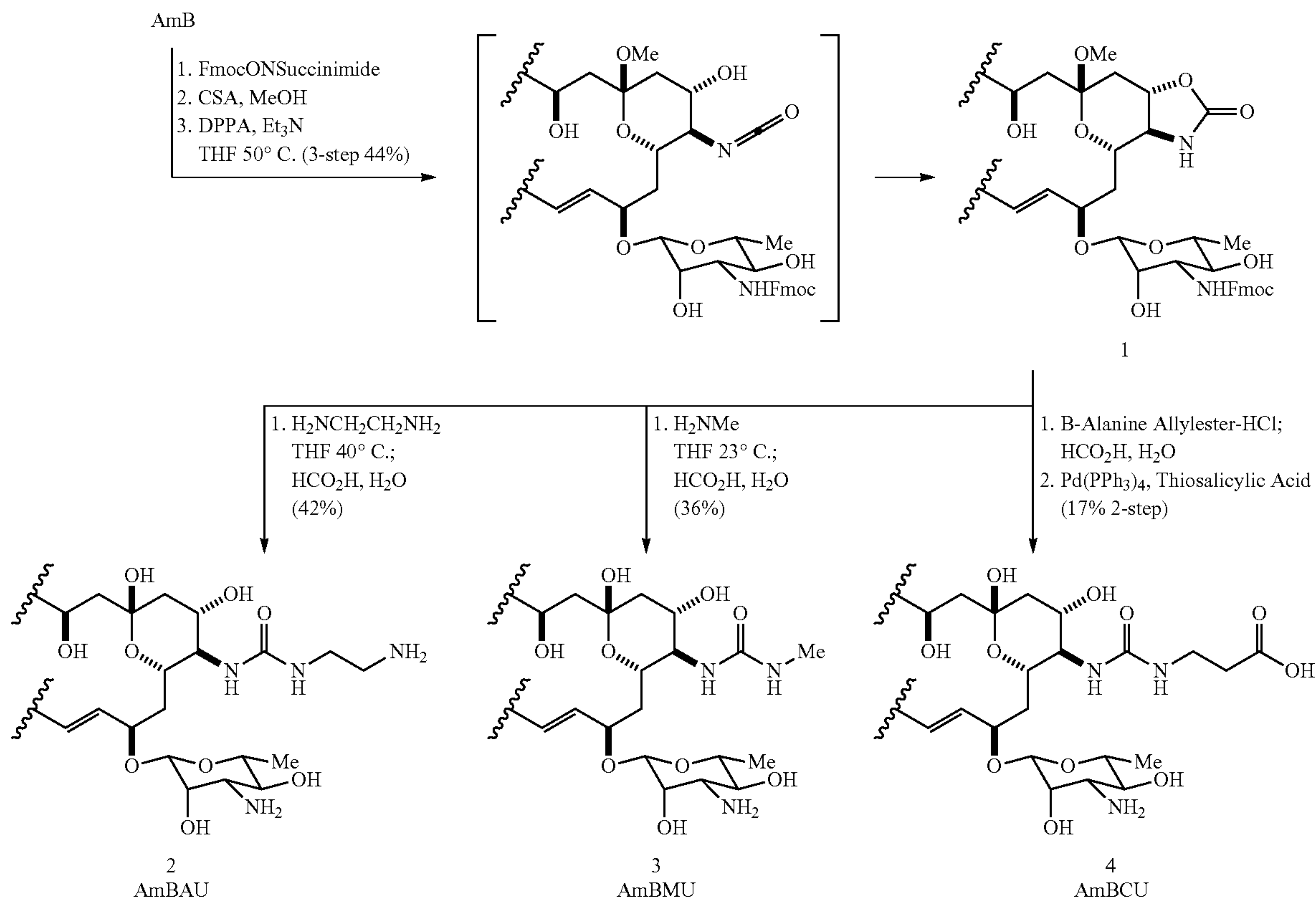
Scheme 1: Synthesis of C16 AmB derivatives
