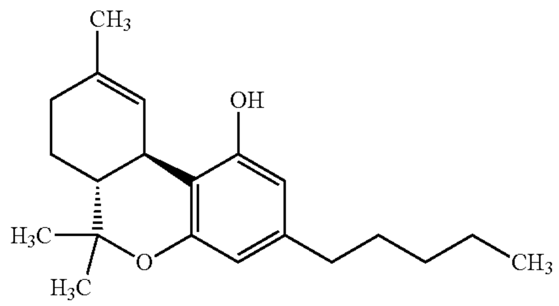
THC
