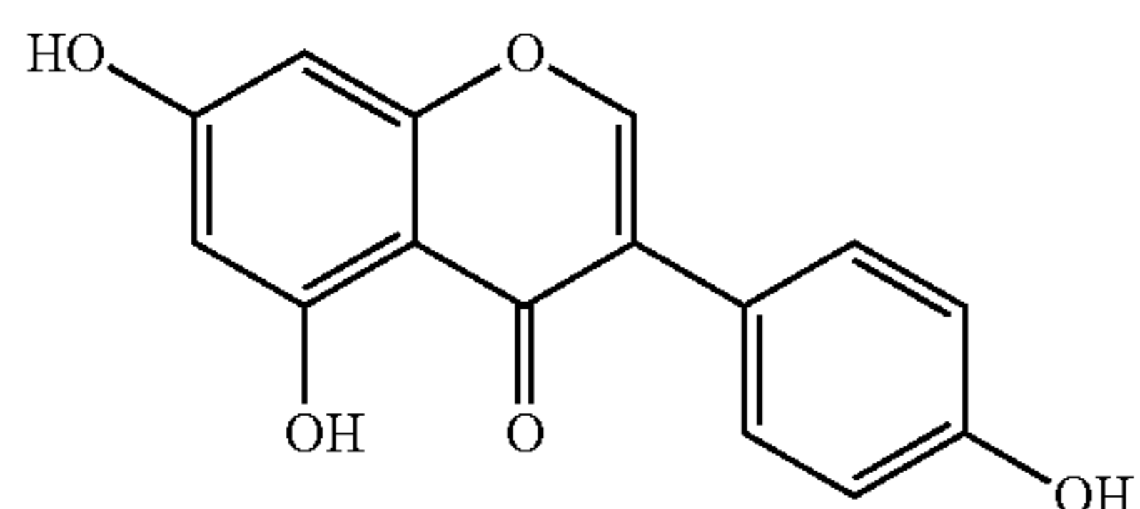
Genistein
