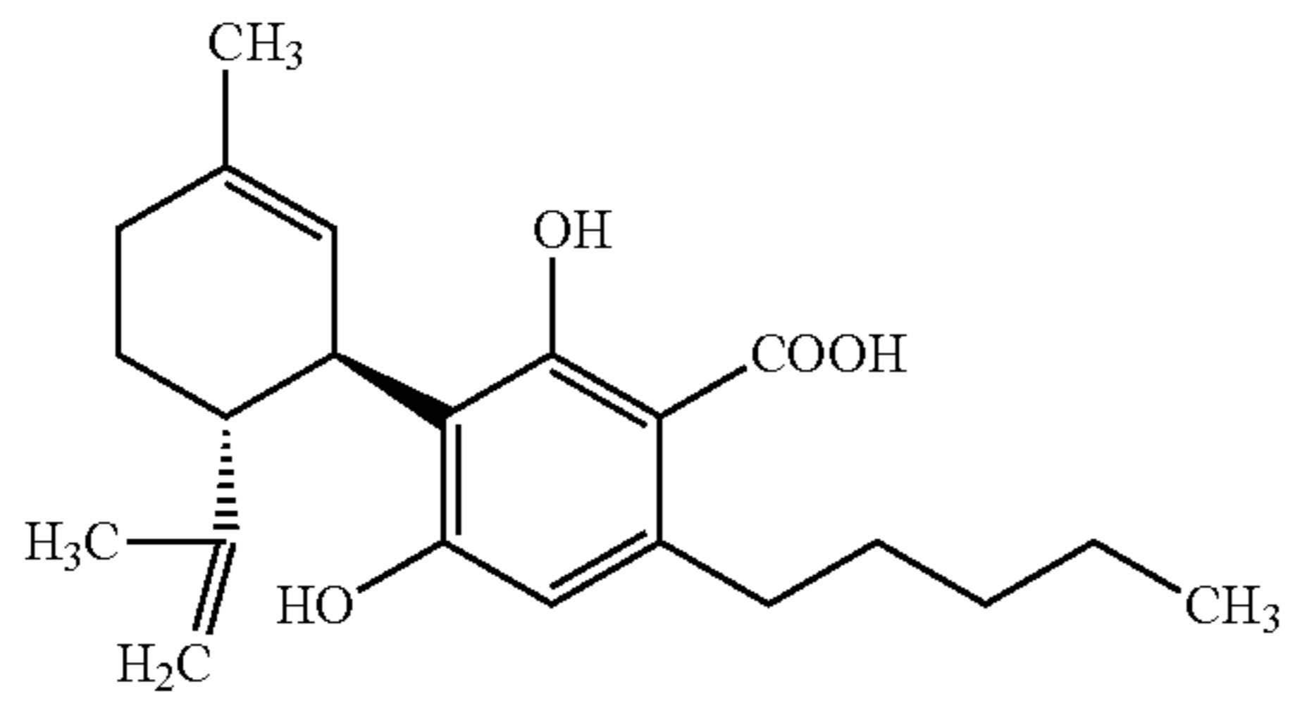
CBDA
