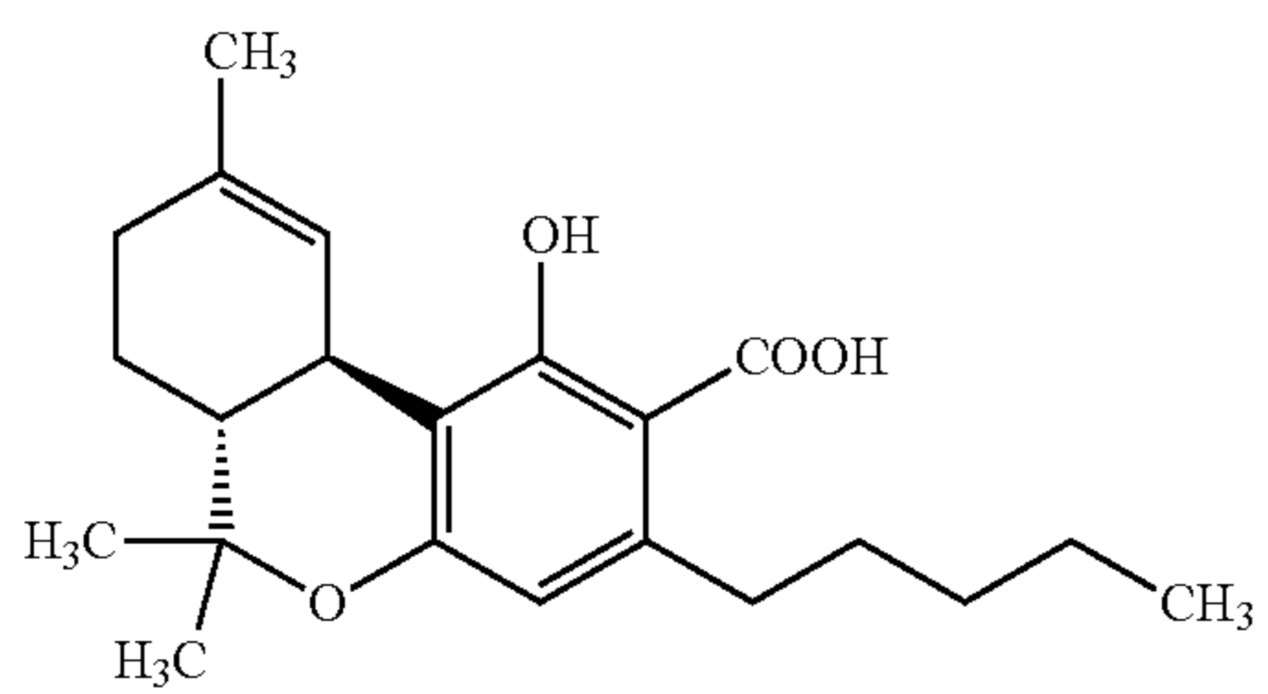
THCA
