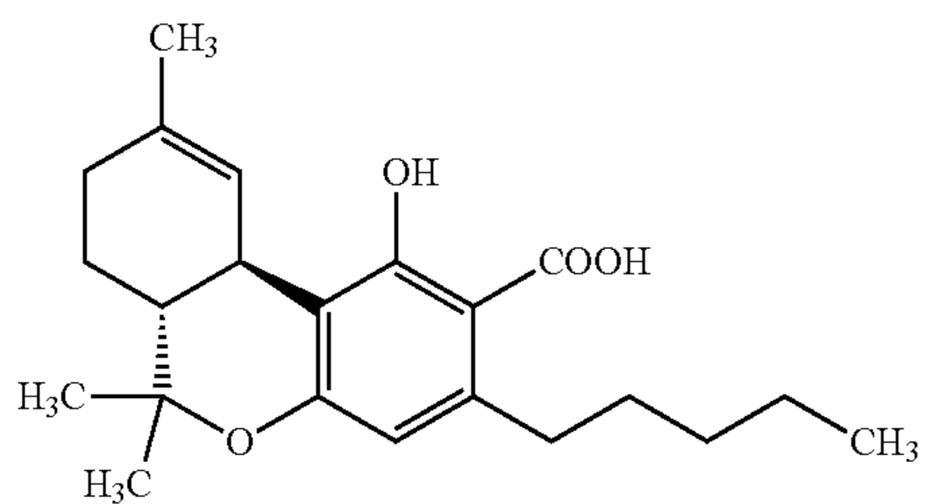
THCA
