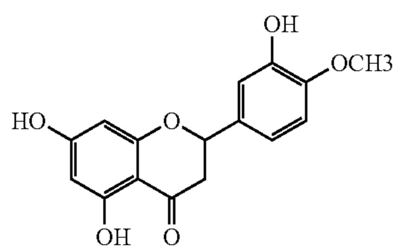
Hesperitin
