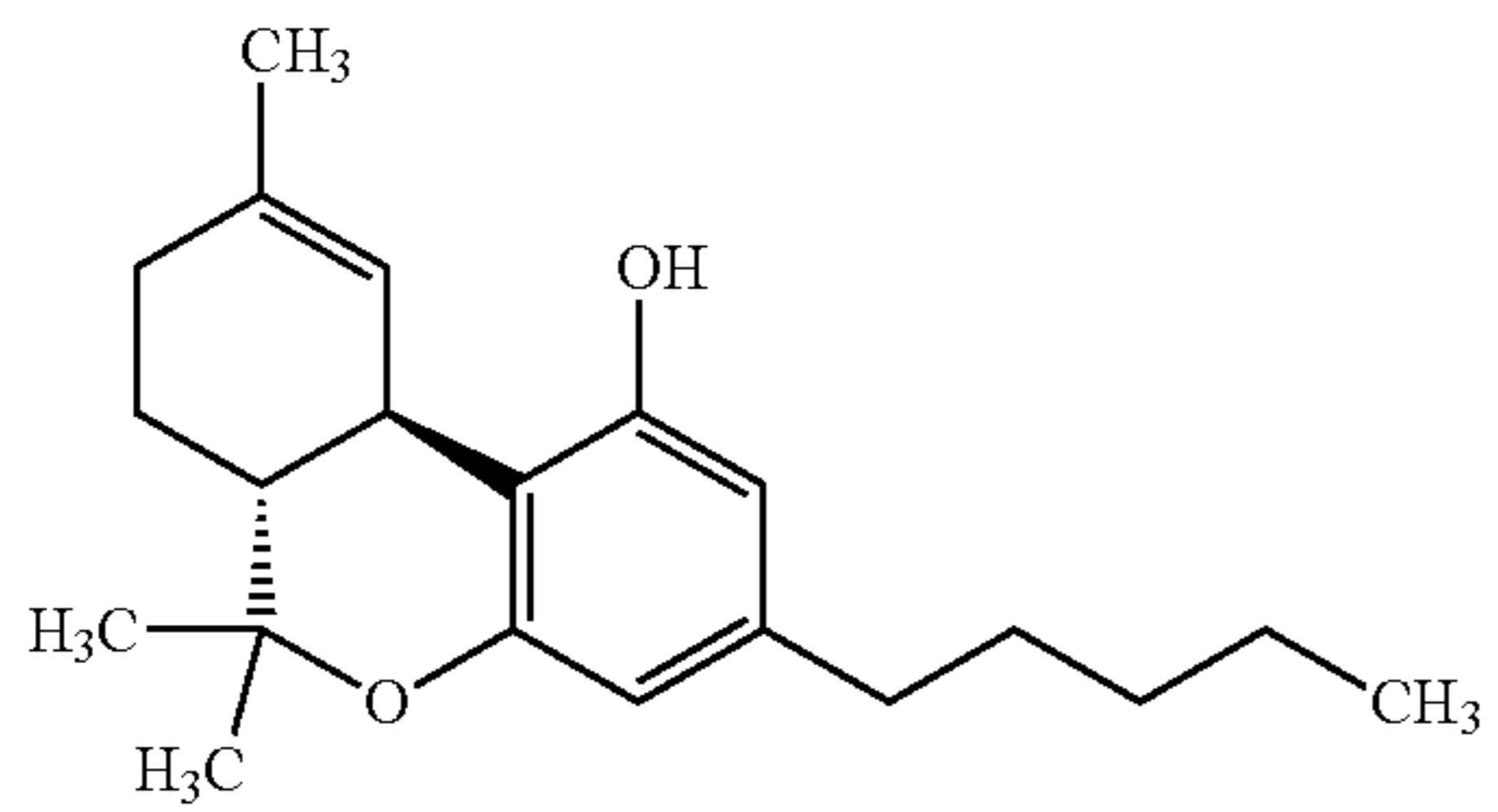
THC
