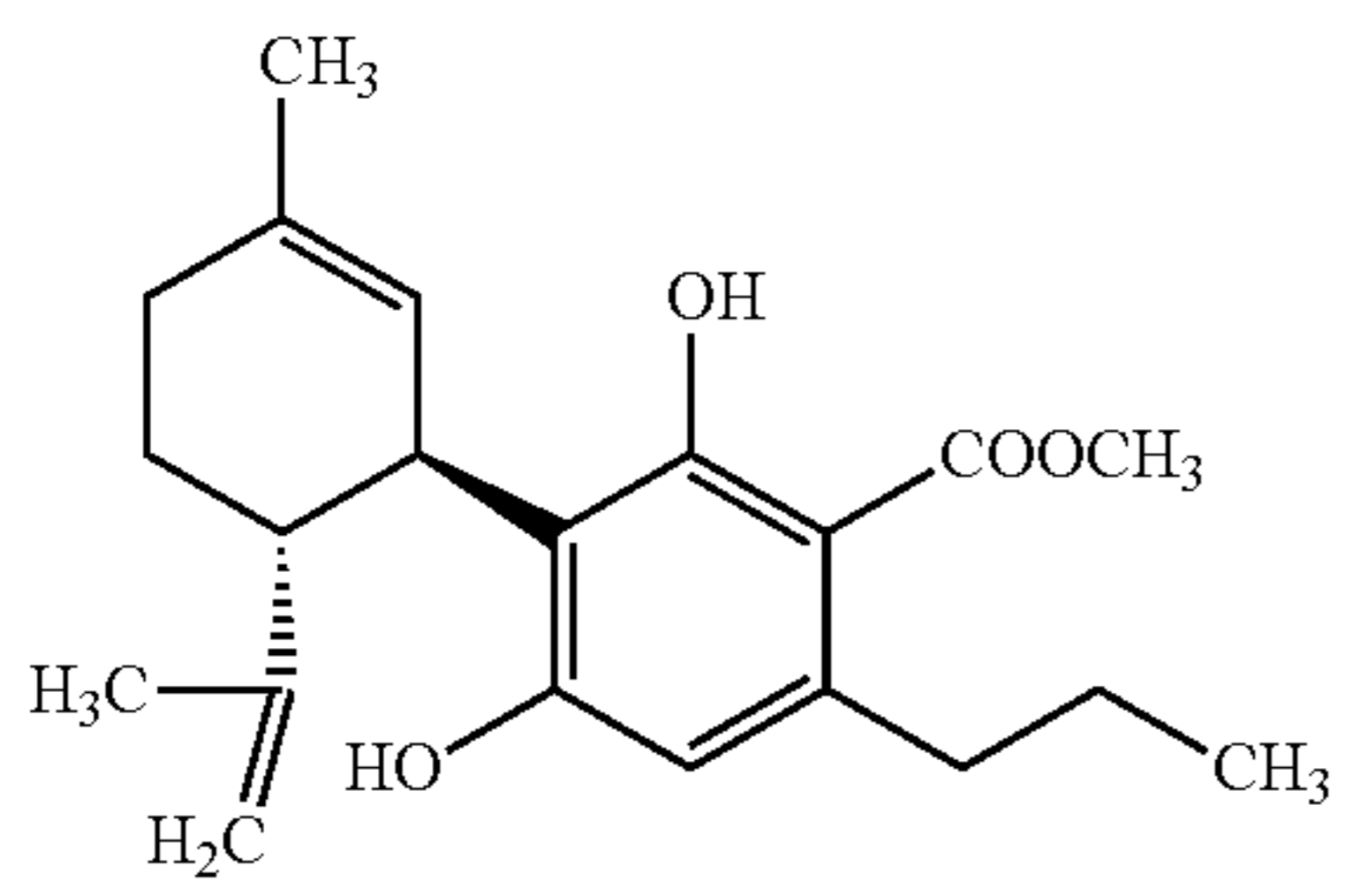
CBDVA-OMe
