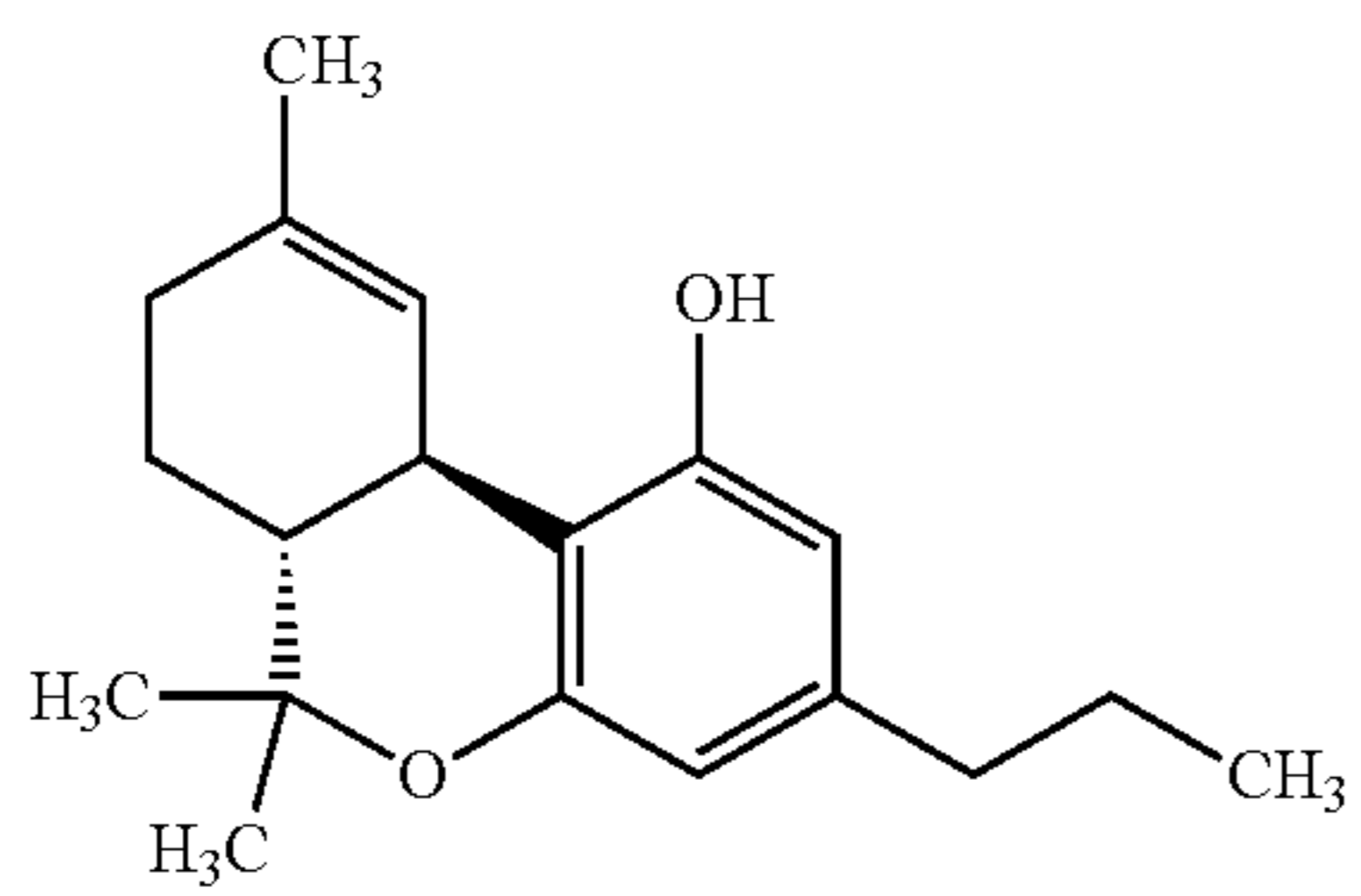
THCV
