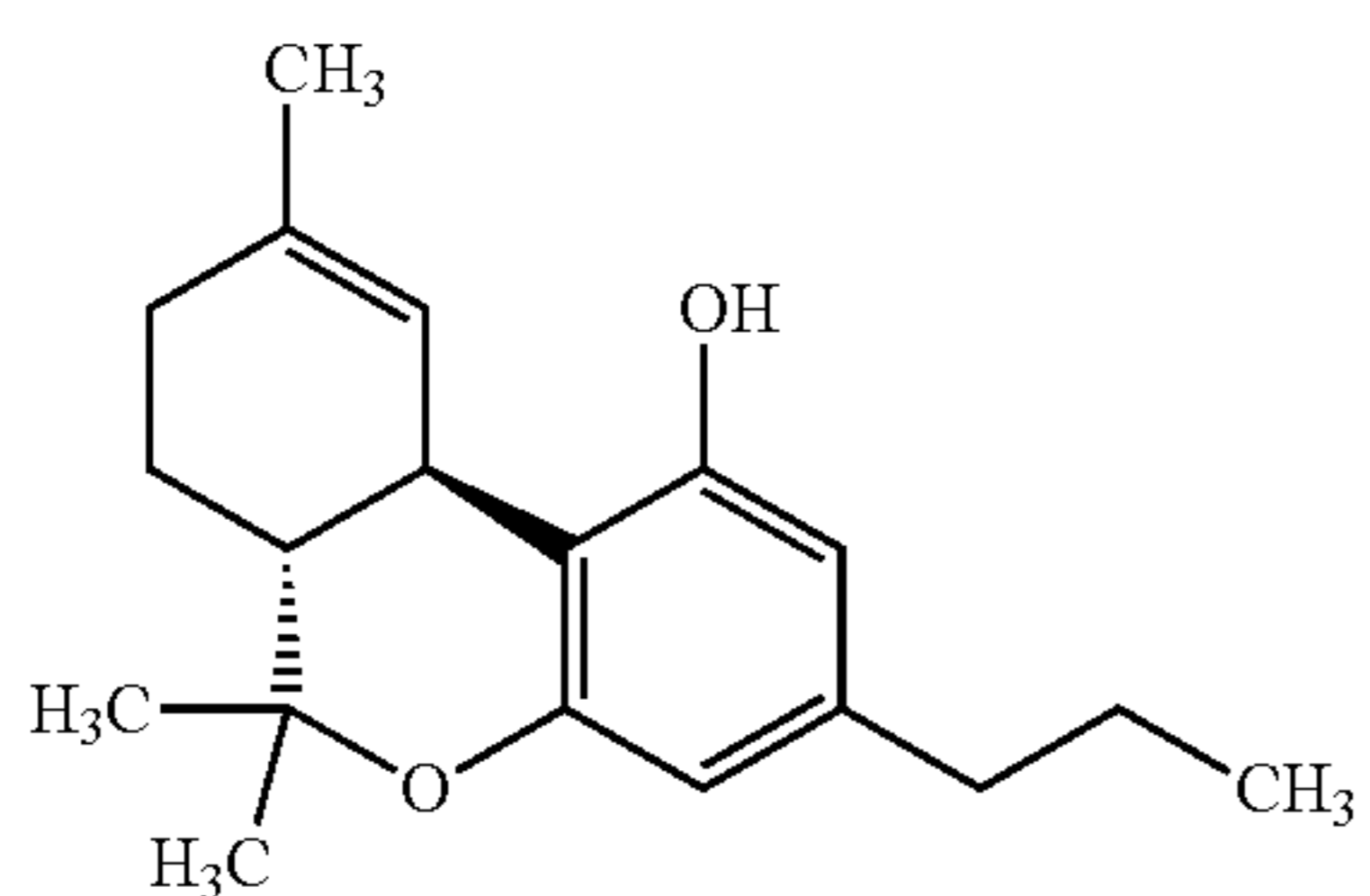
THCV
