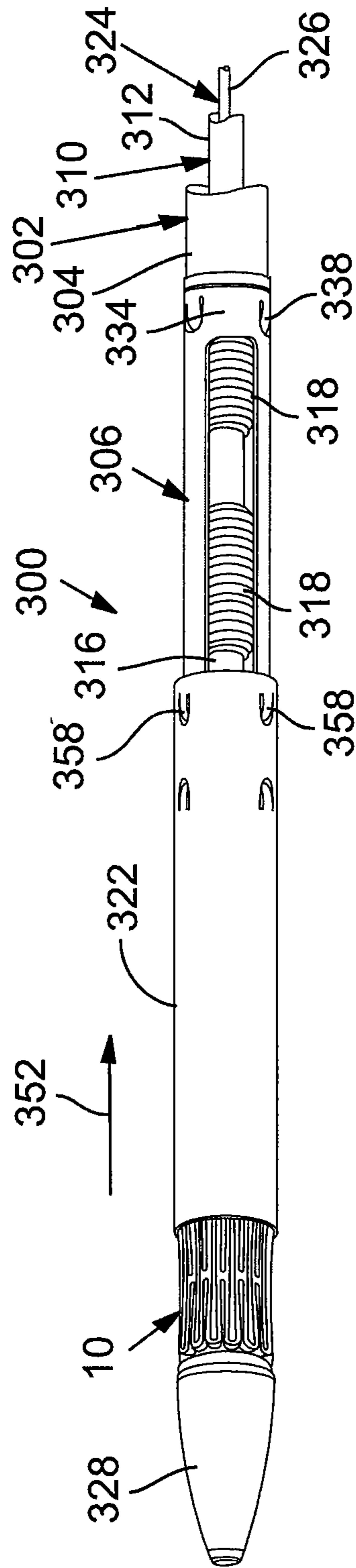
FIG. 31
