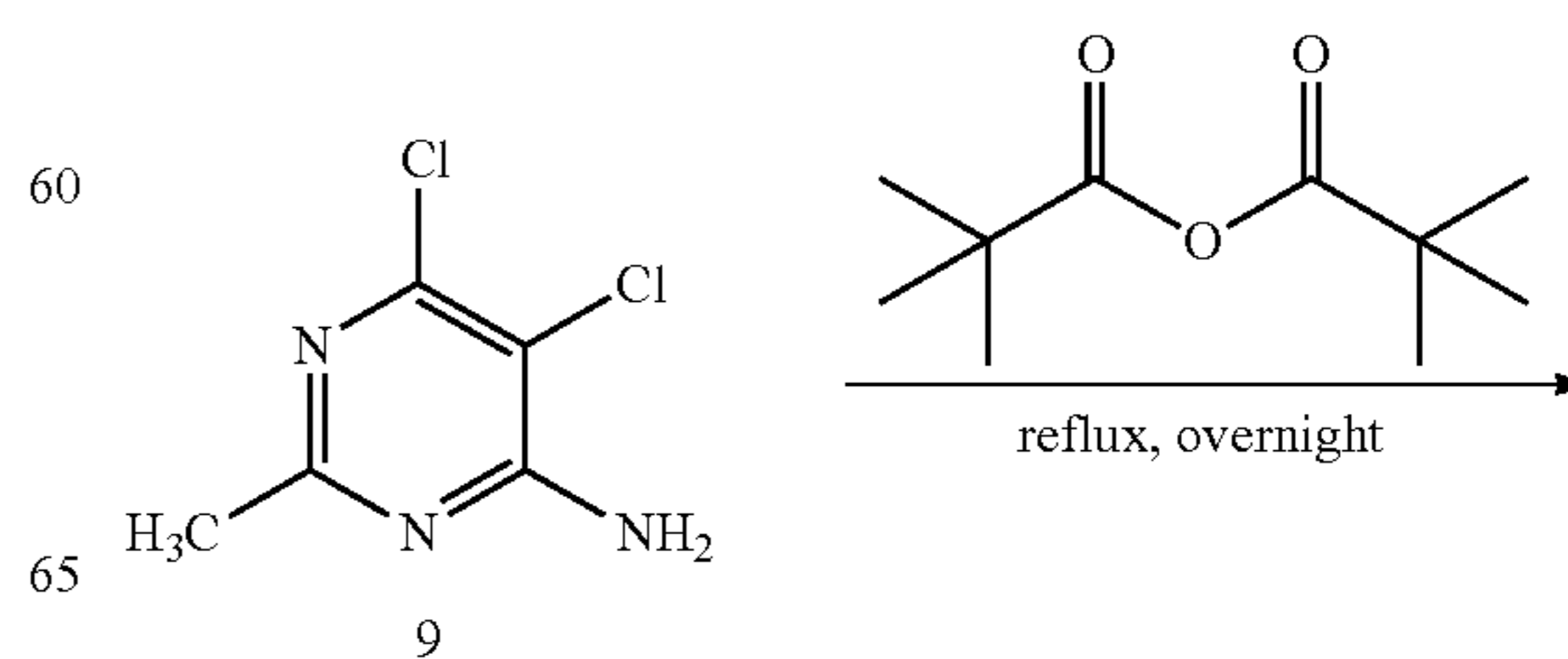
Scheme 1A
