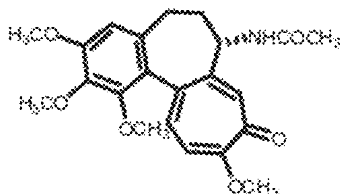
colchicine
