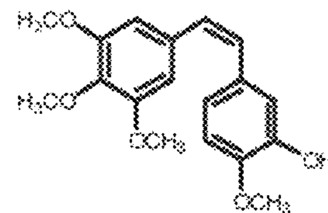
combretastatin A-4
