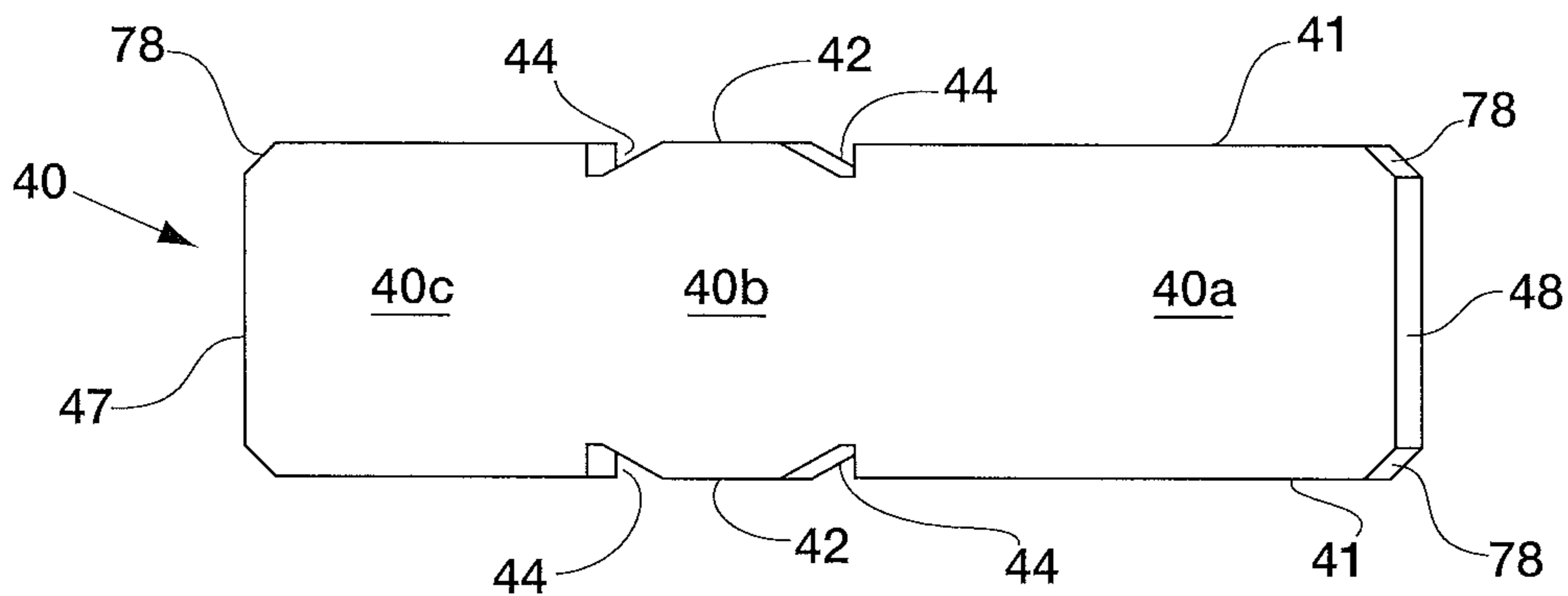
FIG. 2C
