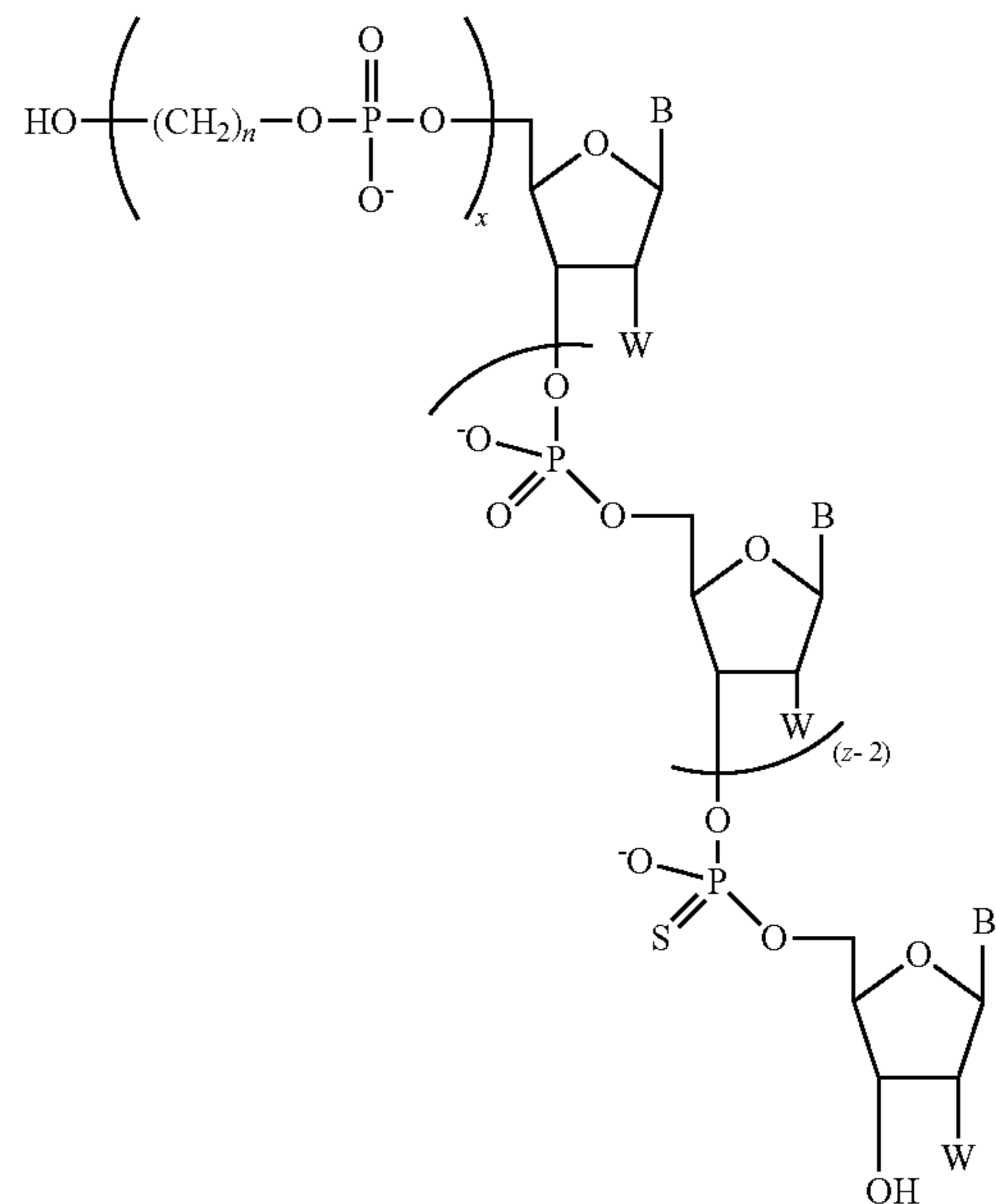
Formula I-A
