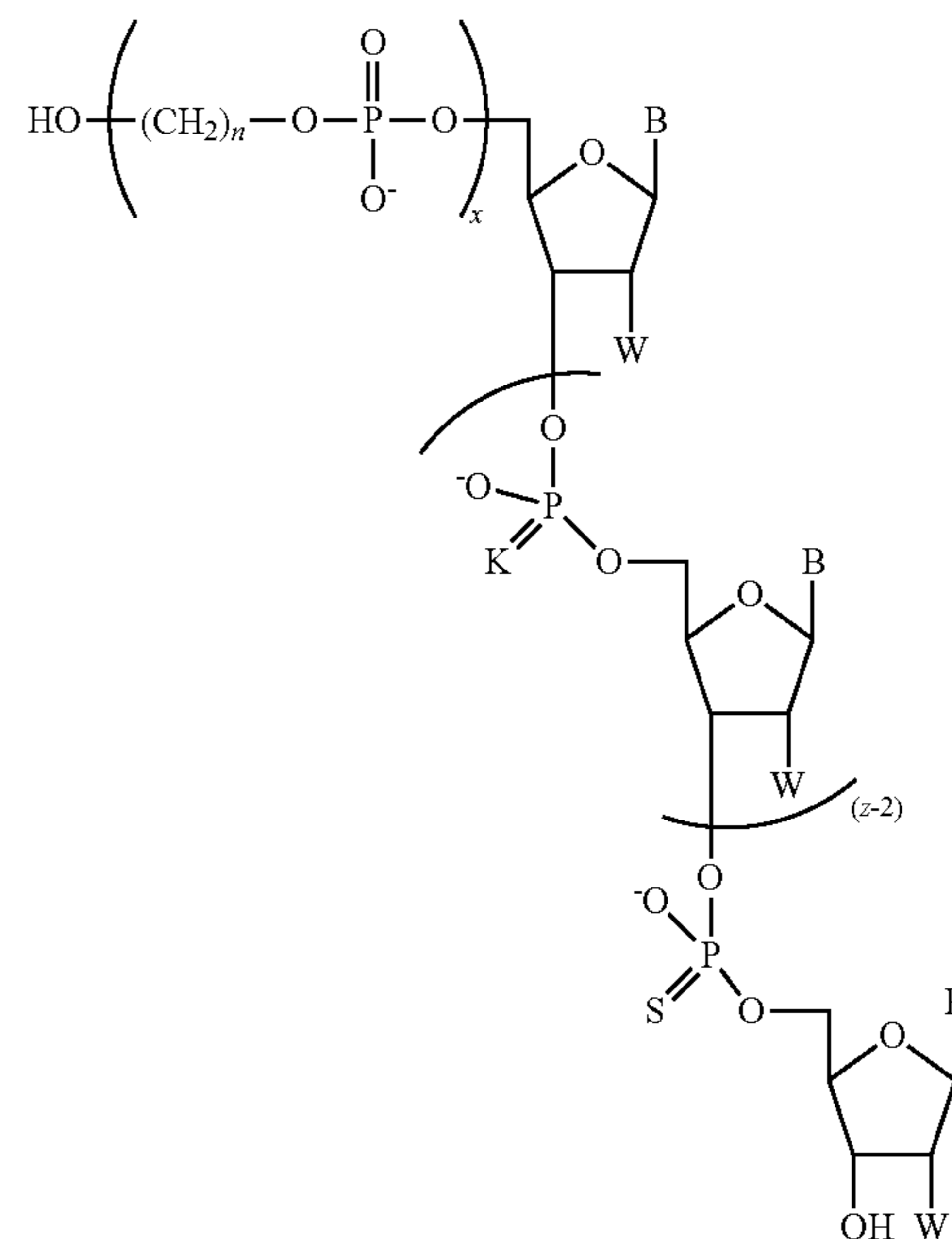
Formula I-A
