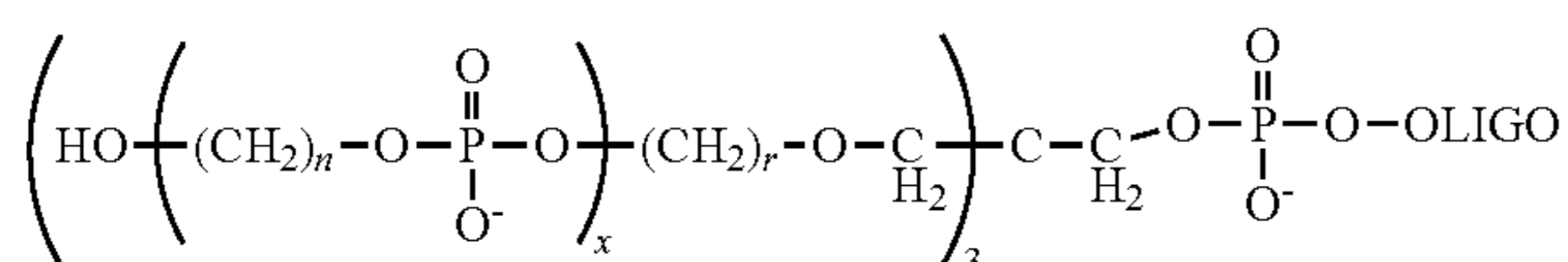
Formula VI-A
