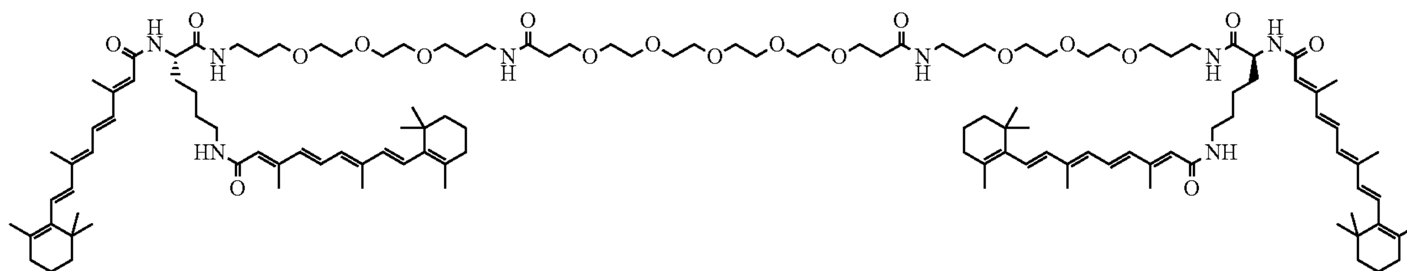
DiVA-PEG-DiVA
