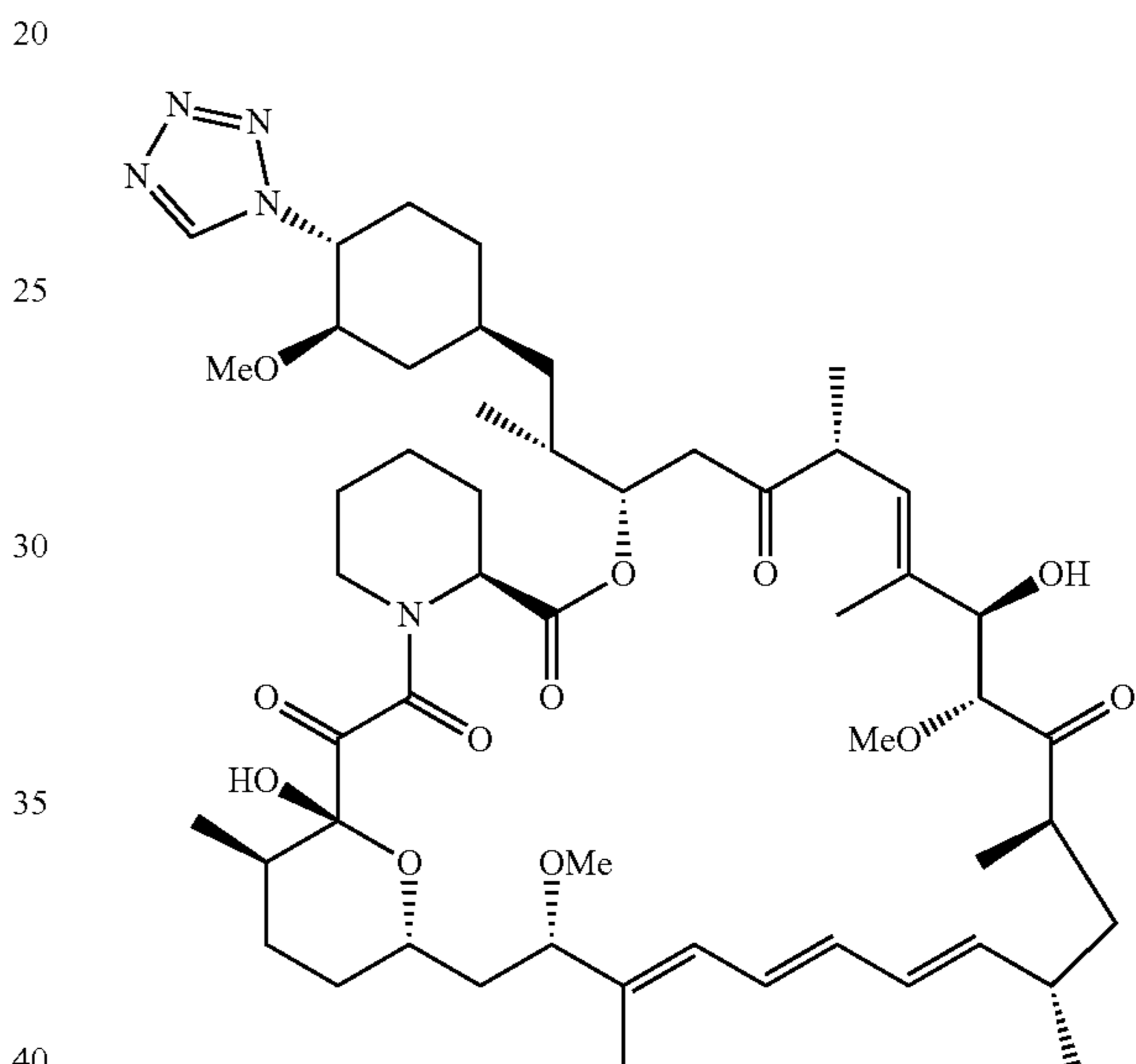
Zotarolimus (ABT-578)
