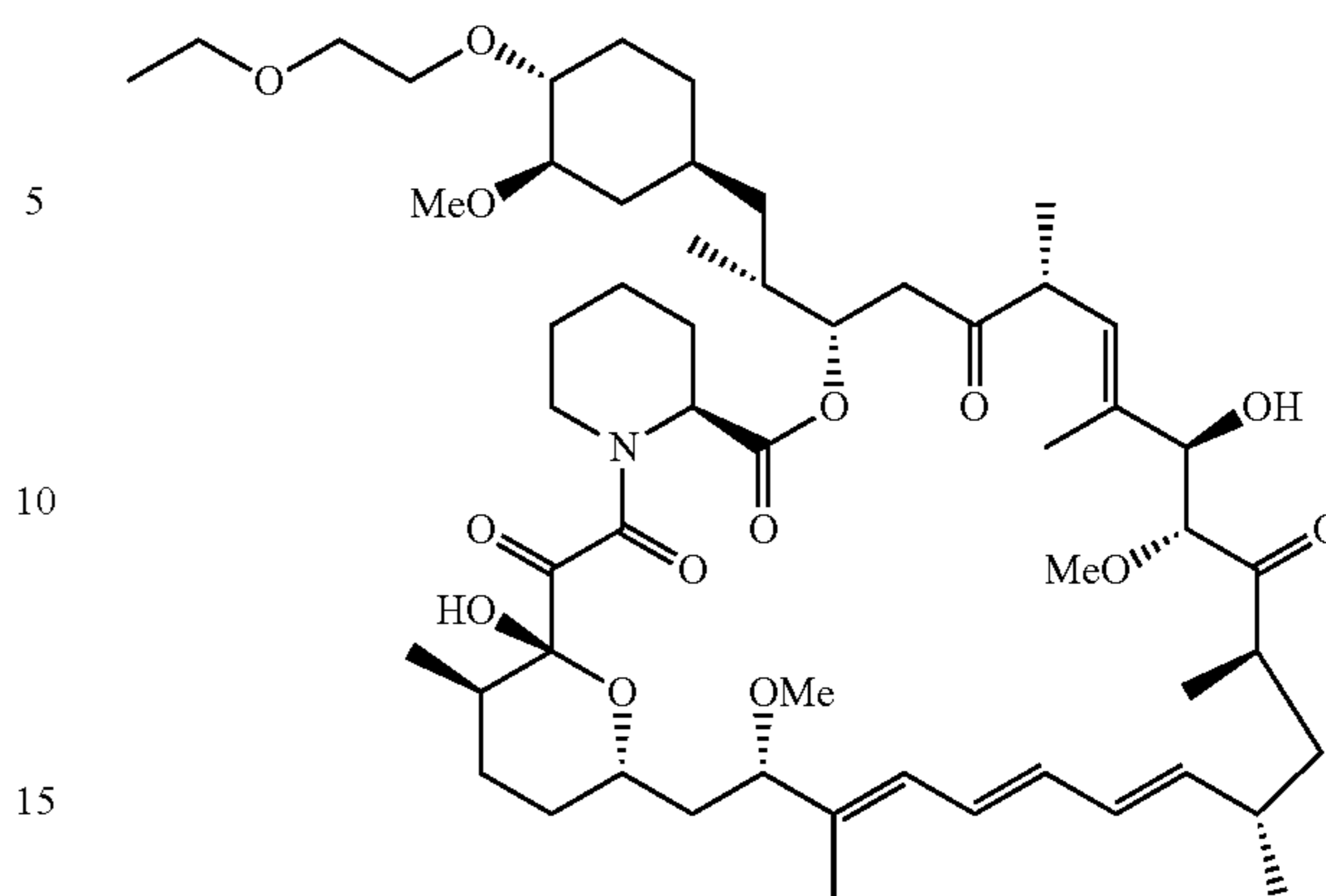
Umirolimus
