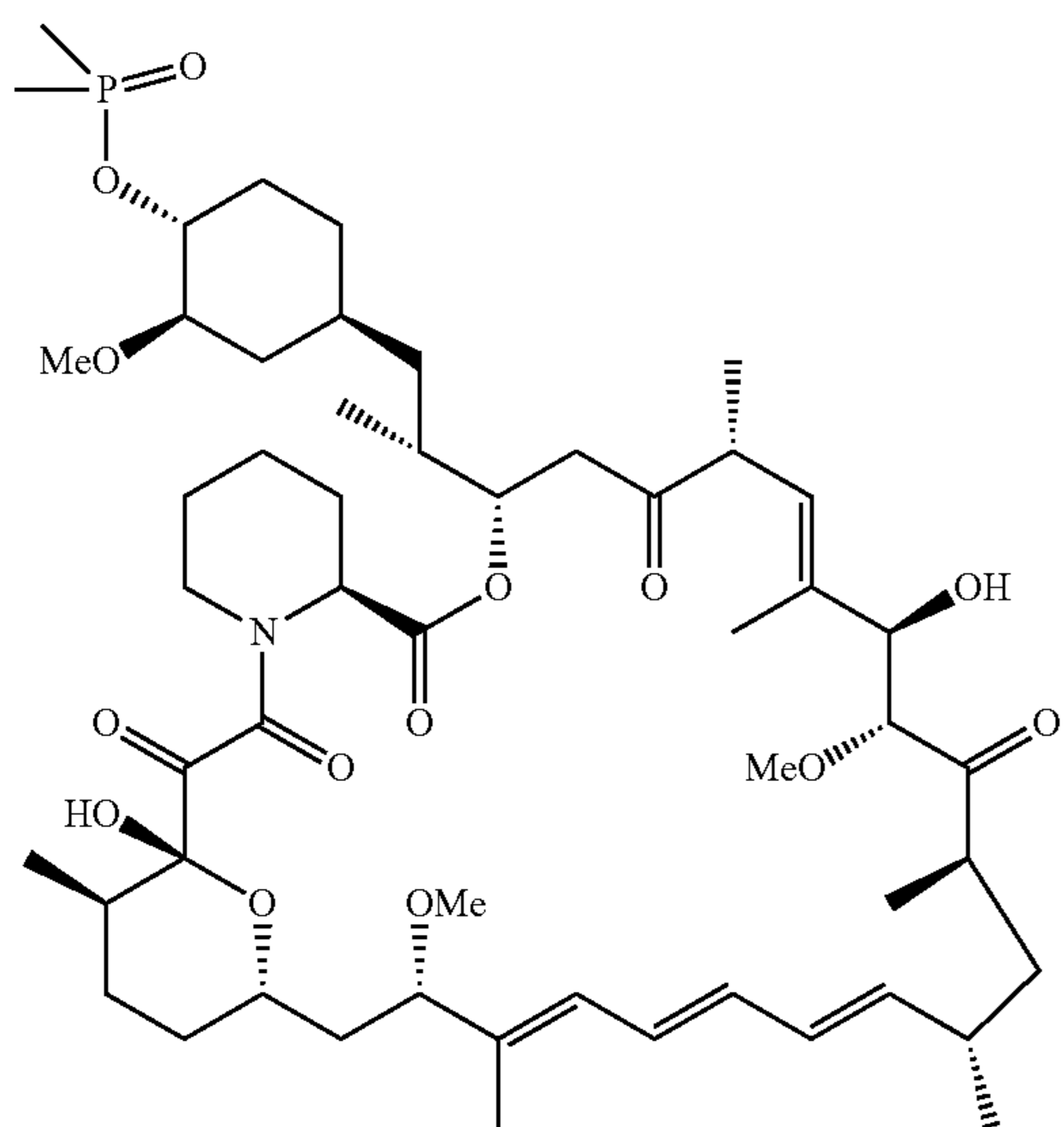
Ridaforolimus (MK-8669)
