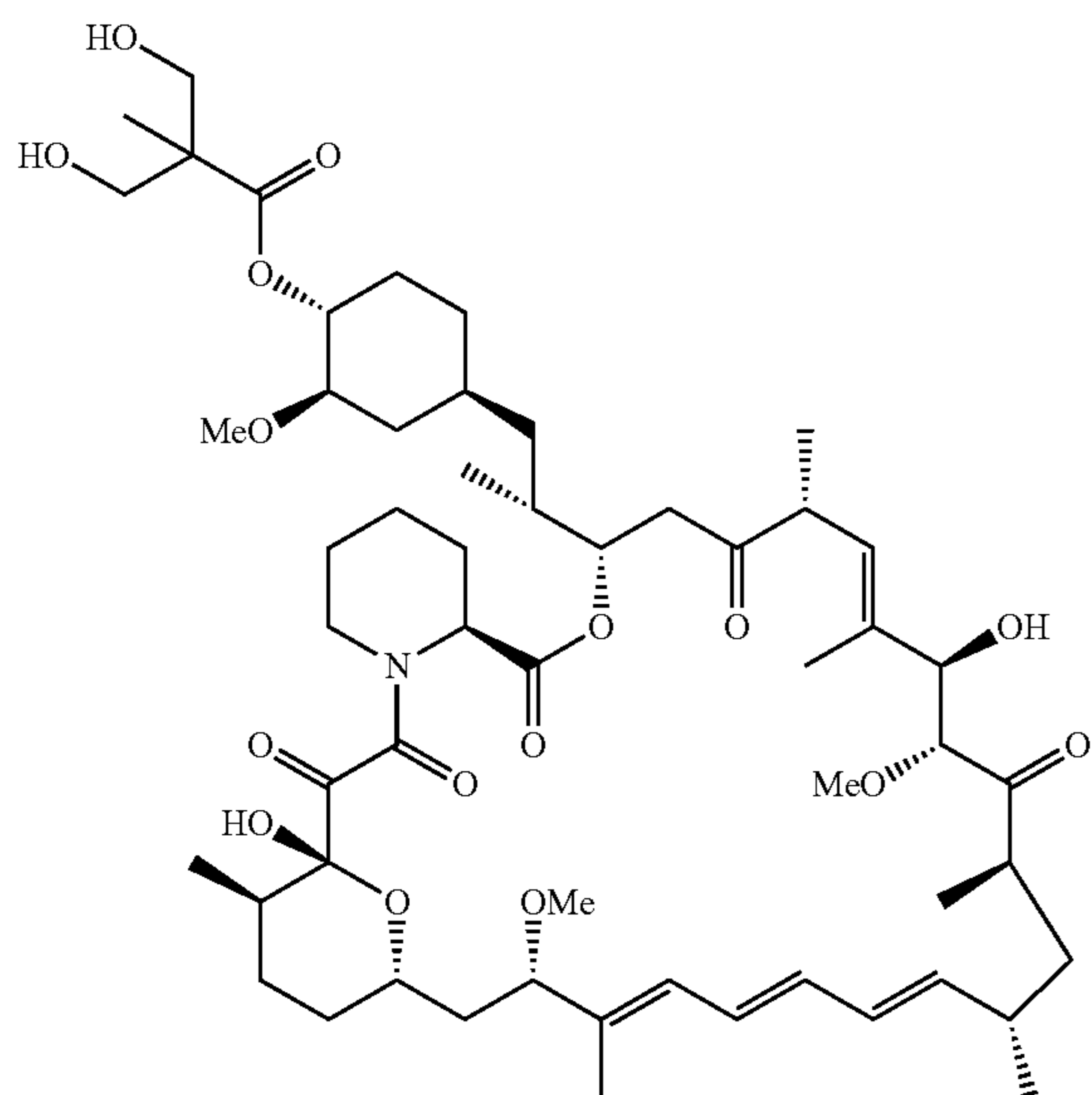
Temsirolimus (CCI-779)
