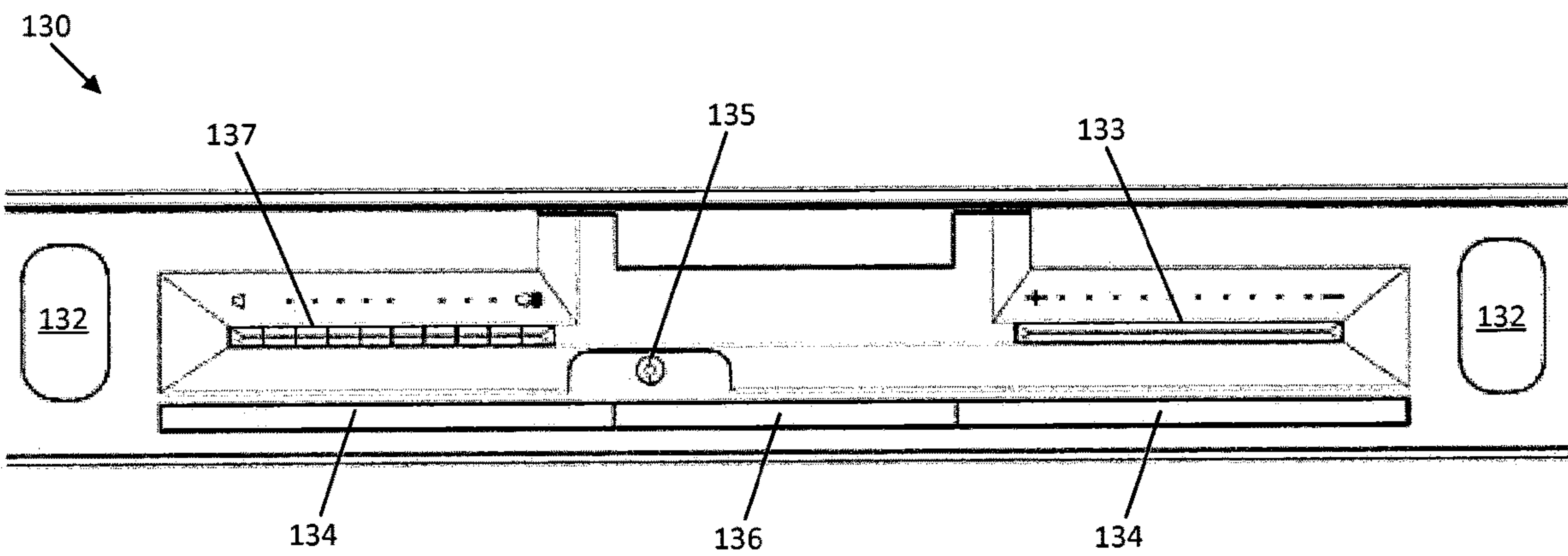
FIG. 15
