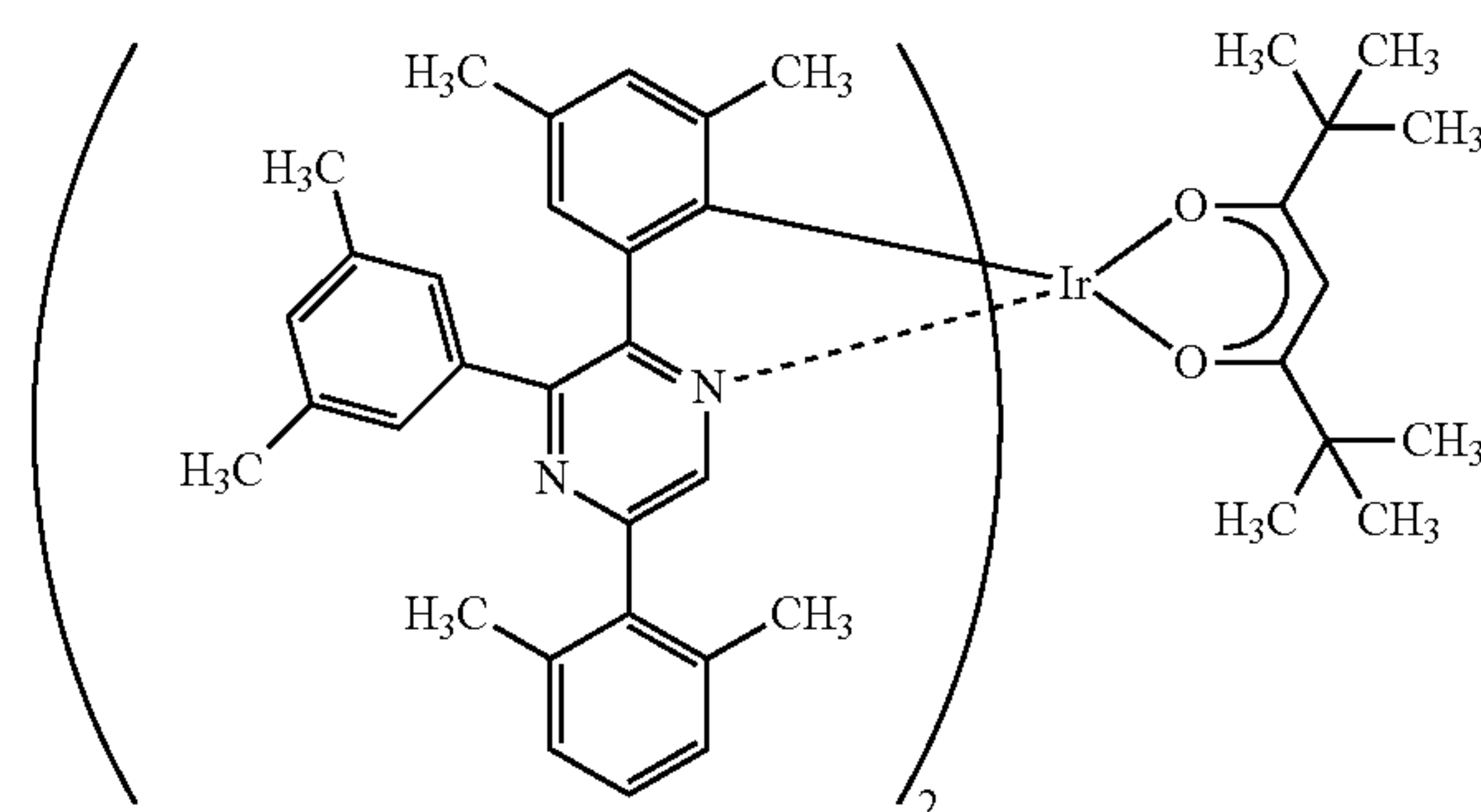
Ir(dmdppr-dmp) 2 (dpm)
