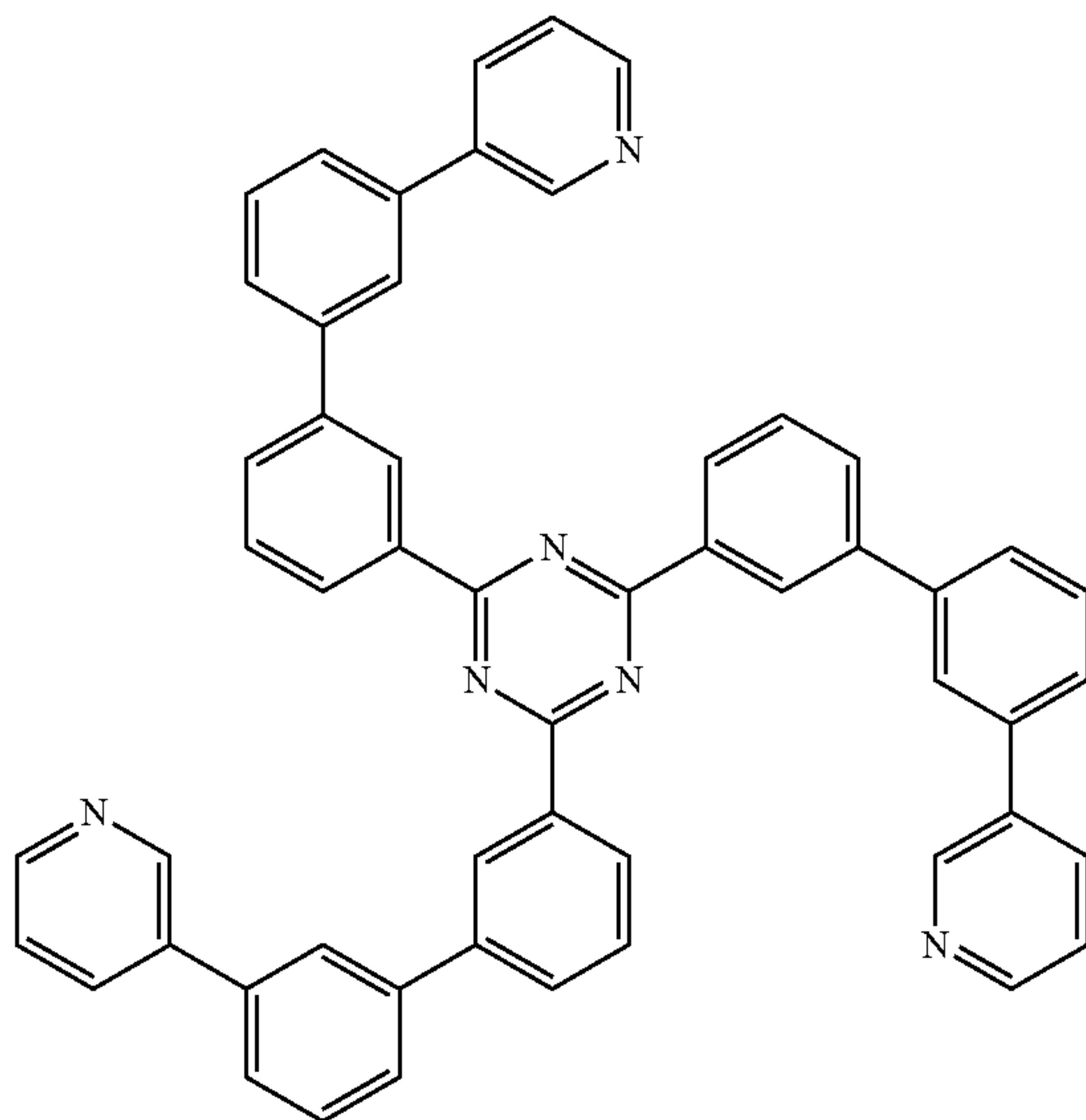
TmPPPyTz
