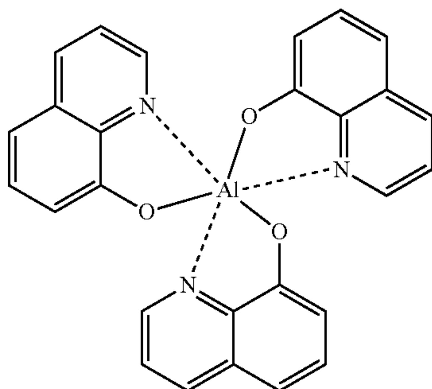
Alq3
