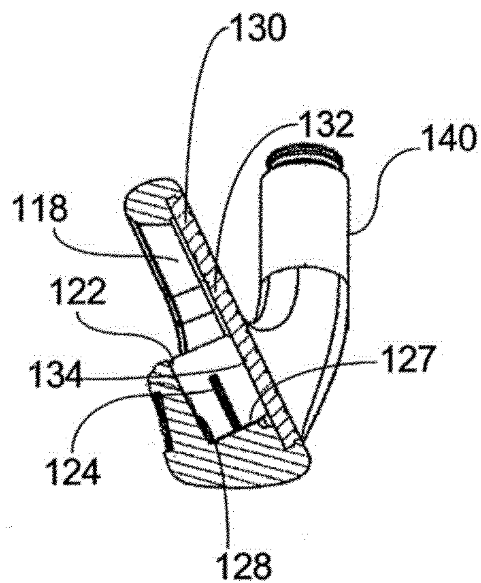
FIG. 3
