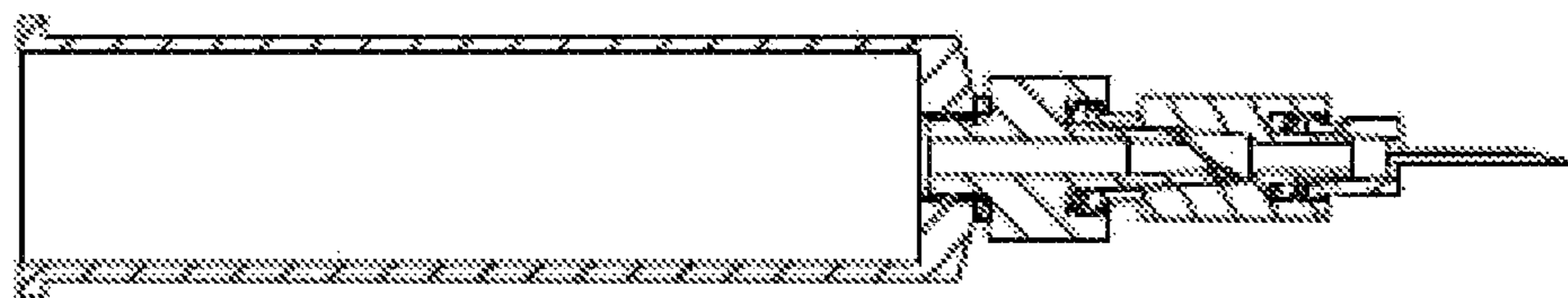
SECTION A-A
