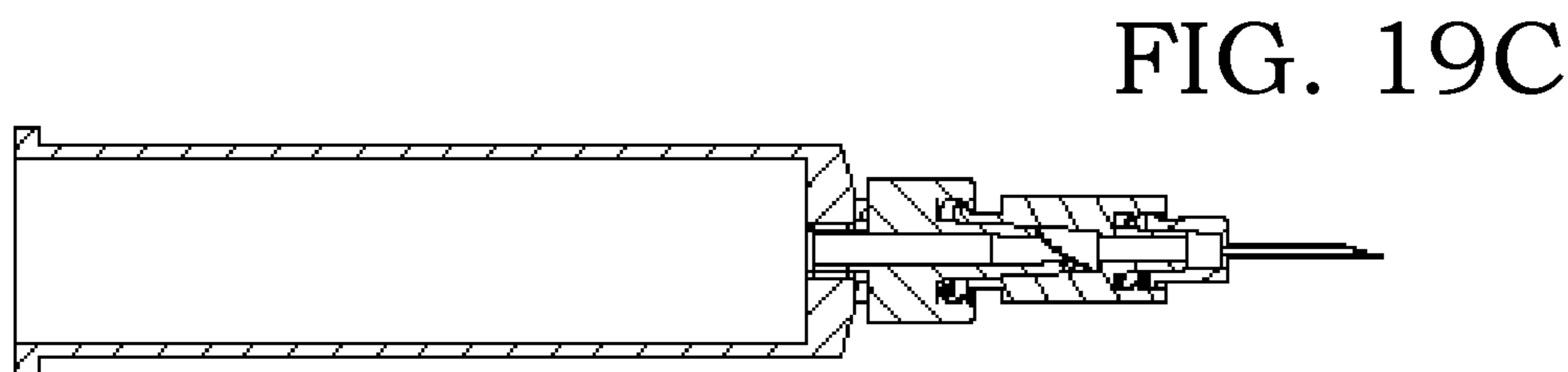
SECTION A-A
