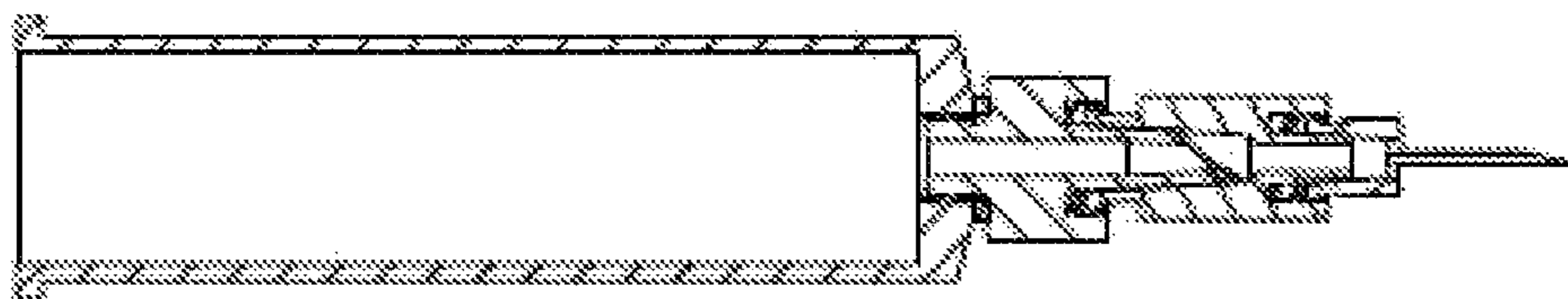
SECTION A-A
