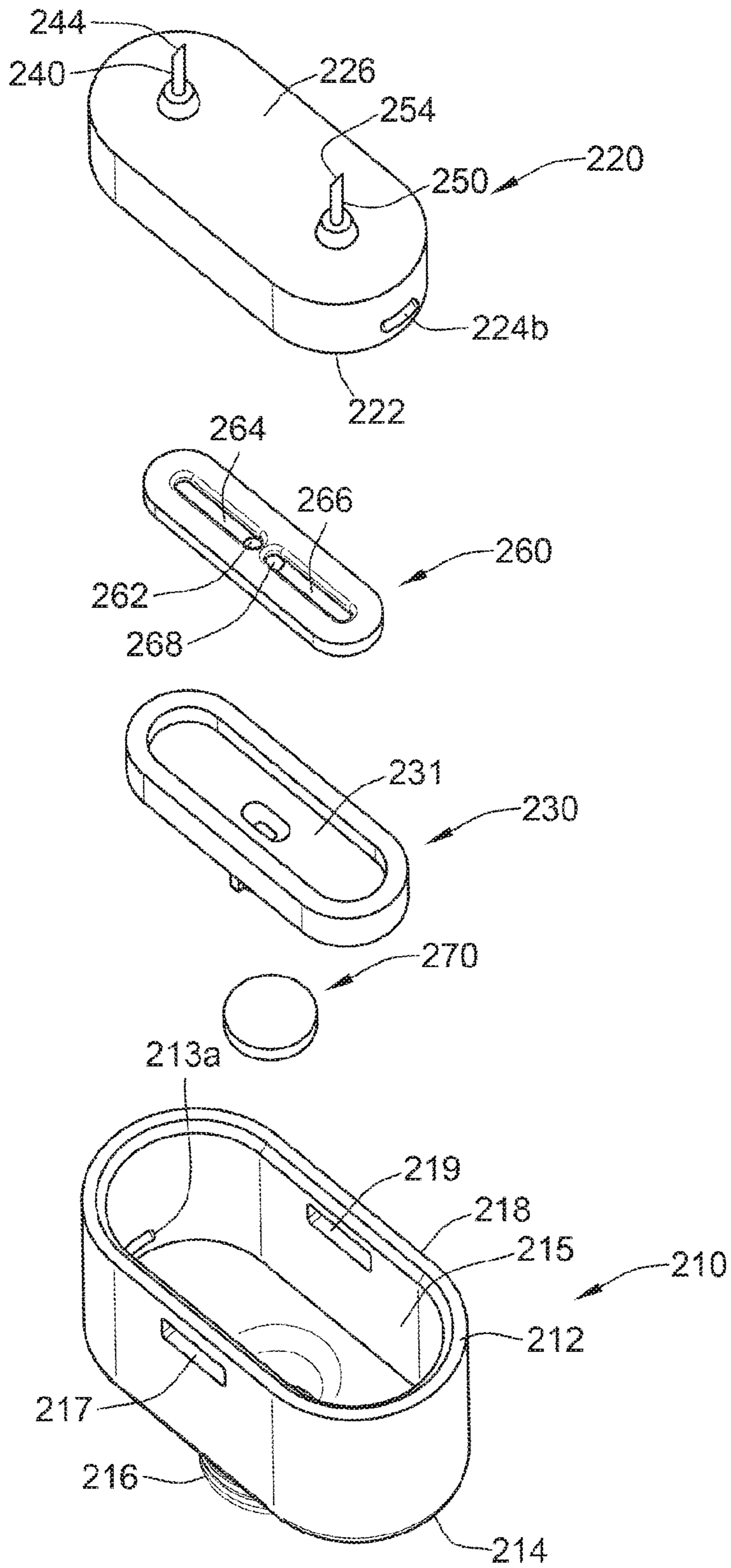
FIG. 17
